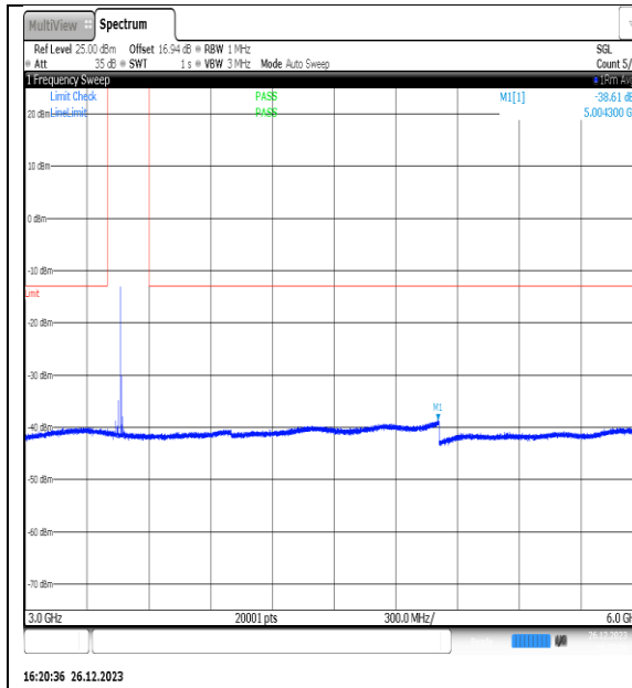
NTNV_N77-3450- 3550_PC2_30_15_L_TID15_NS_01_3000_6000_ #1
