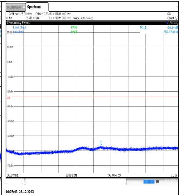
NTNV_N77-3450-3550_PC2_30_15_L_TID12_NS_01_30_1000_#1
