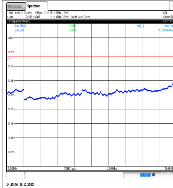
NTNV_N77-3450- 3550_PC2_30_10_H_TID9_NS_01_6000_26000_# 1
