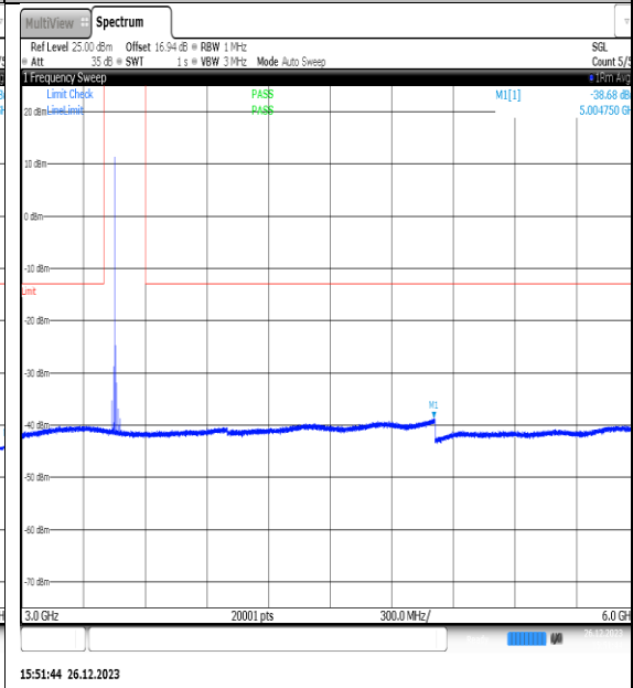
NTNV_N77-3450- 3550_PC2_30_15_L_TID8_NS_01_3000_6000_#1
