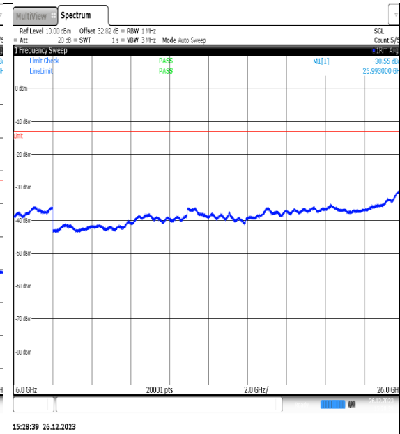
NTNV_N77-3450- 3550_PC2_30_15_L_TID3_NS_01_6000_26000_# #1
