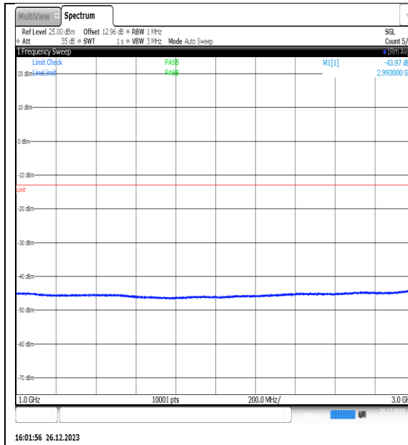
NTNV_N77-3450- 3550_PC2_30_15_L_TID10_NS_01_1000_3000_ #1
