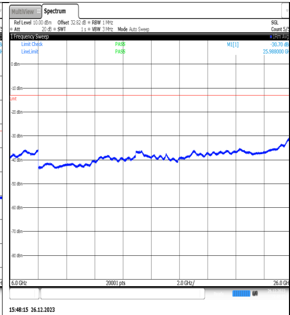
NTNV_N77-3450- 3550_PC2_30_15_L_TID7_NS_01_6000_26000_# 1
