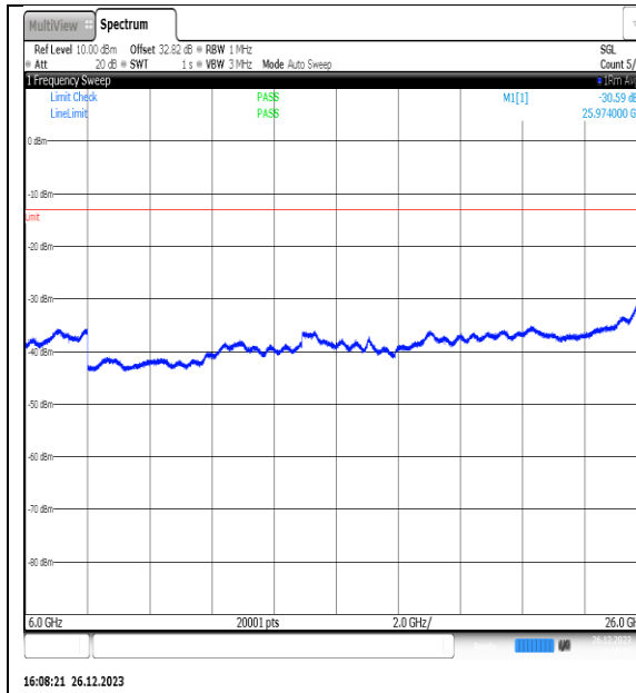
NTNV_N77-3450- 3550_PC2_30_15_L_TID12_NS_01_6000_26000 _#1
