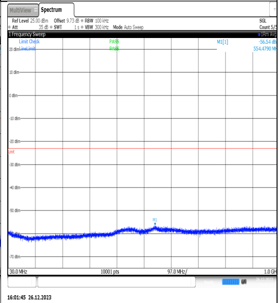
NTNV_N77-3450- 3550_PC2_30_15_L_TID10_NS_01_30_1000_#1
