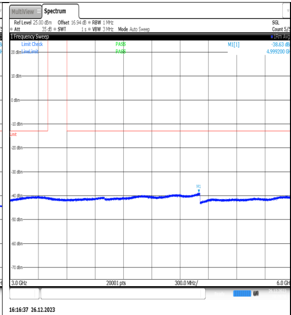
NTNV_N77-3450- 3550_PC2_30_15_L_TID14_NS_01_3000_6000_ #1
