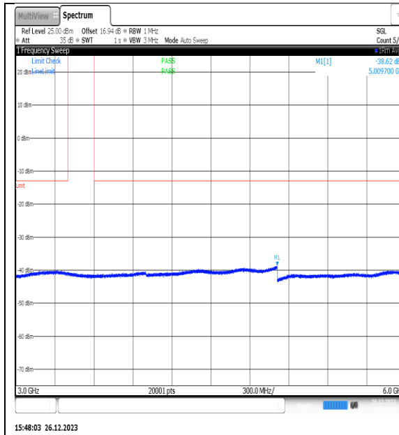
NTNV_N77-3450- 3550_PC2_30_15_L_TID7_NS_01_3000_6000_# 1
