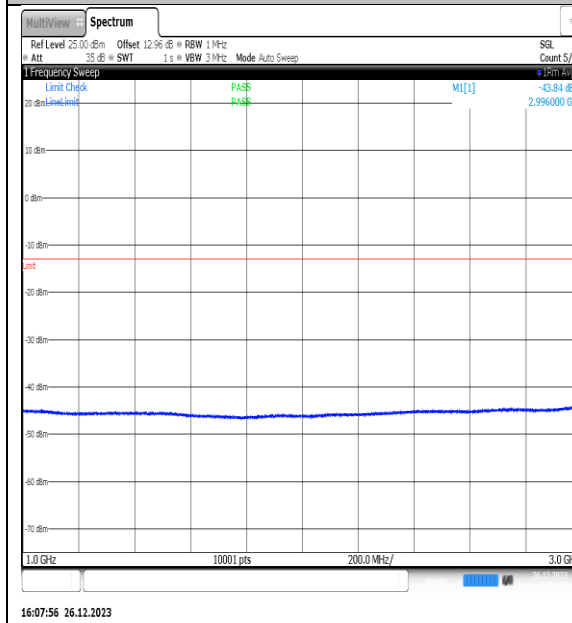
NTNV_N77-3450-3550_PC2_30_15_L_TID12_NS_01_1000_3000_#1
