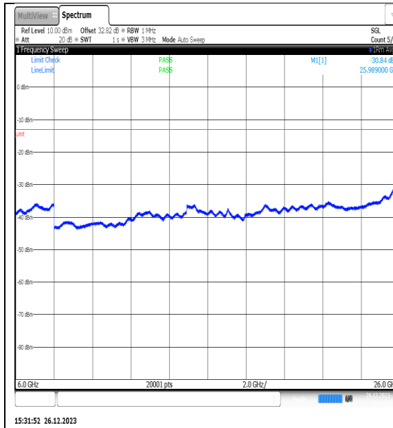
NTNV_N77-3450- 3550_PC2_30_15_L_TID4_NS_01_6000_26000_ #1
