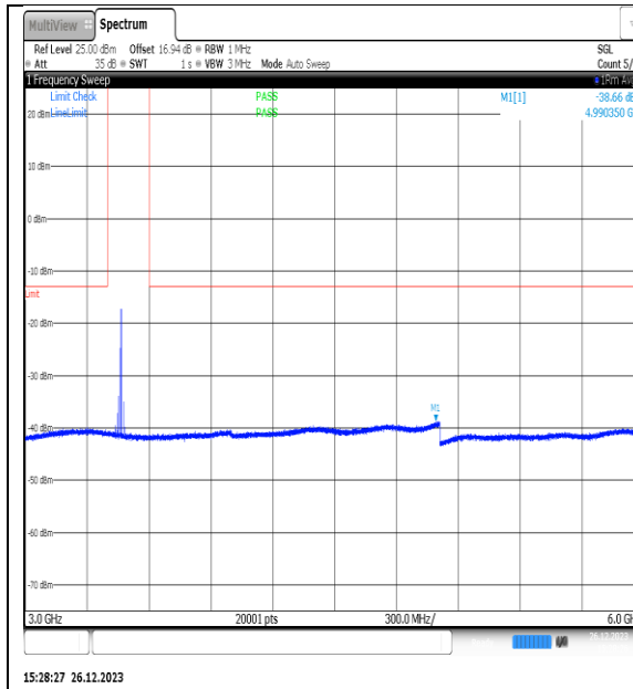
NTNV_N77-3450- 3550_PC2_30_15_L_TID3_NS_01_3000_6000_# 1
