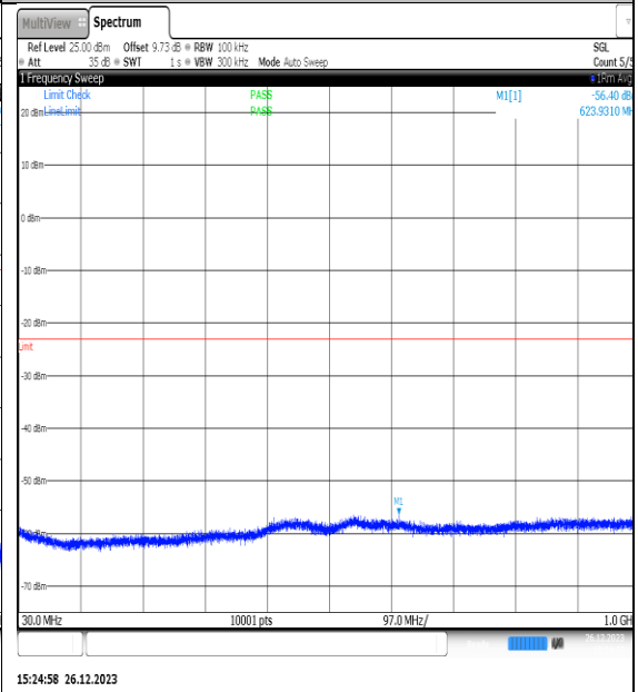
NTNV_N77-3450- 3550_PC2_30_15_L_TID2_NS_01_30_1000_#1
