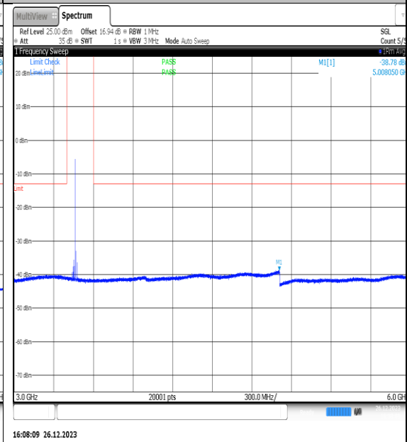
NTNV_N77-3450-3550_PC2_30_15_L_TID12_NS_01_3000_6000_#1
