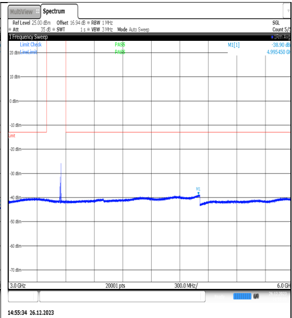
NTNV_N77-3450- 3550_PC2_30_10_H_TID9_NS_01_3000_6000_# 1
