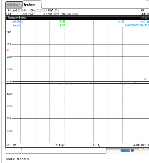
NTNV_N77-3450- 3550_PC2_30_15_L_TID15_NS_01_26000_4000_ 0_#1
