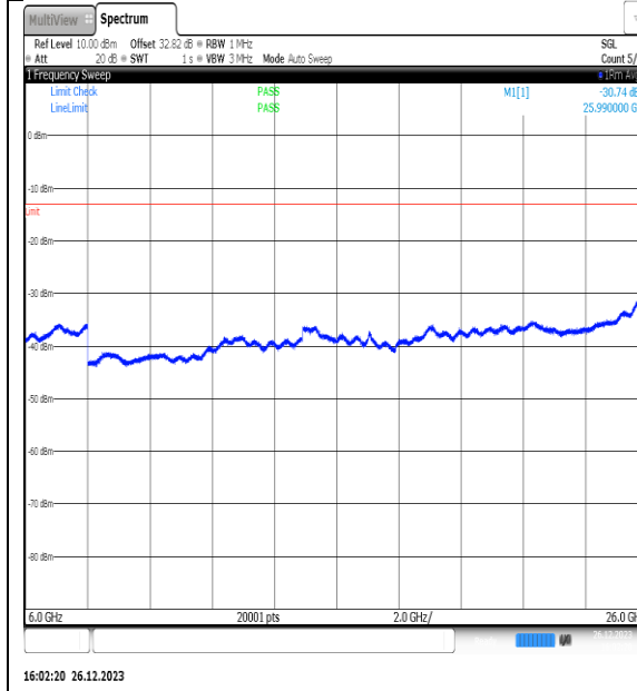
NTNV_N77-3450- 3550_PC2_30_15_L_TID10_NS_01_6000_26000_ #1
