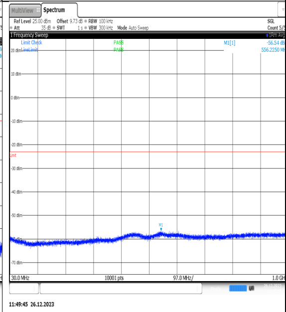
NTNV_N77-3450- 3550_PC2_30_10_L_TID15_NS_01_30_1000_#1
