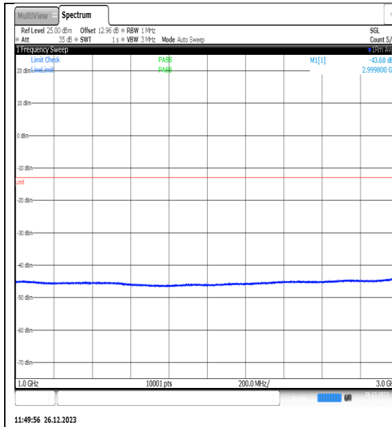
NTNV_N77-3450- 3550_PC2_30_10_L_TID15_NS_01_1000_3000_ #1
