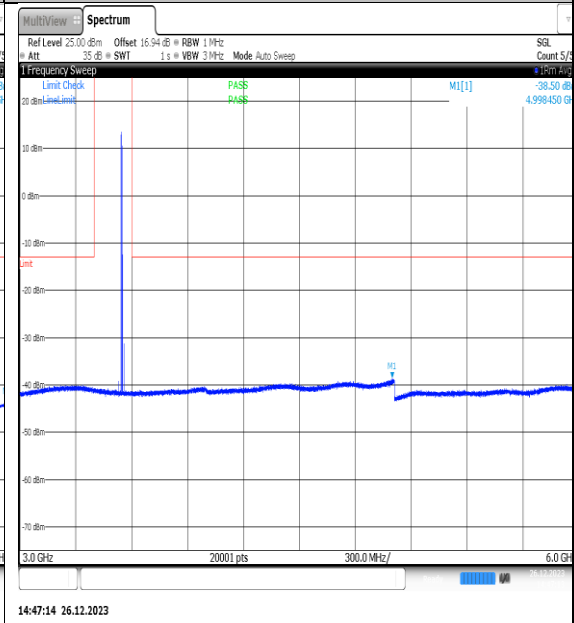
NTNV_N77-3450- 3550_PC2_30_10_H_TID7_NS_01_3000_6000_# 1
