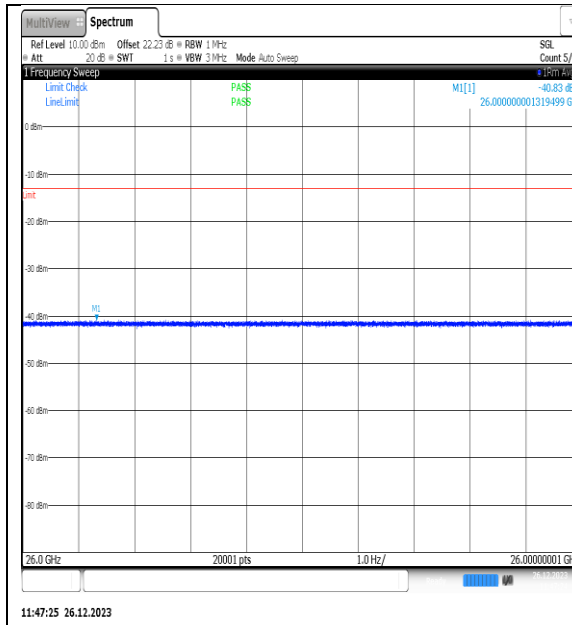
NTNV_N77-3450- 3550_PC2_30_10_L_TID14_NS_01_26000_4000 0_#1
