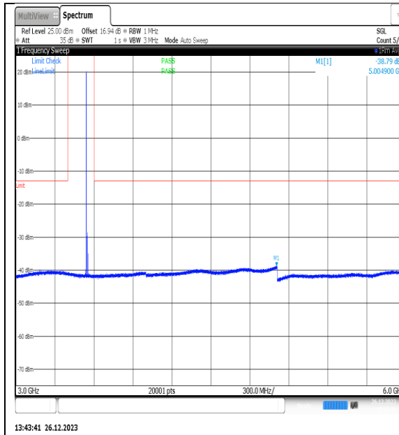
NTNV_N77-3450- 3550_PC2_30_10_H_TID2_NS_01_3000_6000_# 1
