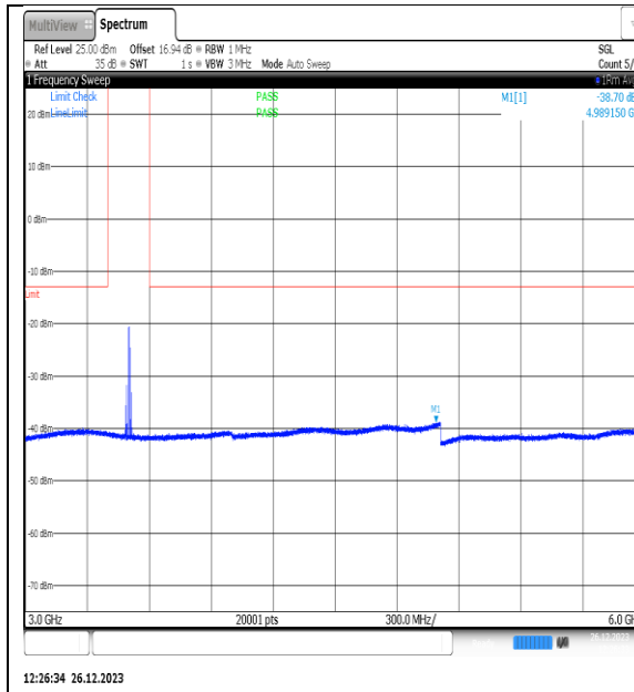
NTNV_N77-3450- 3550_PC2_30_10_M_TID9_NS_01_3000_6000_# 1
