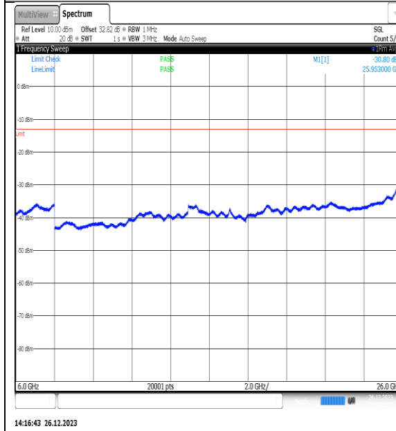
NTNV_N77-3450- 3550_PC2_30_10_H_TID5_NS_01_6000_26000_# 1
