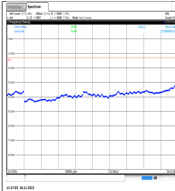
NTNV_N77-3450- 3550_PC2_30_10_M_TID6_NS_01_6000_26000_#1
