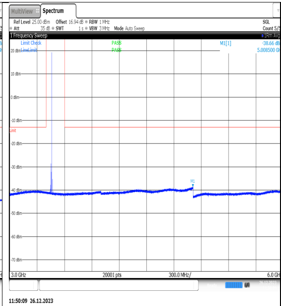
NTNV_N77-3450- 3550_PC2_30_10_L_TID15_NS_01_3000_6000_ #1
