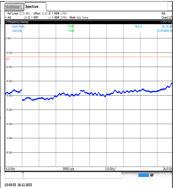
NTNV_N77-3450- 3550_PC2_30_10_H_TID2_NS_01_6000_26000_# 1
