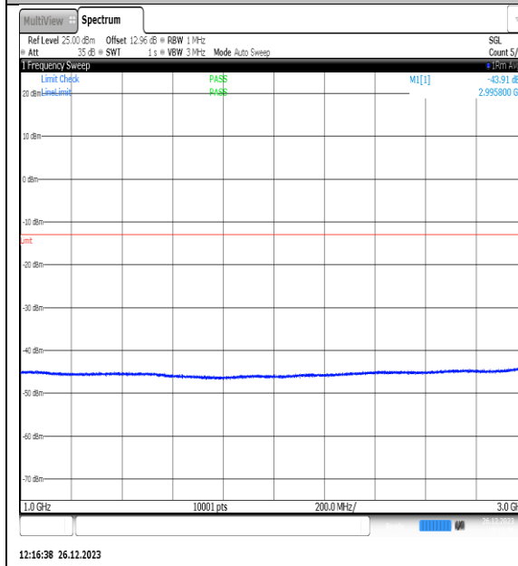
NTNV_N77-3450- 3550_PC2_30_10_M_TID6_NS_01_1000_3000_#
