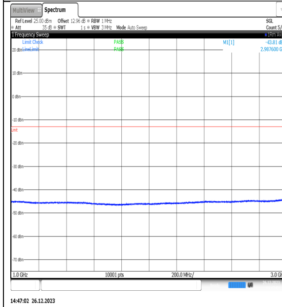
NTNV_N77-3450- 3550_PC2_30_10_H_TID7_NS_01_1000_3000_# 1
