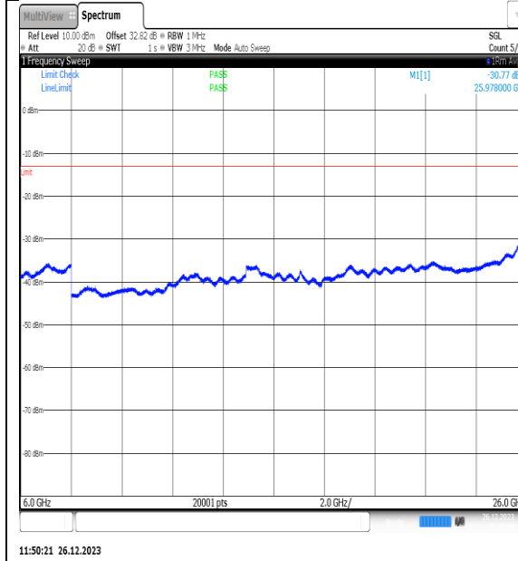
NTNV_N77-3450- 3550_PC2_30_10_L_TID15_NS_01_6000_26000 #1
