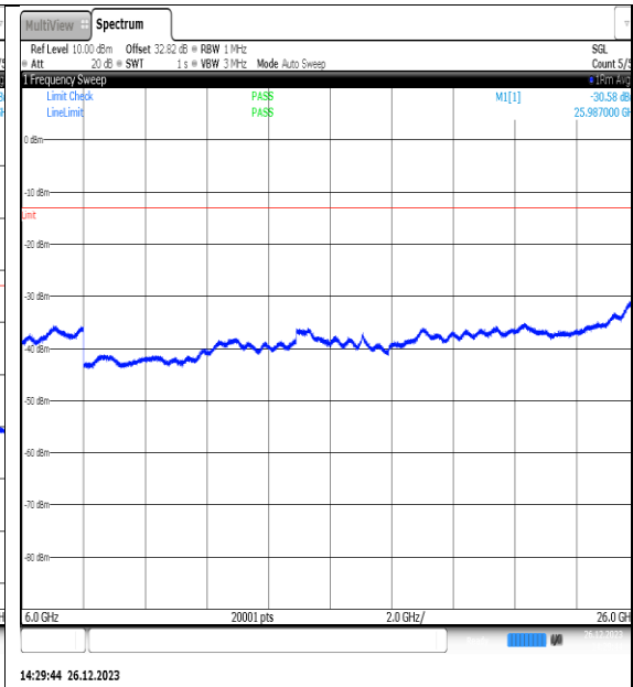
NTNV_N77-3450- 3550_PC2_30_10_H_TID6_NS_01_6000_26000_# #1
