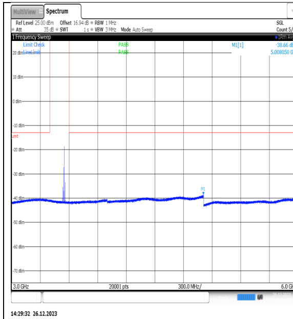
NTNV_N77-3450- 3550_PC2_30_10_H_TID6_NS_01_3000_6000_# 1
