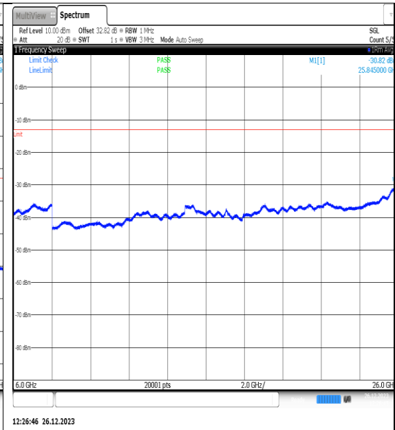
NTNV_N77-3450- 3550_PC2_30_10_M_TID9_NS_01_6000_26000_# 1
