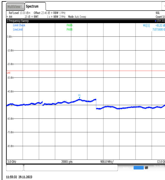
NTVN_N7_PC3_15_25_L_TID2_NS_01_3000_12_000_#1
