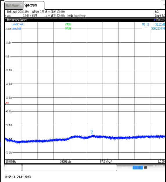
NTVN_N7_PC3_15_25_L_TID2_NS_01_30_1000_#1
