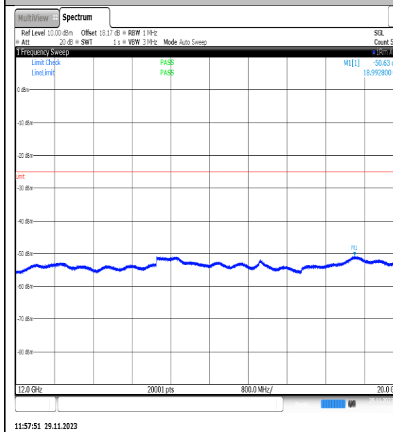
NTVN_N7_PC3_15_25_L_TID3_NS_01_12000_2 0000_#1
