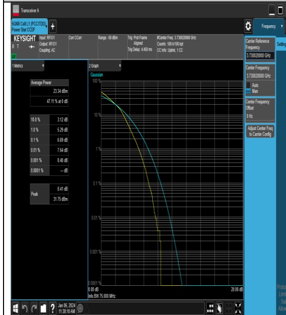
NTNV_N77-3700-3980_PC2_30_60_L_TID3_#1
