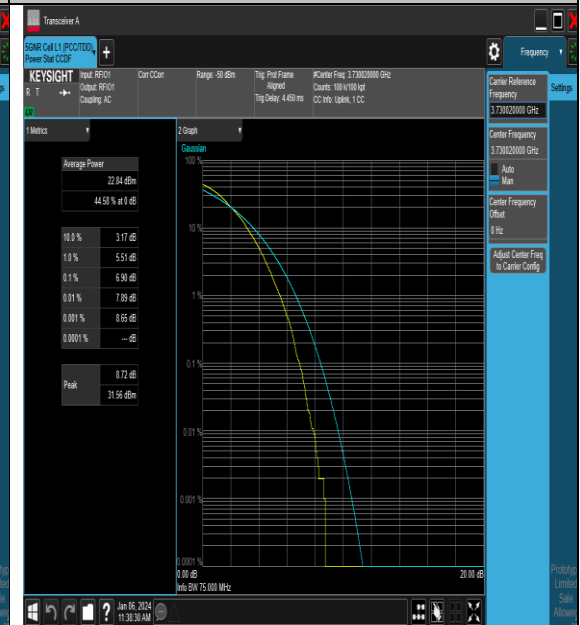
NTNV_N77-3700-3980_PC2_30_60_L_TID4_#1
