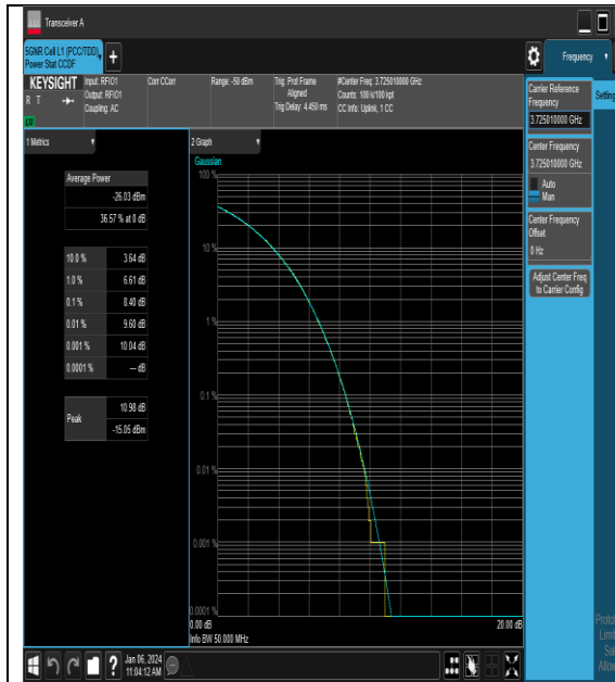
NTNV_N77-3700-3980_PC2_30_50_L_TID4_#1
