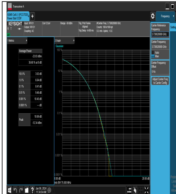
NTNV_N77-3700-3980_PC2_30_60_L_TID1_#1
