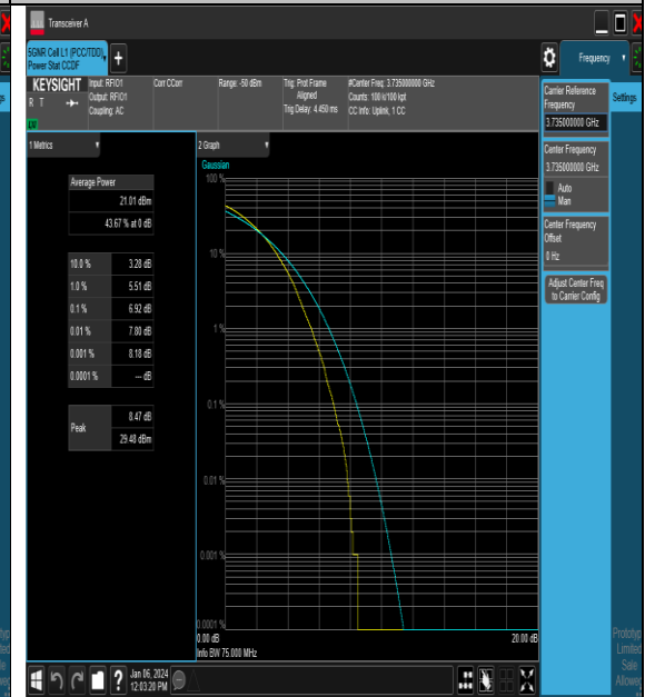
NTNV_N77-3700-3980_PC2_30_70_L_TID5_#1
