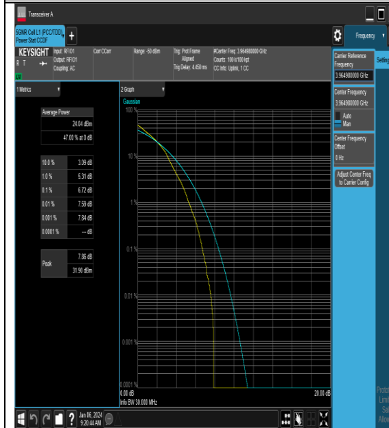
NTNV_N77-3700-3980_PC2_30_30_H_TID3_#1
