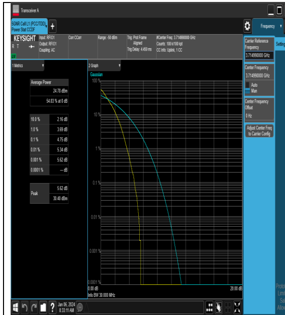
NTNV_N77-3700-3980_PC2_30_30_L_TID1_#1
