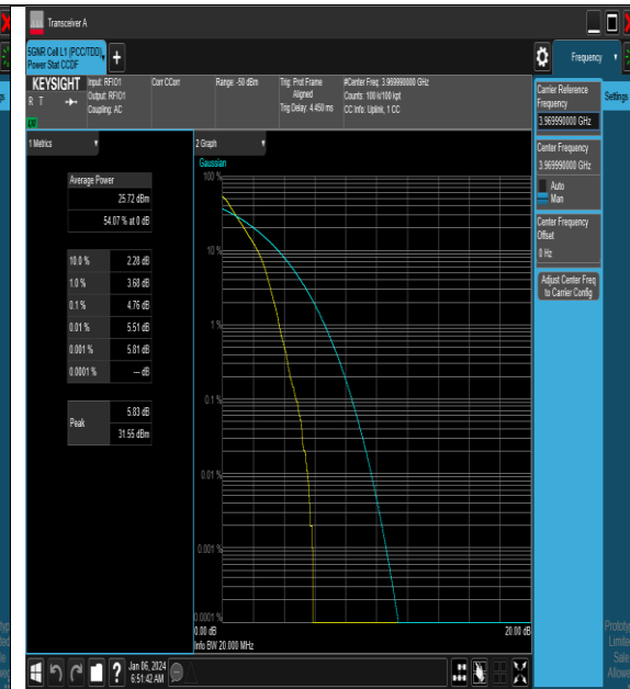
NTNV_N77-3700-3980_PC2_30_20_H_TID1_#1
