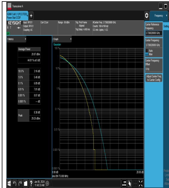
NTNV_N77-3700-3980_PC2_30_60_L_TID5_#1
