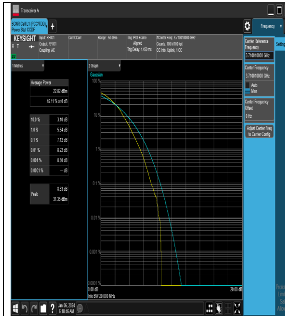
NTNV_N77-3700-3980_PC2_30_20_L_TID4_#1
