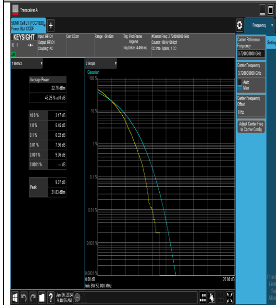
NTNV_N77-3700-3980_PC2_30_40_L_TID4_#1
