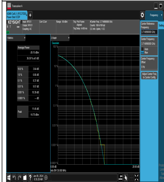
NTNV_N77-3700-3980_PC2_30_30_L_TID3_#1
