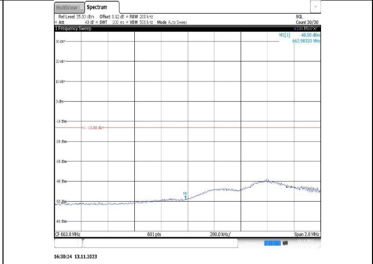
Band71-10MHz-QPSK-133422-1RB#0
