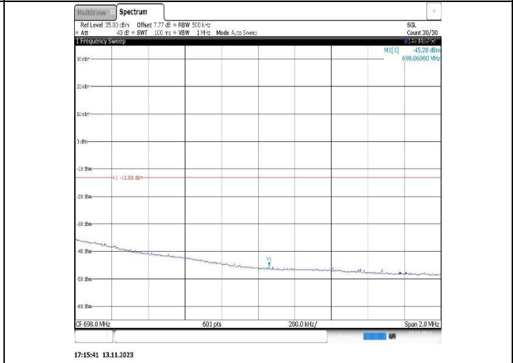
Band71-20MHz-QPSK-133372-100RB#0
