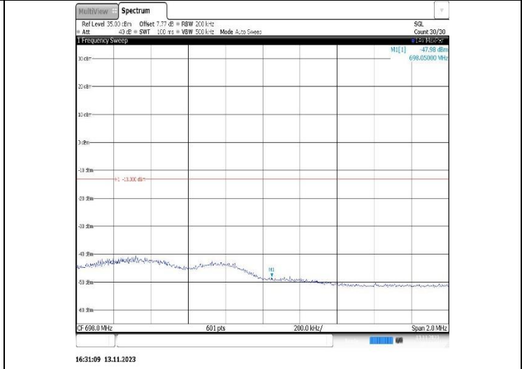
Band71-10MHz-QPSK-133422-50RB#0
