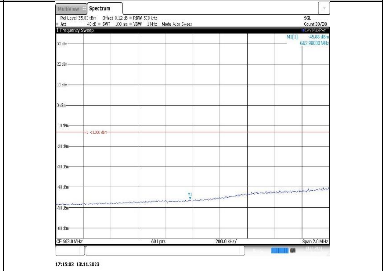
Band71-20MHz-16QAM-133372-1RB#0
