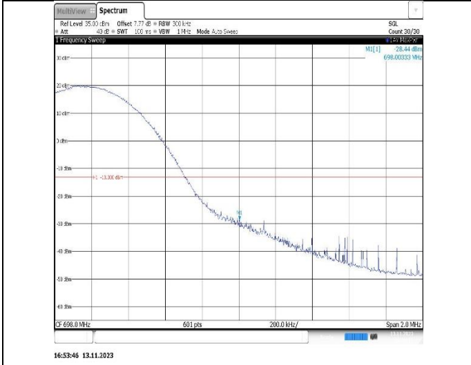
Band71-20MHz-QPSK-133222-1RB#0
