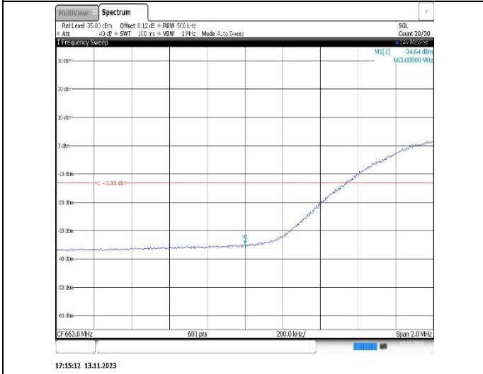
Band71-20MHz-QPSK-133372-1RB#99
