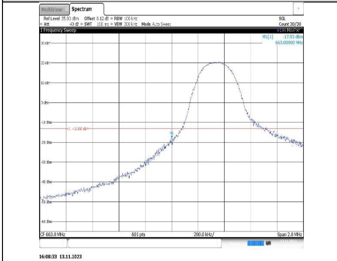
Band71-5MHz-QPSK-133147-25RB#0
