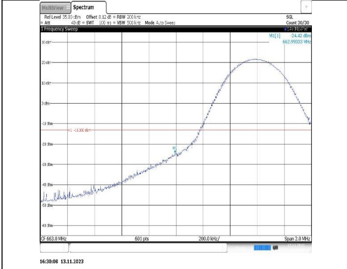
Band71-10MHz-QPSK-133172-50RB#0
