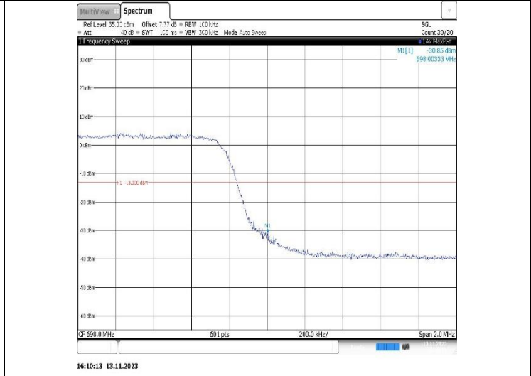
Band71-10MHz-QPSK-133172-1RB#49
