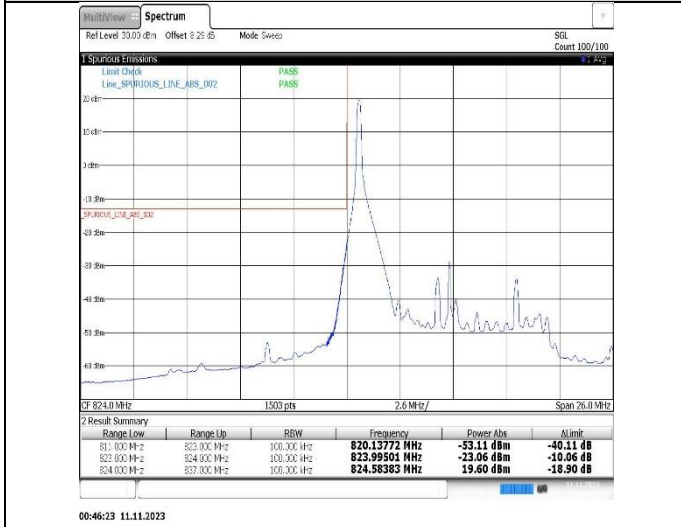
Band5-10MHz-QPSK-20450-1RB#0
