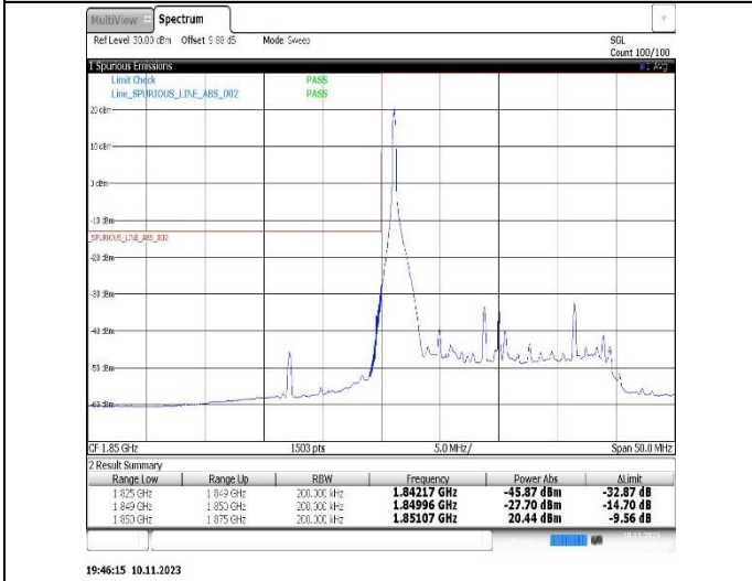
Band2-20MHz-QPSK-18700-1RB#0
