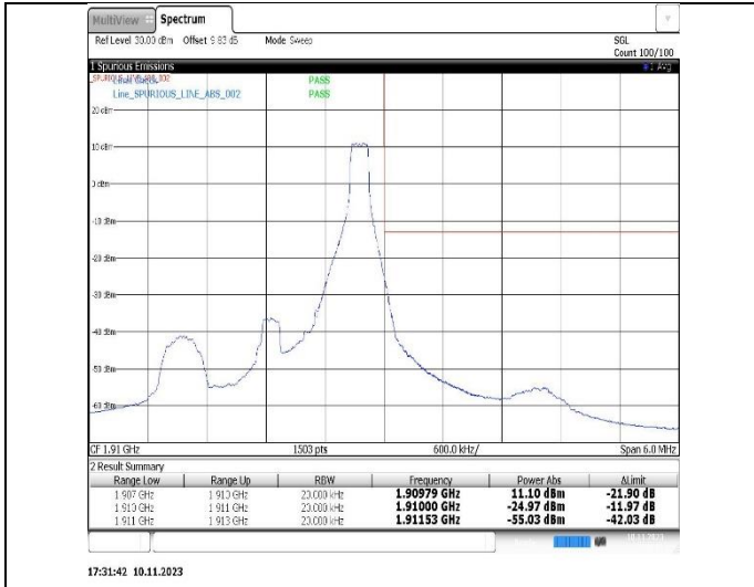
Band2-3MHz-QPSK-18615-1RB#0
