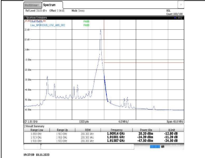
Band2-15MHz-16QAM-19125-1RB#74
