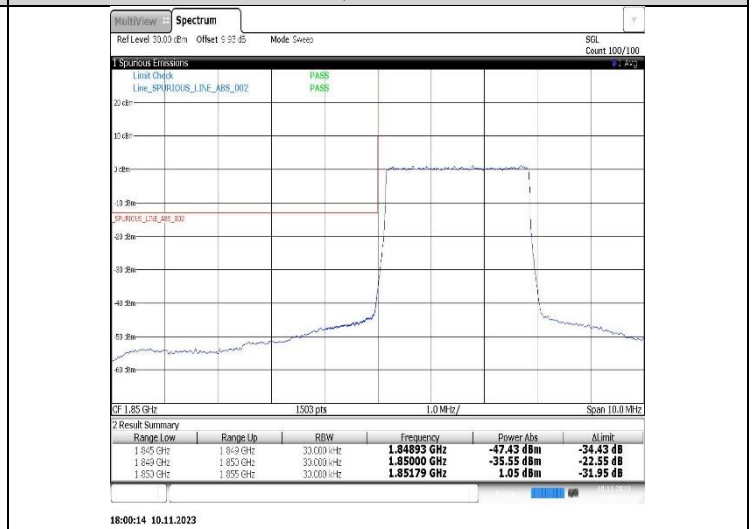
Band2-3MHz-QPSK-19185-15RB#0
