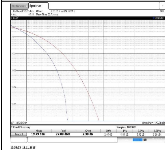
Band25-10MHz-QPSK-26365-50RB#0
