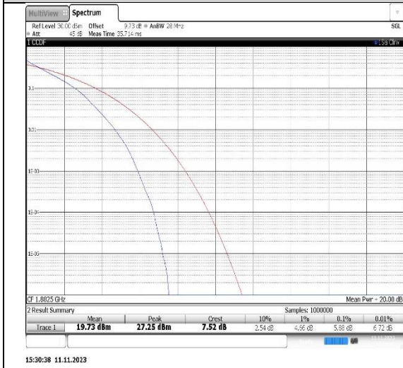
Band25-5MHz-QPSK-26365-25RB#0
