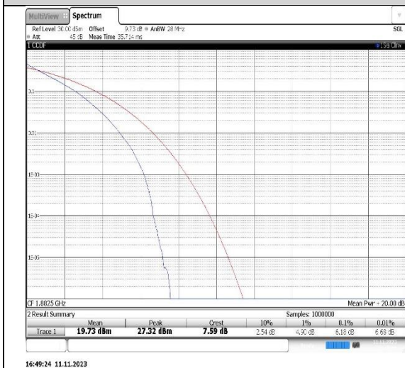
Band25-20MHz-QPSK-26365-100RB#0
