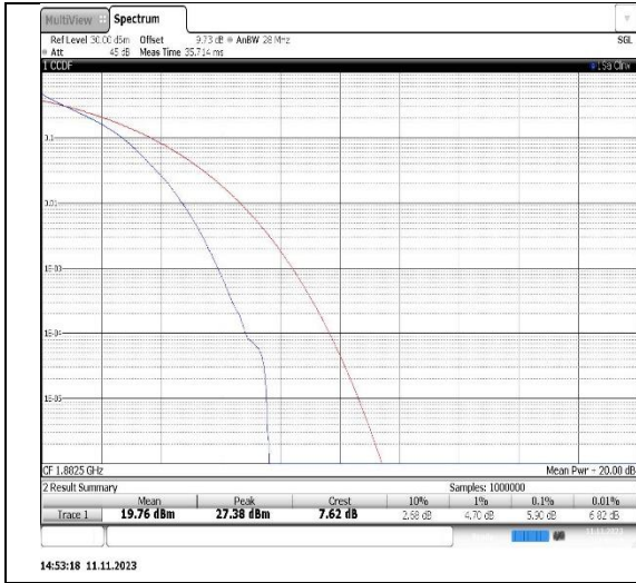
Band25-3MHz-QPSK-26365-15RB#0
