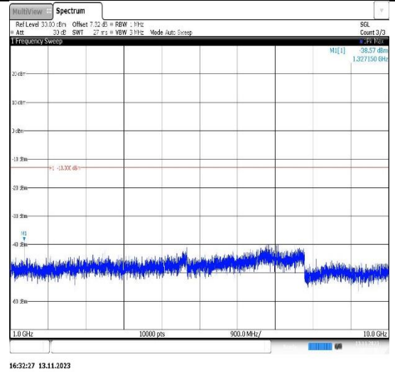
Band71-10MHz-QPSK-133297-1RB#0-Range2:1000~10000MHz
