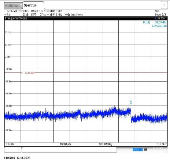
Band26(824-849)-5MHz-QPSK-26915-1RB#0-Range2:1000~10000MHz
