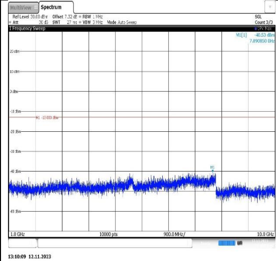
Band26(824-849)-1.4MHz-QPSK-27033-1RB#0-Range2:1000~10000MHz
