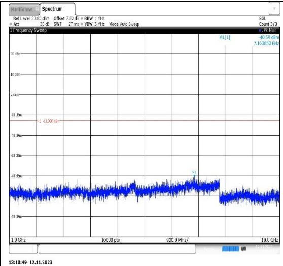
Band26(824-849)-1.4MHz-16QAM-26797-1RB#0-Range2:1000~10000MHz
