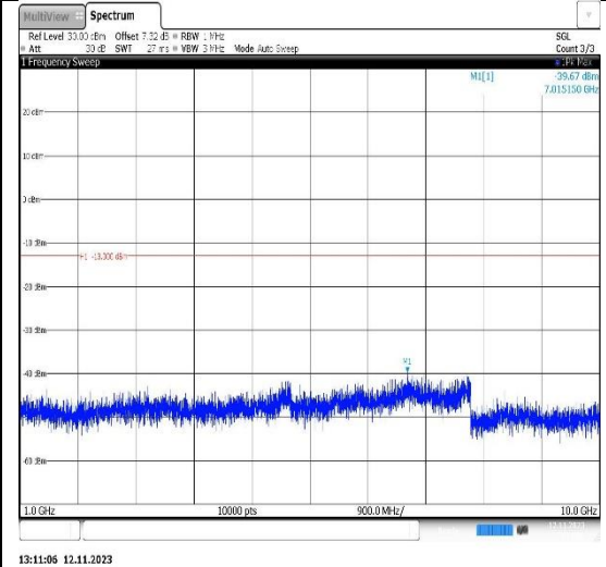
Band26(824-849)-3MHz-QPSK-26805-1RB#0-Range2:1000~10000MHz
