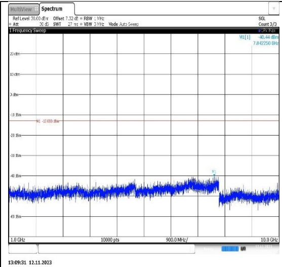
Band26(824-849)-1.4MHz-QPSK-26915-1RB#0-Range2:1000~10000MHz
