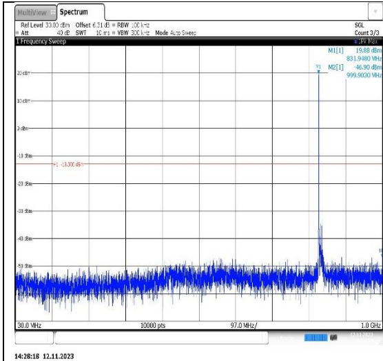
Band26(824-849)-10MHz-16QAM-26990-1RB#0-Range1:30~1000MHz
