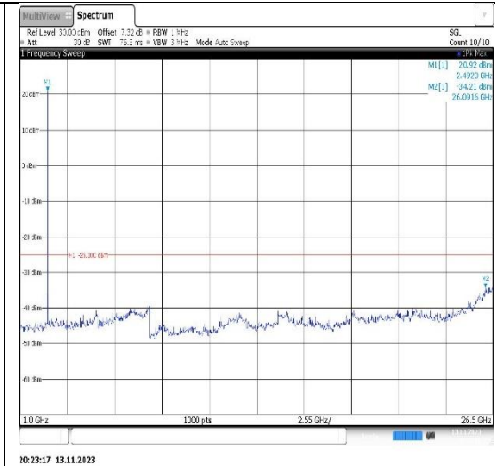
Band41-5MHz-QPSK-40620-1RB#0- Range2:1000~26500MHz
