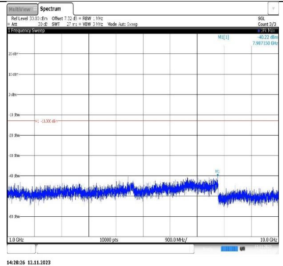
Band26(824-849)-10MHz-16QAM-26990-1RB#0-Range2:1000~10000MHz
