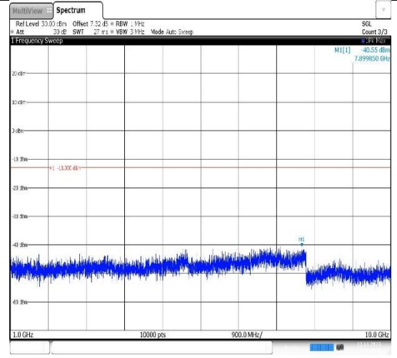
Band26(824-849)-5MHz-QPSK-26915-1RB#0-Range2:1000~10000MHz
