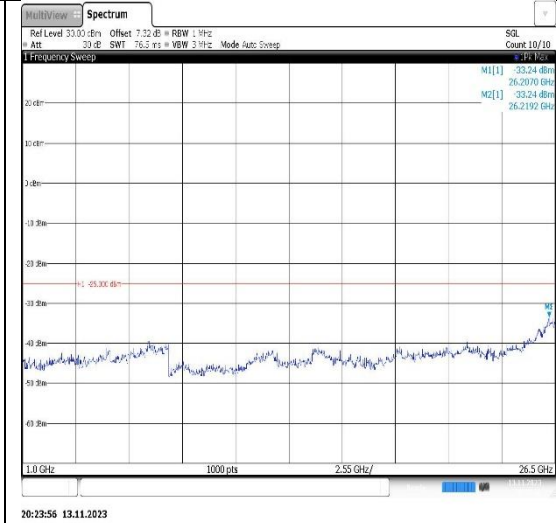
Band41-5MHz-QPSK-41565-1RB#0- Range2:1000~26500MHz
