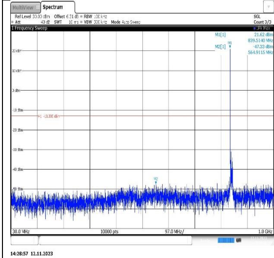
Band26(824-849)-15MHz-QPSK-26865-1RB#0-Range1:30~1000MHz
