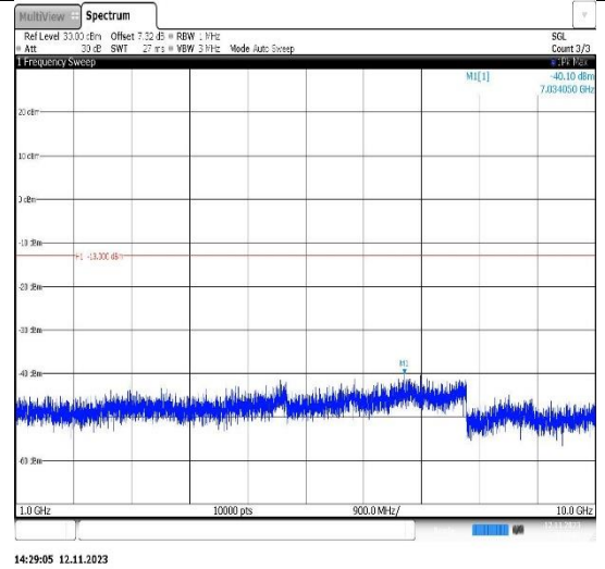
Band26(824-849)-15MHz-QPSK-26865-1RB#0-Range2:1000~10000MHz
