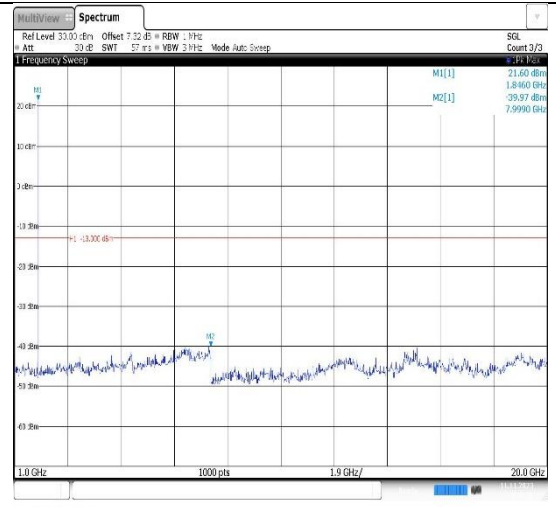
Band25-1.4MHz-QPSK-26365-1RB#0-Range2:1000~20000MHz
