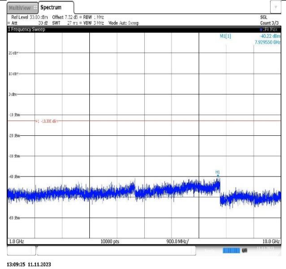
Band12-5MHz-QPSK-23155-1RB#0- Range2:1000~10000MHz
