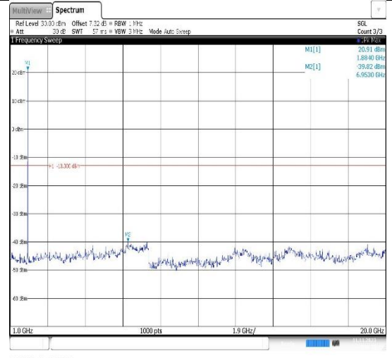
Band25-1.4MHz-QPSK-26683-1RB#0-Range2:1000~20000MHz
