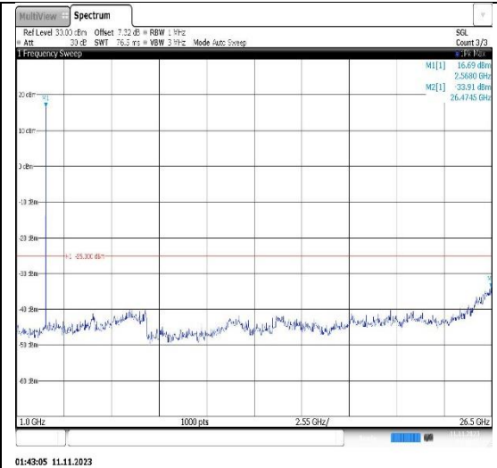
Band7-10MHz-16QAM-20800-1RB#0- Range2:1000~26500MHz
