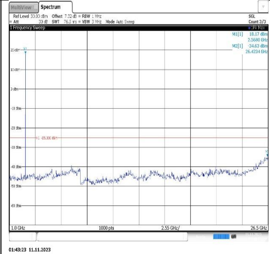
Band7-15MHz-QPSK-20825-1RB#0- Range2:1000~26500MHz
