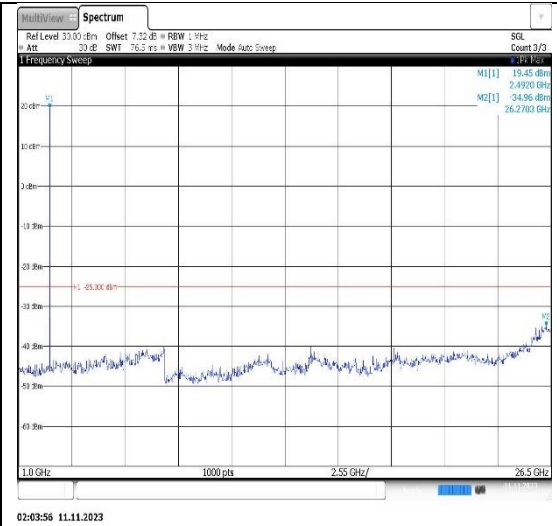
Band7-15MHz-QPSK-21100-1RB#0- Range2:1000~26500MHz
