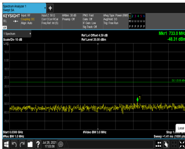
Band41-20MHz-QPSK-40140:30~1000MHz
