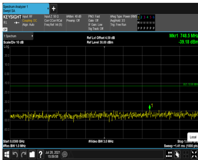
Band25-20MHz-QPSK-26365:30~1000MHz
