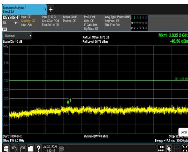
Band13-5MHz-QPSK-23230:1000~10000MHz
