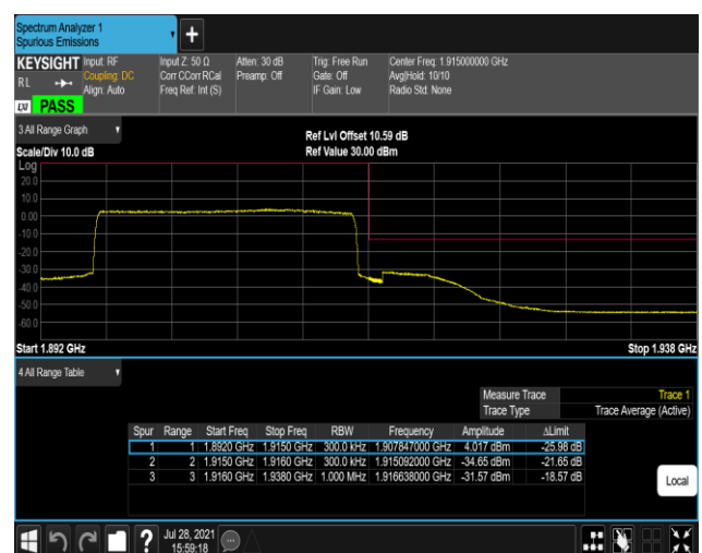
Band25-20MHz-QPSK-26590-100RB#0
