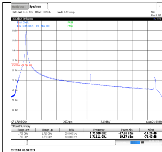
Band66-20MHz-QPSK-132072-1RB#99-PASS
