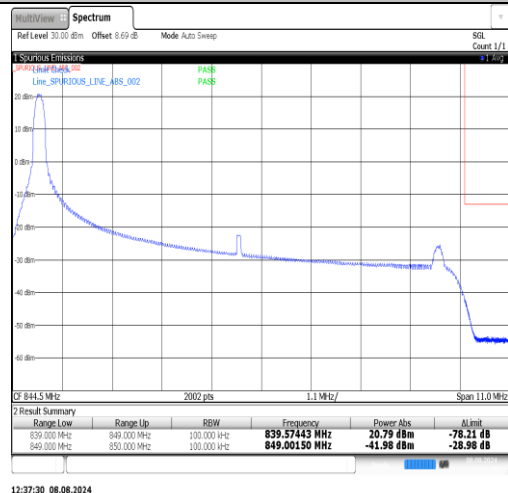
Band26(824-849)-10MHz-QPSK-26990-1RB#49-PASS
