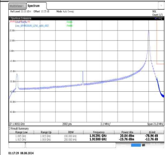
Band25-20MHz-16QAM-26590-1RB#99-PASS
