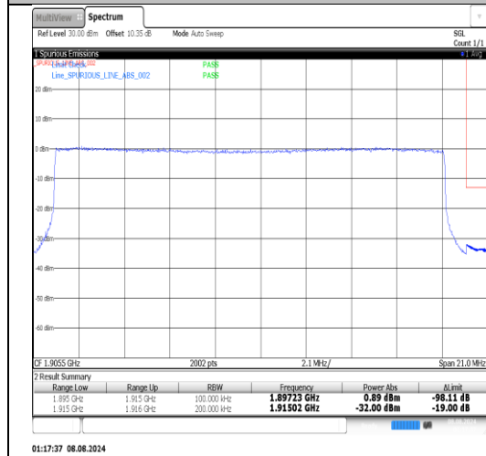
Band25-20MHz-QPSK-26590-100RB#0-PASS
