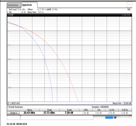
Band25-20MHz-16QAM-26365-100RB#0-PASS
