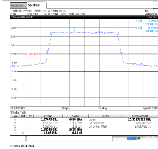
Band25-20MHz-QPSK-26365-100RB#0-PASS
