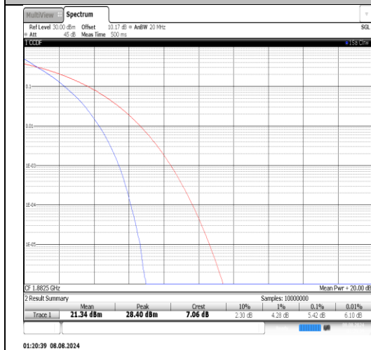
Band25-20MHz-QPSK-26365-100RB#0-PASS
