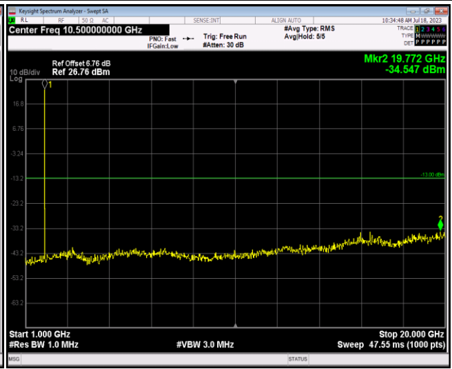
Band25-1.4MHz-16QAM-26365-1RB#0-Range2:1000 ~20000MHz
