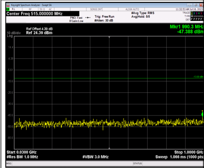
Band25-20MHz-QPSK-26140-1RB#0-Range1:30~1 000MHz
