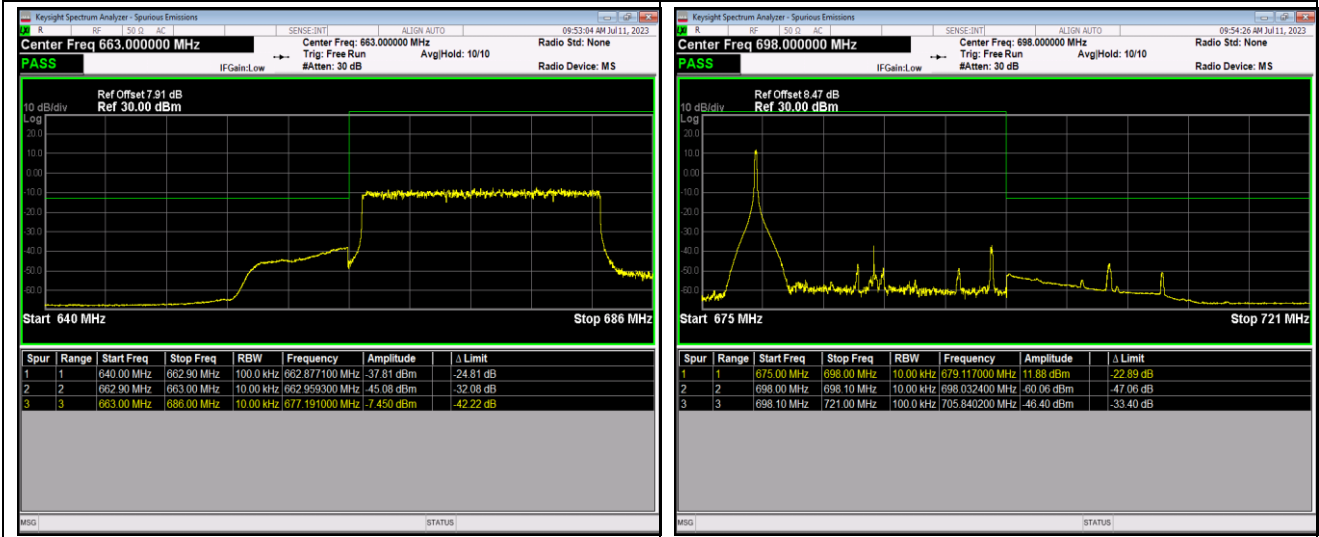
Band71-20MHz-QPSK-133372-1RB#99
