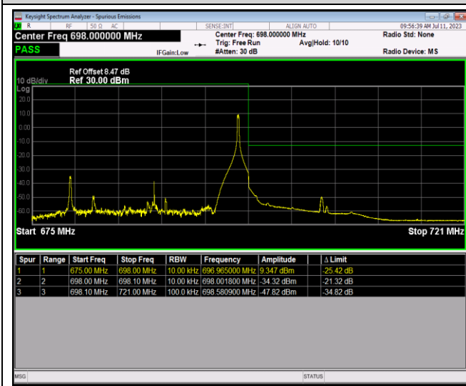
Band71-20MHz-64QAM-133372-1RB#99
