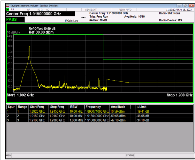
Band25-20MHz-QPSK-26590-100RB#0
