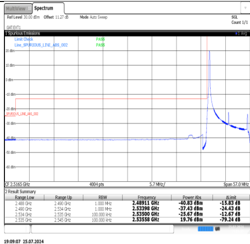
Band41(2535-2655)-10MHz-16QAM-40090-1RB#49-PASS
