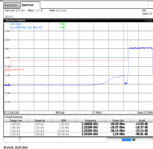
Band41(2535-2655)-10MHz-16QAM-41190-1RB#0-PASS
