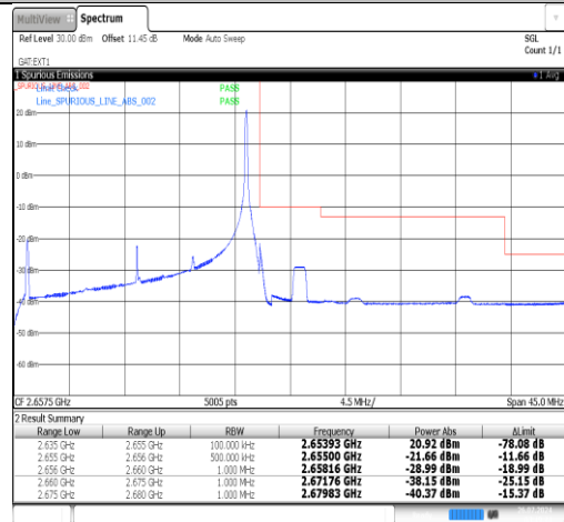
Band41(2535-2655)-20MHz-QPSK-41140-1RB#99-PASS
