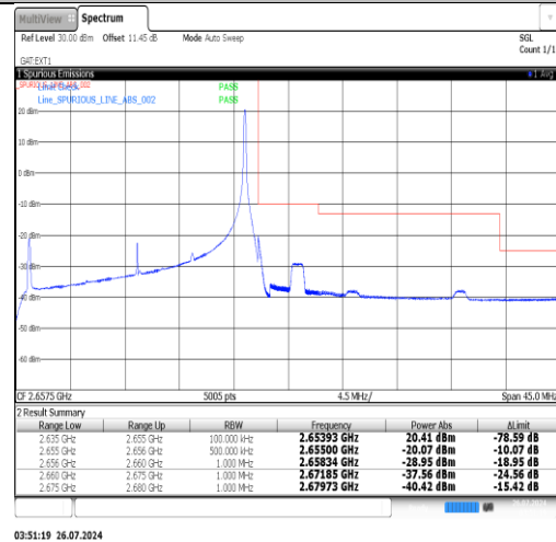
Band41(2535-2655)-20MHz-16QAM-41140-1RB#99-PASS
