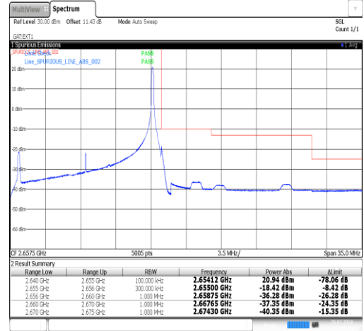
Band41(2535-2655)-15MHz-QPSK-41165-1RB#74-PASS
