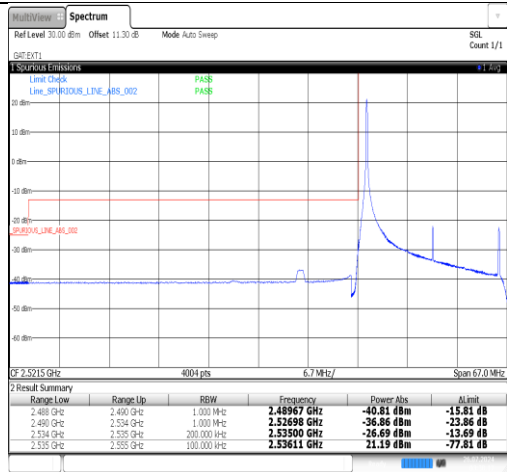
Band41(2535-2655)-20MHz-QPSK-40140-1RB#99-PASS
