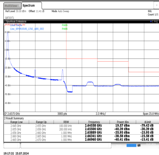
Band41(2535-2655)-10MHz-16QAM-41190-1RB#49-PASS
