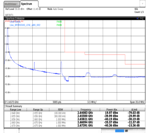
Band41(2535-2655)-15MHz-QPSK-41165-1RB#0-PASS
