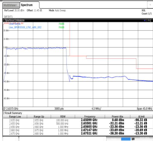
Band41(2535-2655)-20MHz-QPSK-41140-100RB#0-PASS
