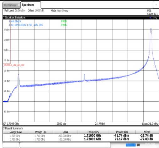
Band66-20MHz-QPSK-132072-1RB#99-PASS
