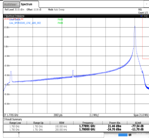
Band66-20MHz-QPSK-132572-1RB#99-PASS
