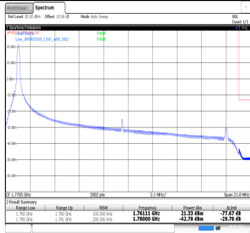
Band66-20MHz-QPSK-132572-1RB#0-PASS
