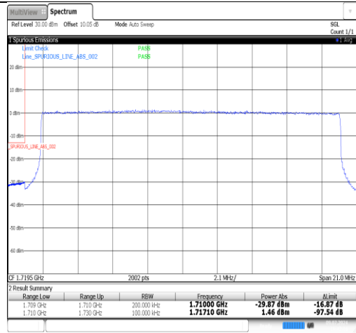
Band66-20MHz-QPSK-132572-1RB#0-PASS
