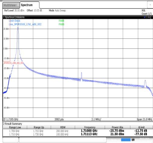
Band66-20MHz-QPSK-132072-1RB#99-PASS
