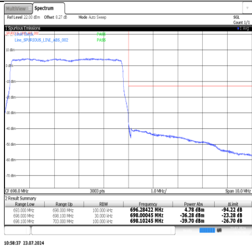
Band71-10MHz-QPSK-133172-1RB#0-PASS
