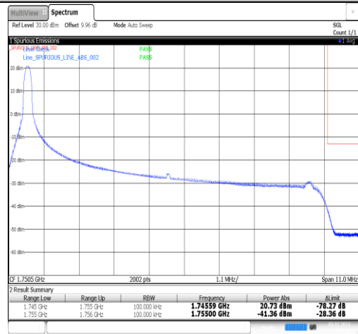
Band4-10MHz-QPSK-20350-1RB#49-PASS
