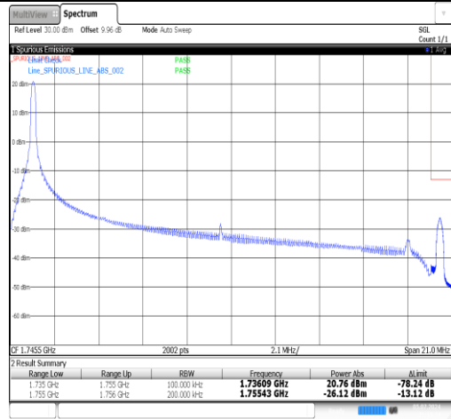
Band4-20MHz-QPSK-20300-1RB#99-PASS
