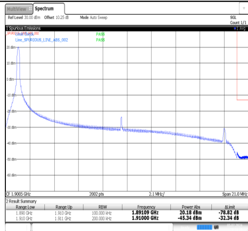
Band2-20MHz-16QAM-19100-1RB#99-PASS
