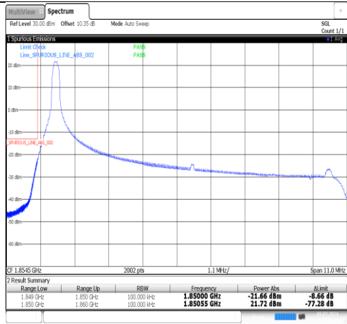
Band2-10MHz-QPSK-18650-1RB#49-PASS
