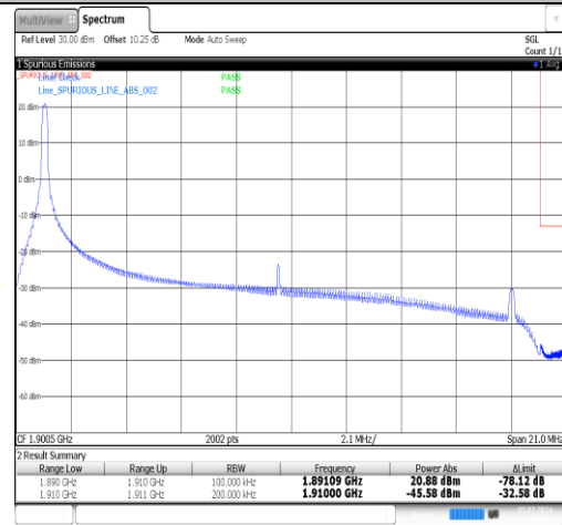
Band2-20MHz-QPSK-19100-1RB#99-PASS
