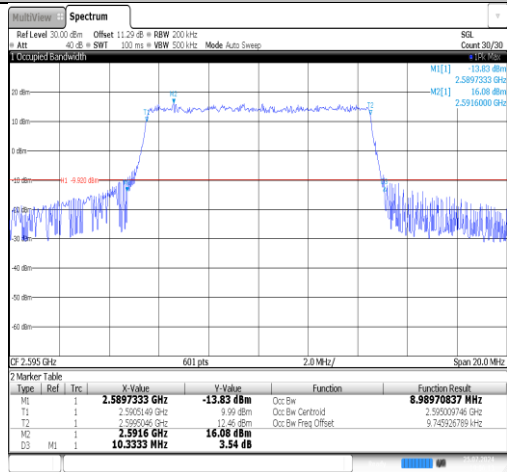
Band41(2535-2655)-10MHz-QPSK-40640-50RB#0-PASS
