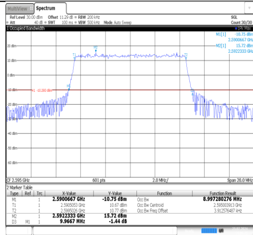
Band41(2535-2655)-10MHz-16QAM-40640-50RB#0-PASS
