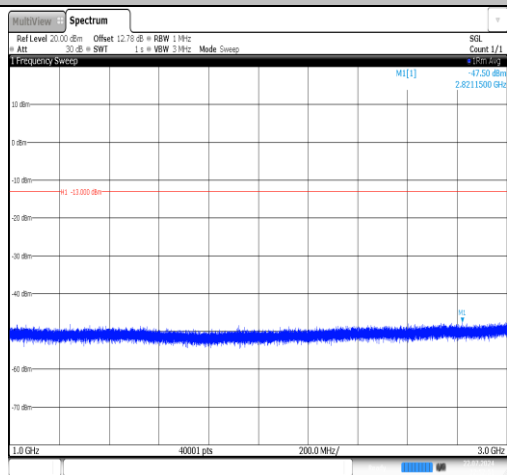
Band26(824-849)-3MHz-QPSK-26915-1RB#0-1000~3000-PASS
