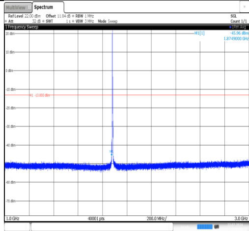
Band25-3MHz-QPSK-26365-1RB#0-1000~3000-PASS
