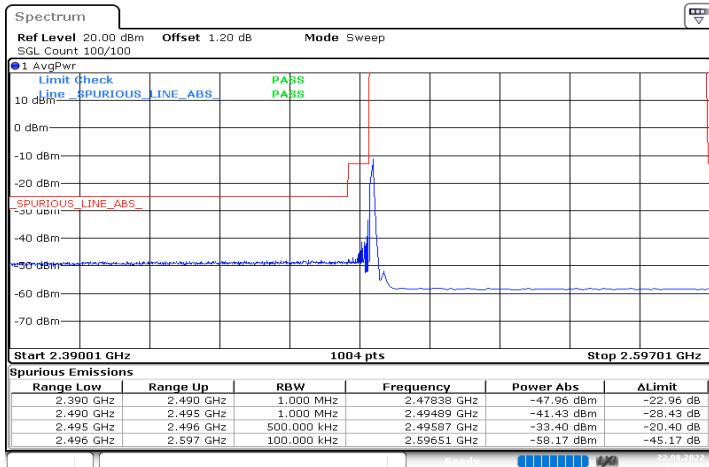
n41_40MHz_30kHz_2516.01MHz_DFT-s-OFDM QPSK_RB1@0
