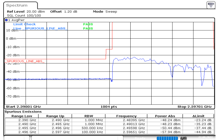
n41_100MHz_30kHz_2546.01MHz_DFT-s-OFDM QPSK_RB270@0
