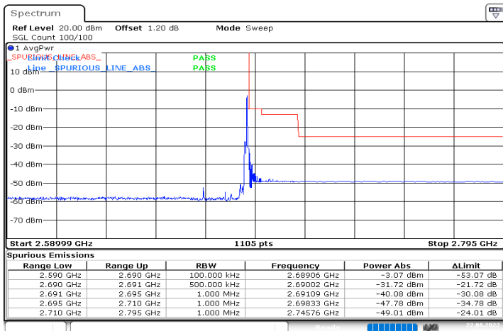
n41_20MHz_30kHz_2679.99MHz_DFT-s-OFDM QPSK_RB1@50
