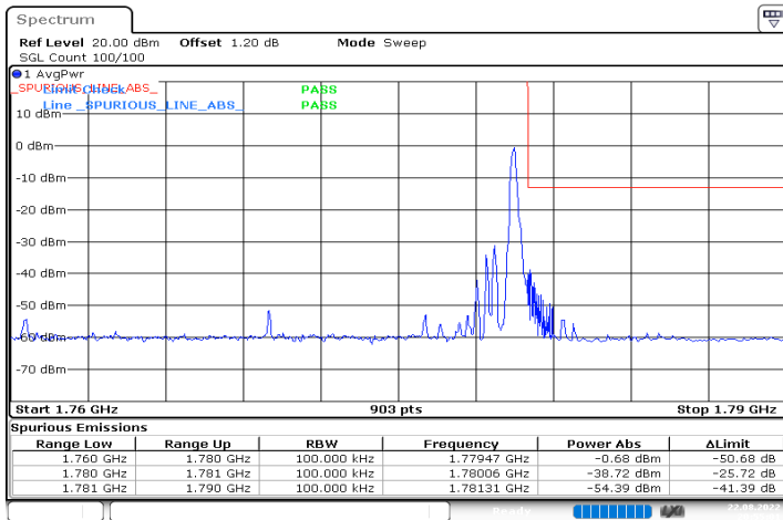
n66_20MHz_15kHz_1770MHz_DFT-s-OFDM QPSK_RB1@105
