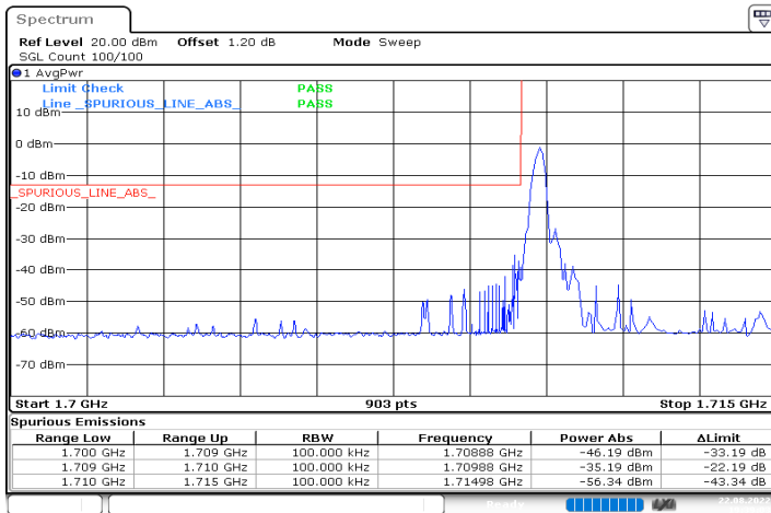
n66_5MHz_15kHz_1712.5MHz_DFT-s-OFDM QPSK_RB1@0
