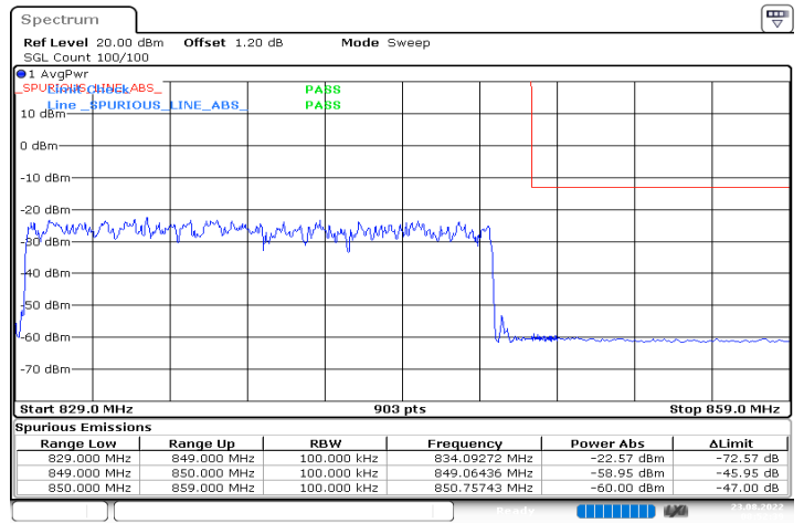
n5_20MHz_15kHz_839MHz_DFT-s-OFDM QPSK_RB100@0
