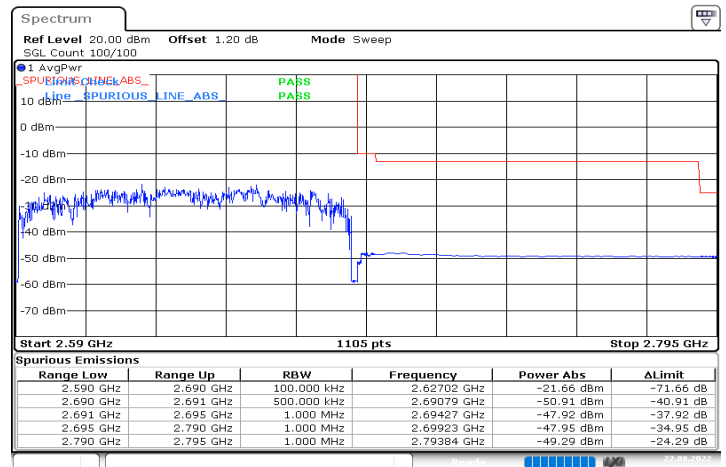
n41_100MHz_30kHz_2640MHz_DFT-s-OFDM QPSK_RB270@0
