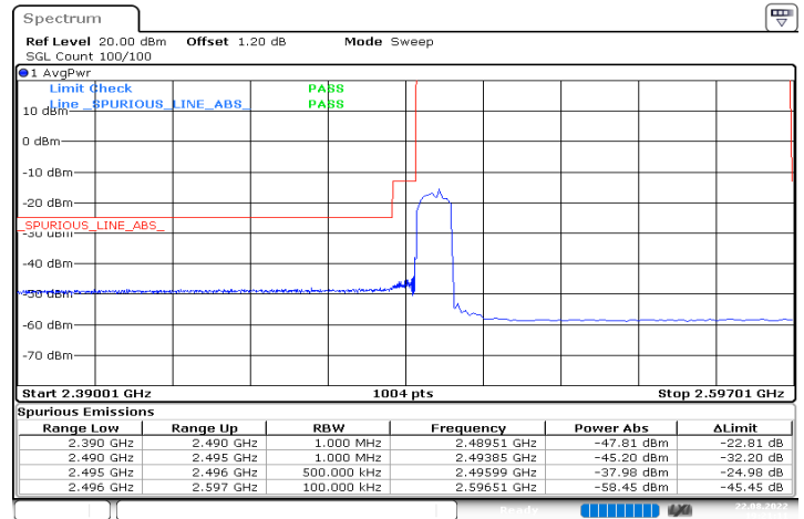
n41_10MHz_30kHz_2501.01MHz_DFT-s-OFDM QPSK_RB24@0
