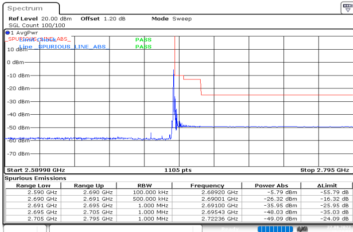
n41_15MHz_30kHz_2682.48MHz_DFT-s-OFDM QPSK_RB1@37
