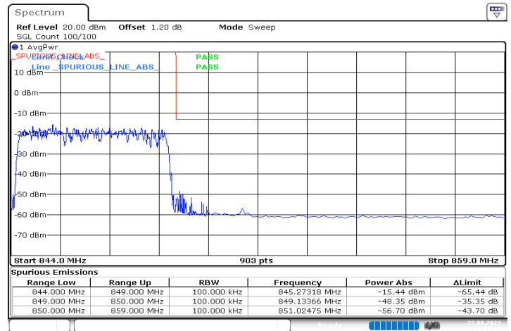
n5_5MHz_15kHz_846.5MHz_DFT-s-OFDM QPSK_RB25@0
