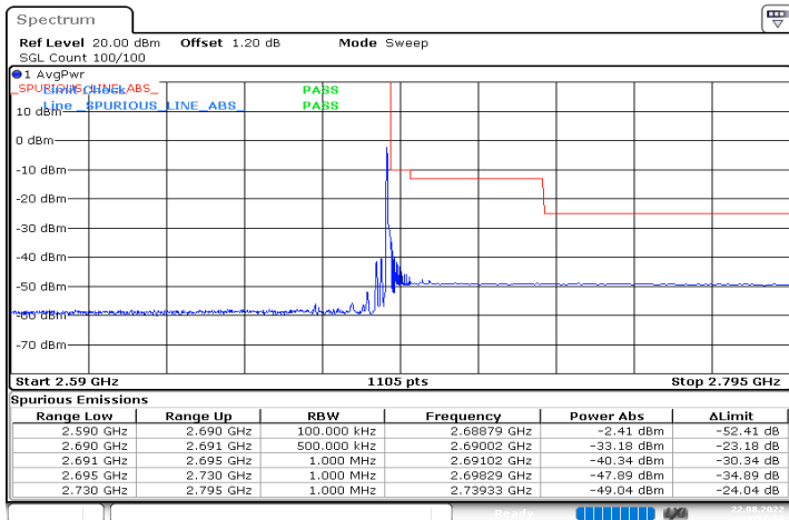
n41_40MHz_30kHz_2670MHz_DFT-s-OFDM QPSK_RB1@105
