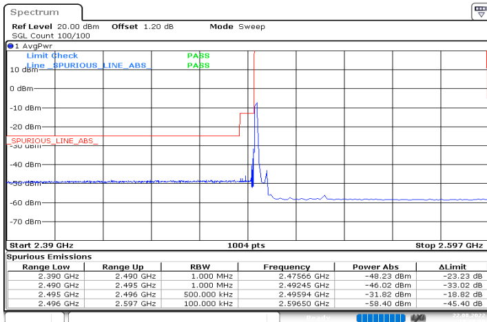
n41_60MHz_30kHz_2526MHz_DFT-s-OFDM QPSK_RB1@0
