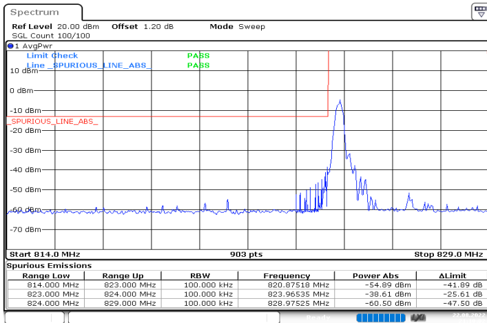
n5_5MHz_15kHz_826.5MHz_DFT-s-OFDM QPSK_RB1@0
