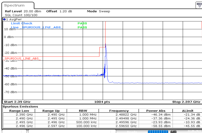
n41_15MHz_30kHz_2503.5MHz_DFT-s-OFDM QPSK_RB1@0
