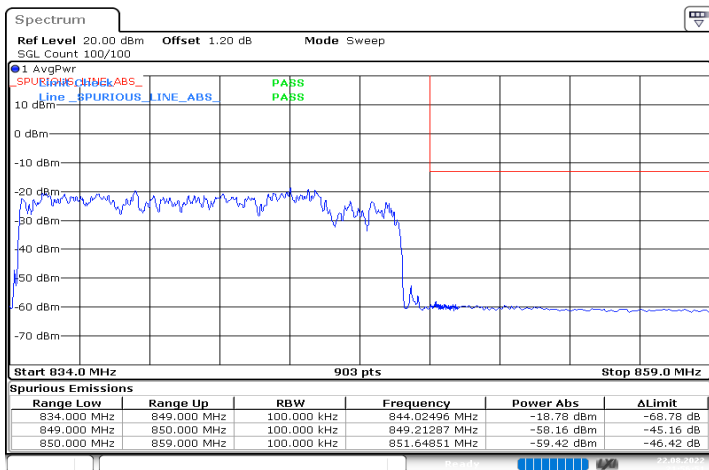
n5_15MHz_15kHz_841.5MHz_DFT-s-OFDM QPSK_RB75@0
