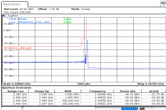
n41_20MHz_30kHz_2506.02MHz_DFT-s-OFDM QPSK_RB1@0
