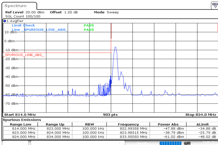
n5_10MHz_15kHz_829MHz_DFT-s-OFDM QPSK_RB1@0
