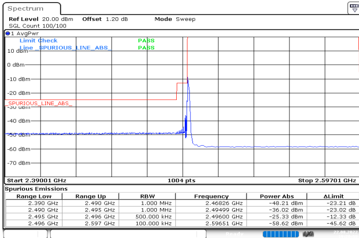
n41_10MHz_30kHz_2501.01MHz_DFT-s-OFDM QPSK_RB1@0
