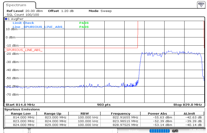
n5_5MHz_15kHz_826.5MHz_DFT-s-OFDM QPSK_RB25@0
