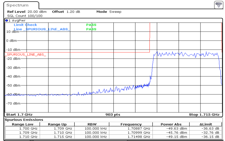
n66_5MHz_15kHz_1712.5MHz_DFT-s-OFDM QPSK_RB25@0
