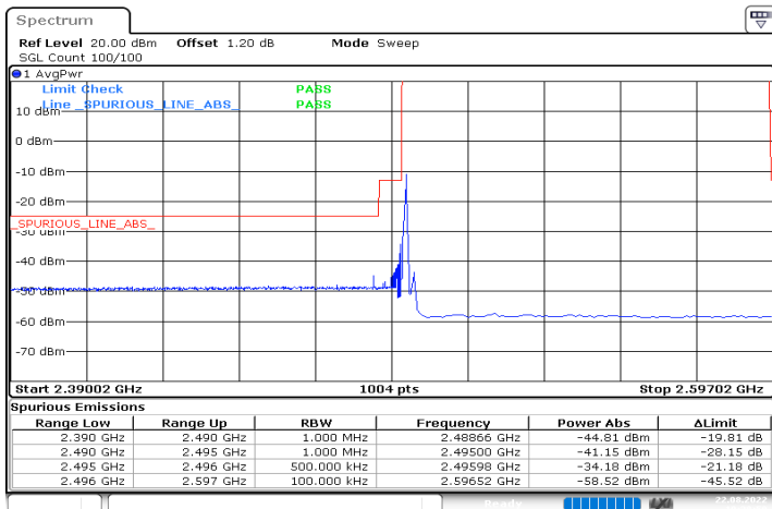
n41_50MHz_30kHz_2521.02MHz_DFT-s-OFDM QPSK_RB1@0
