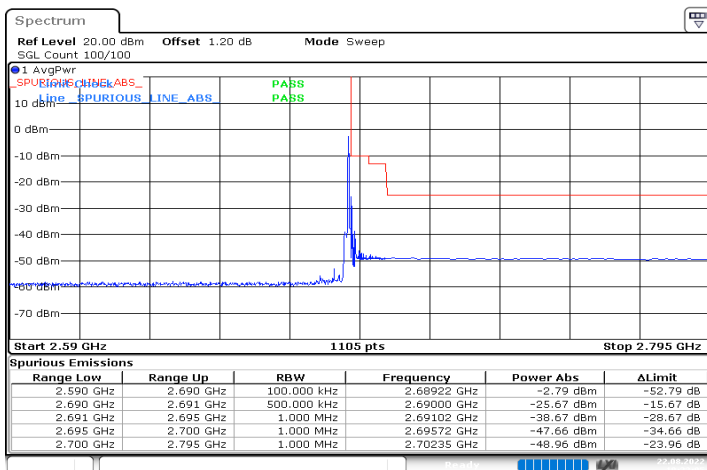
n41_10MHz_30kHz_2685MHz_DFT-s-OFDM QPSK_RB1@23
