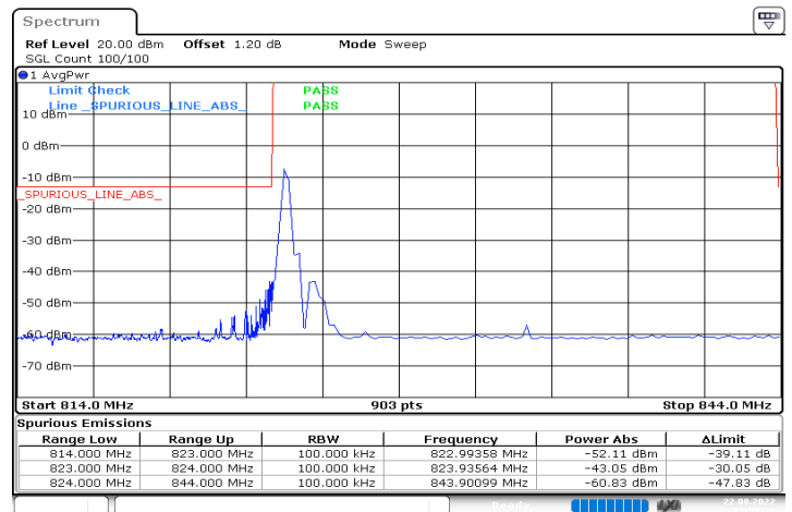
n5_20MHz_15kHz_834MHz_DFT-s-OFDM QPSK_RB1@0
