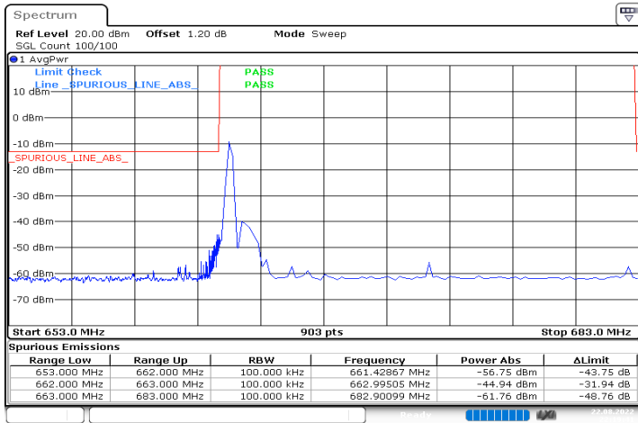
n71_20MHz_15kHz_673MHz_DFT-s-OFDM QPSK_RB1@0
