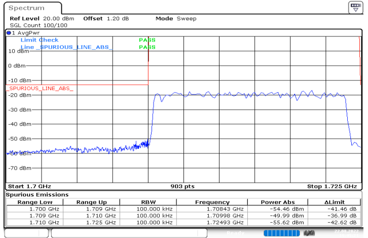
n66_15MHz_15kHz_1717.5MHz_DFT-s-OFDM QPSK_RB75@0
