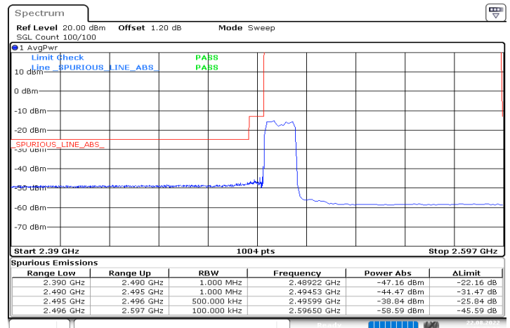
n41_15MHz_30kHz_2503.5MHz_DFT-s-OFDM QPSK_RB36@0
