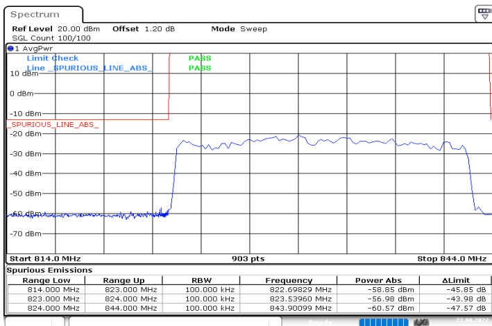
n5_20MHz_15kHz_834MHz_DFT-s-OFDM QPSK_RB100@0
