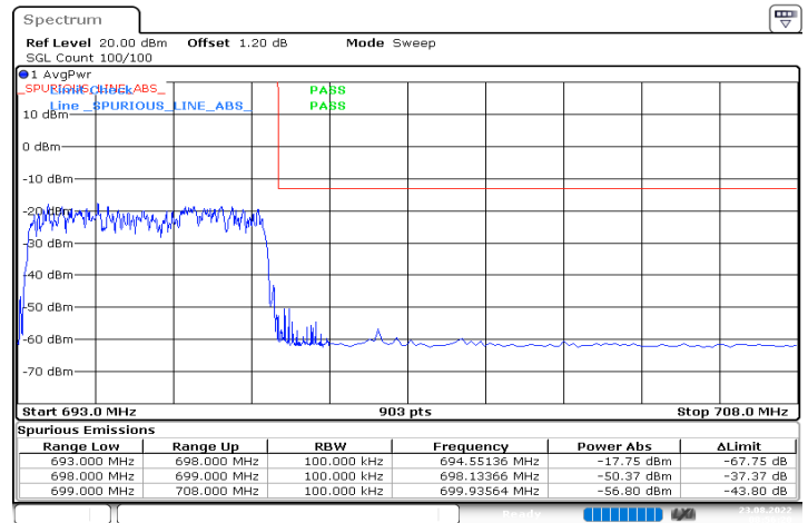
n71_5MHz_15kHz_695.5MHz_DFT-s-OFDM QPSK_RB25@0
