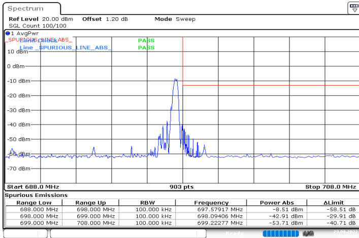
n71_10MHz_15kHz_693MHz_DFT-s-OFDM QPSK_RB1@51
