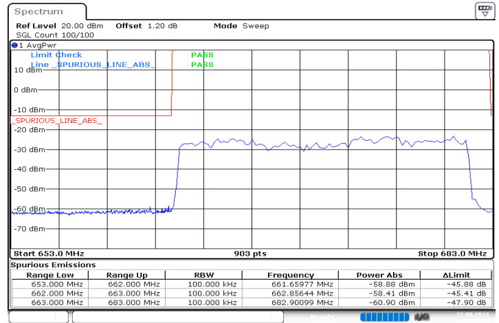
n71_20MHz_15kHz_673MHz_DFT-s-OFDM QPSK_RB100@0
