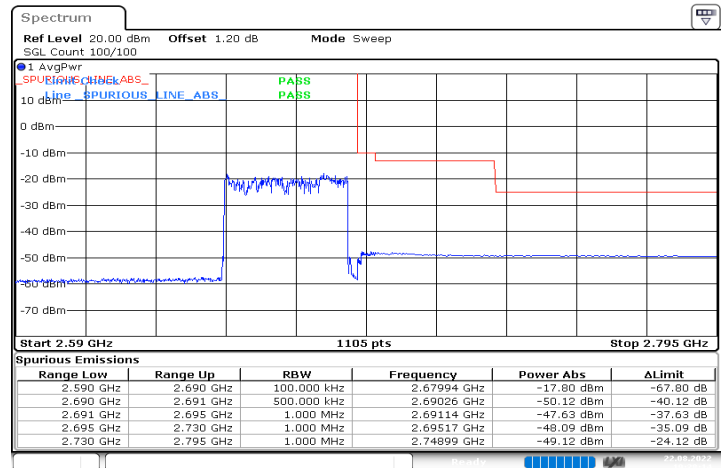
n41_40MHz_30kHz_2670MHz_DFT-s-OFDM QPSK_RB100@0
