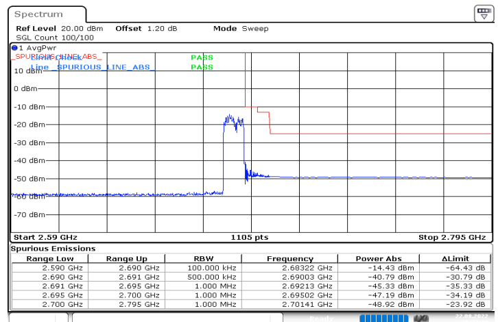
n41_10MHz_30kHz_2685MHz_DFT-s-OFDM QPSK_RB24@0
