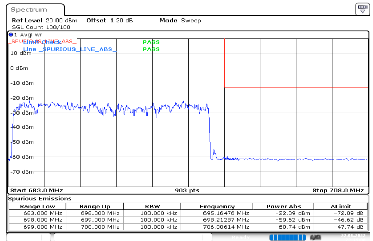
n71_15MHz_15kHz_690.5MHz_DFT-s-OFDM QPSK_RB75@0
