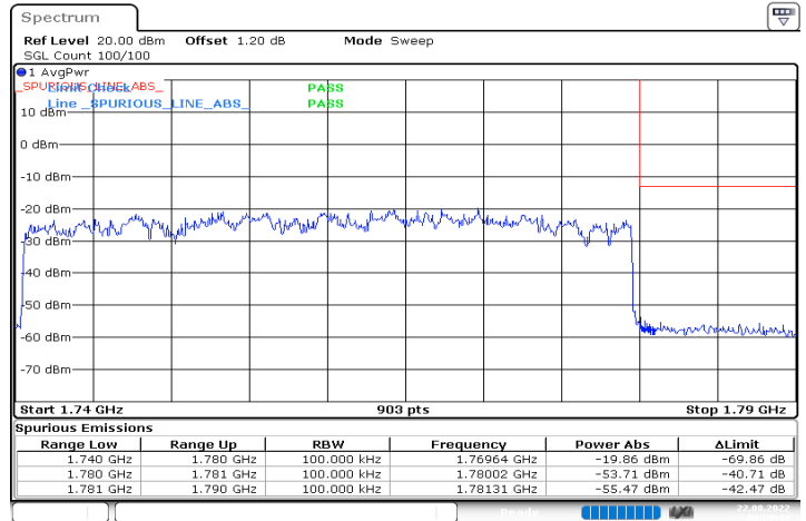
n66_40MHz_15kHz_1760MHz_DFT-s-OFDM QPSK_RB216@0
