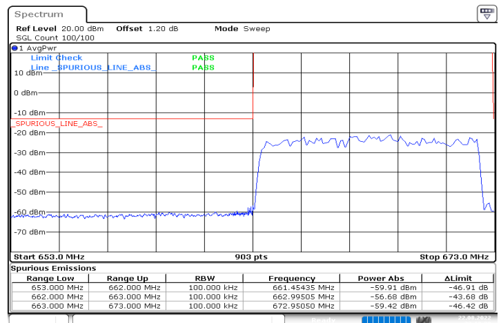
n71_10MHz_15kHz_668MHz_DFT-s-OFDM QPSK_RB50@0
