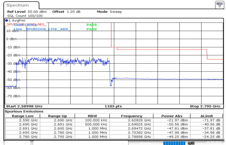
n41_90MHz_30kHz_2644.98MHz_DFT-s-OFDM QPSK_RB243@0
