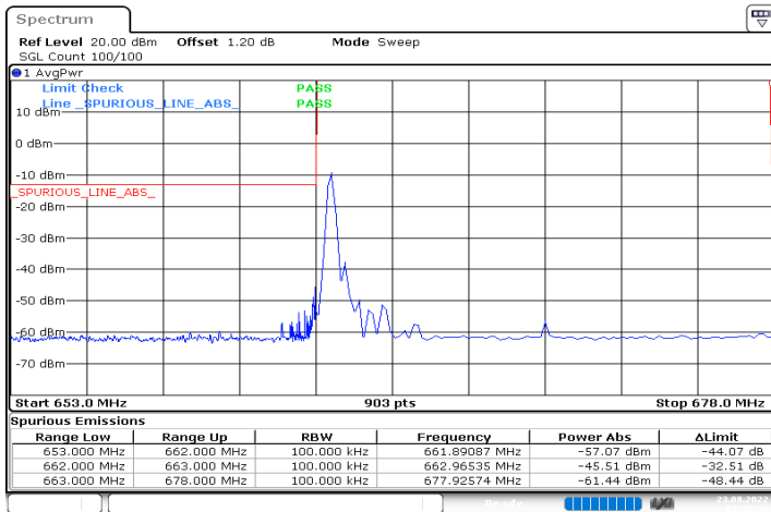
n71_15MHz_15kHz_670.5MHz_DFT-s-OFDM QPSK_RB1@0
