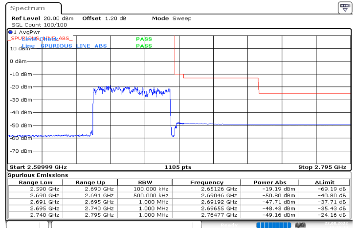
n41_50MHz_30kHz_2664.99MHz_DFT-s-OFDM QPSK_RB128@0
