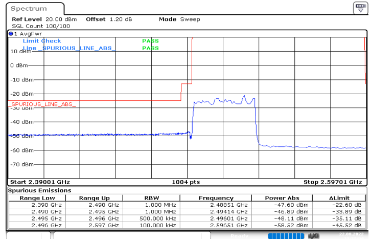
n41_40MHz_30kHz_2516.01MHz_DFT-s-OFDM QPSK_RB100@0
