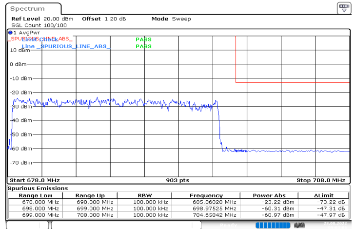
n71_20MHz_15kHz_688MHz_DFT-s-OFDM QPSK_RB100@0
