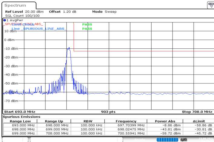
n71_5MHz_15kHz_695.5MHz_DFT-s-OFDM QPSK_RB1@24
