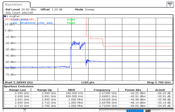
n41_20MHz_30kHz_2679.99MHz_DFT-s-OFDM QPSK_RB50@0
