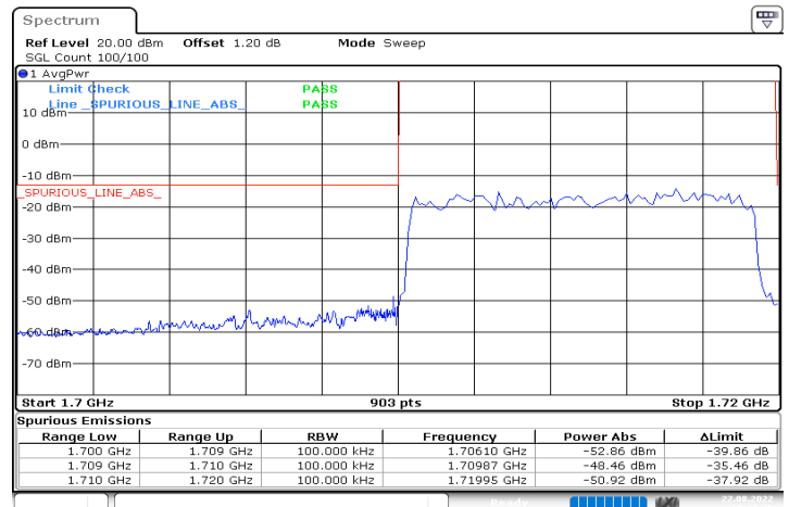
n66_10MHz_15kHz_1715MHz_DFT-s-OFDM QPSK_RB50@0
