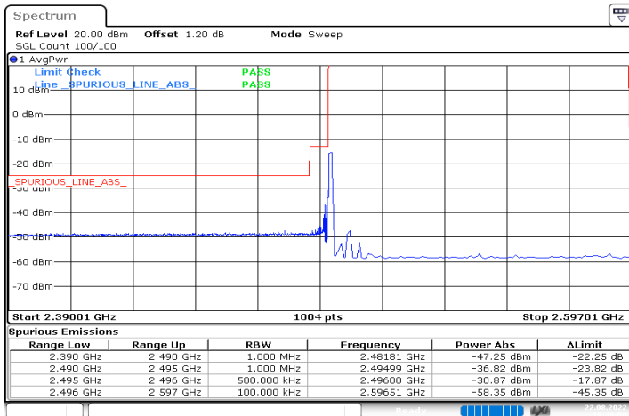
n41_100MHz_30kHz_2546.01MHz_DFT-s-OFDM QPSK_RB1@0
