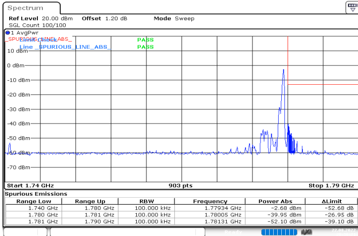
n66_40MHz_15kHz_1760MHz_DFT-s-OFDM QPSK_RB1@215
