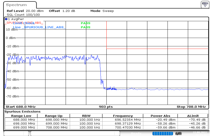
n71_10MHz_15kHz_693MHz_DFT-s-OFDM QPSK_RB50@0
