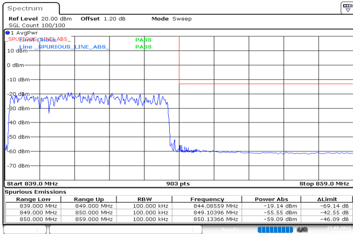
n5_10MHz_15kHz_844MHz_DFT-s-OFDM QPSK_RB50@0
