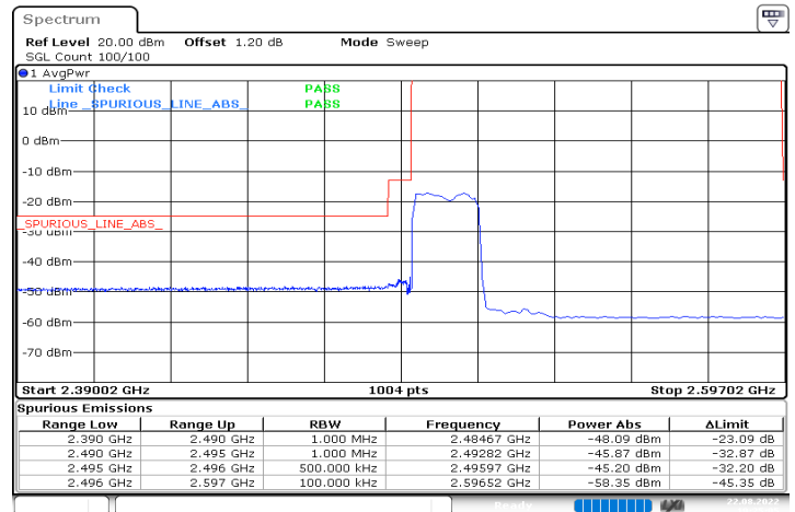
n41_20MHz_30kHz_2506.02MHz_DFT-s-OFDM QPSK_RB50@0
