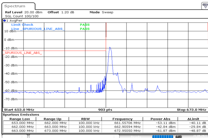
n71_10MHz_15kHz_668MHz_DFT-s-OFDM QPSK_RB1@0
