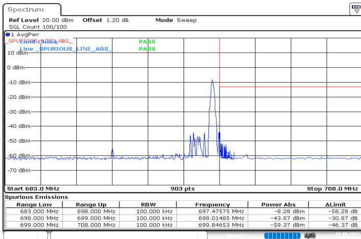
n71_15MHz_15kHz_690.5MHz_DFT-s-OFDM QPSK_RB1@78
