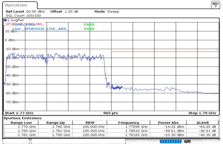
n66_10MHz_15kHz_1775MHz_DFT-s-OFDM QPSK_RB50@0
