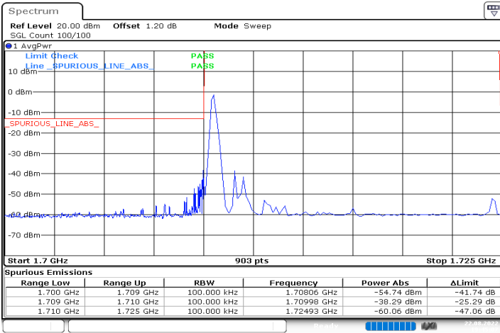
n66_15MHz_15kHz_1717.5MHz_DFT-s-OFDM QPSK_RB1@0
