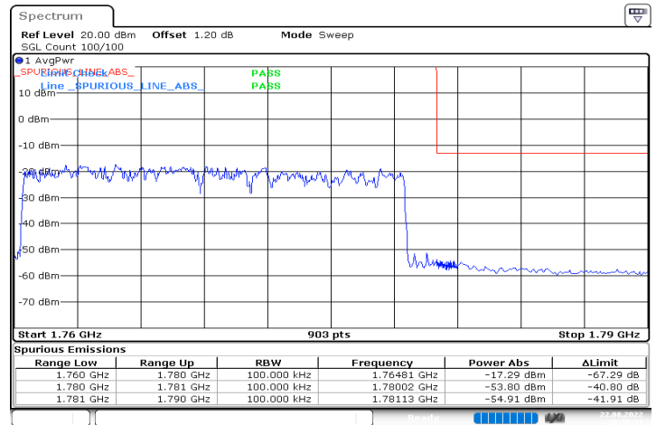
n66_20MHz_15kHz_1770MHz_DFT-s-OFDM QPSK_RB100@0
