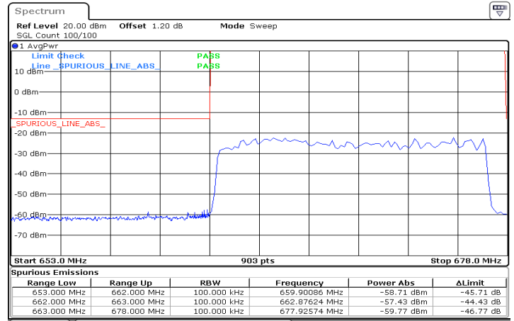
n71_15MHz_15kHz_670.5MHz_DFT-s-OFDM QPSK_RB75@0
