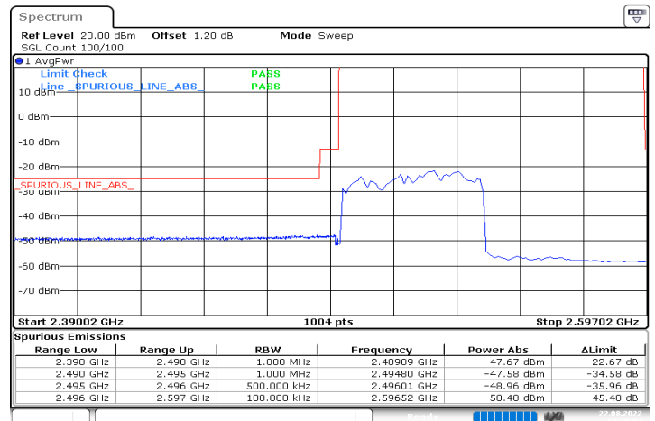
n41_50MHz_30kHz_2521.02MHz_DFT-s-OFDM QPSK_RB128@0
