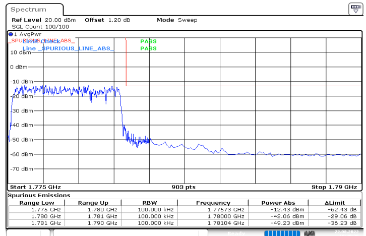
n66_5MHz_15kHz_1777.5MHz_DFT-s-OFDM QPSK_RB25@0
