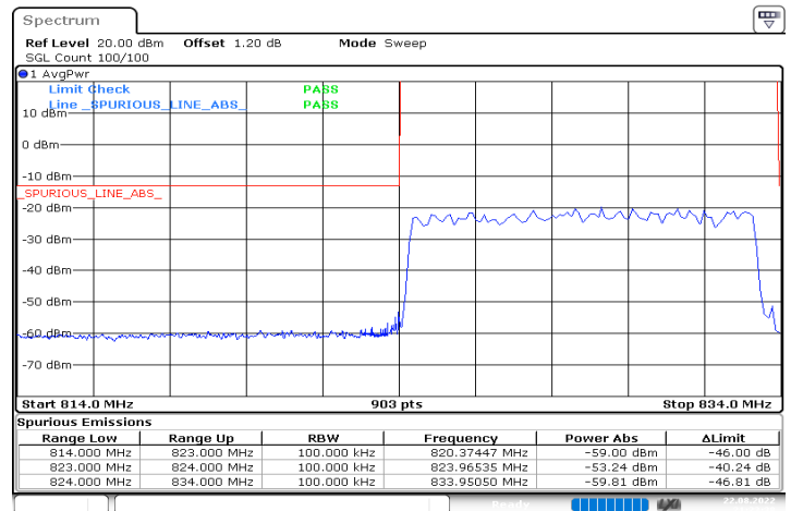
n5_10MHz_15kHz_829MHz_DFT-s-OFDM QPSK_RB50@0
