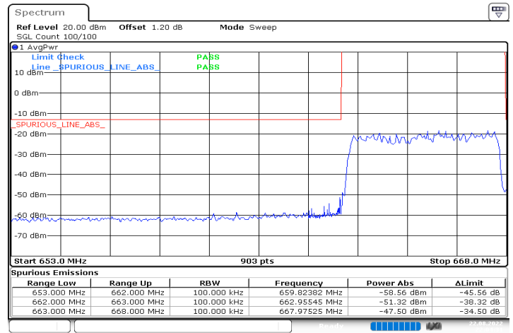
n71_5MHz_15kHz_665.5MHz_DFT-s-OFDM QPSK_RB25@0
