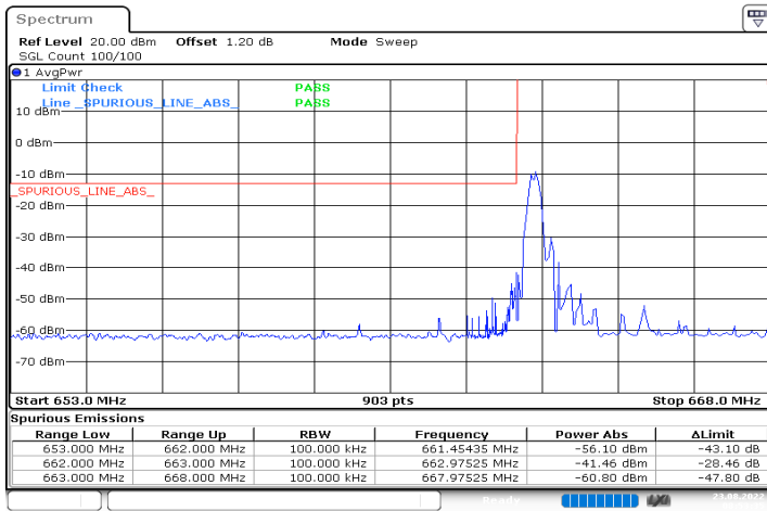
n71_5MHz_15kHz_665.5MHz_DFT-s-OFDM QPSK_RB1@0
