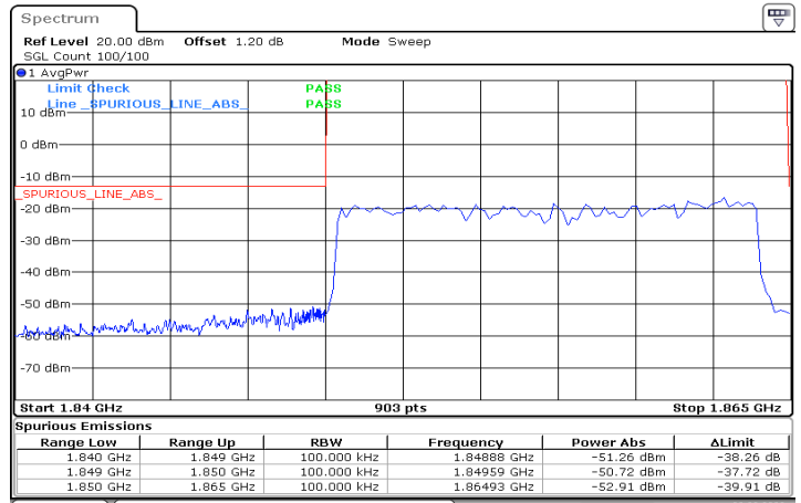
n2_15MHz_15kHz_1857.5MHz_DFT-s-OFDM QPSK_RB75@0
