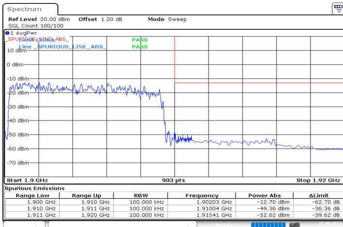
n2_10MHz_15kHz_1905MHz_DFT-s-OFDM QPSK_RB50@0
