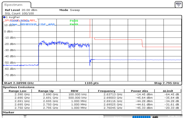
DC_66A_n41A_10MHz|60MHz_30kHz_1745MHz|2659.98MHz_DFT-s-OFDM QPSK_RB0|RB162@0
