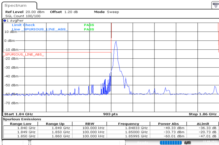
n2_10MHz_15kHz_1855MHz_DFT-s-OFDM QPSK_RB1@0
