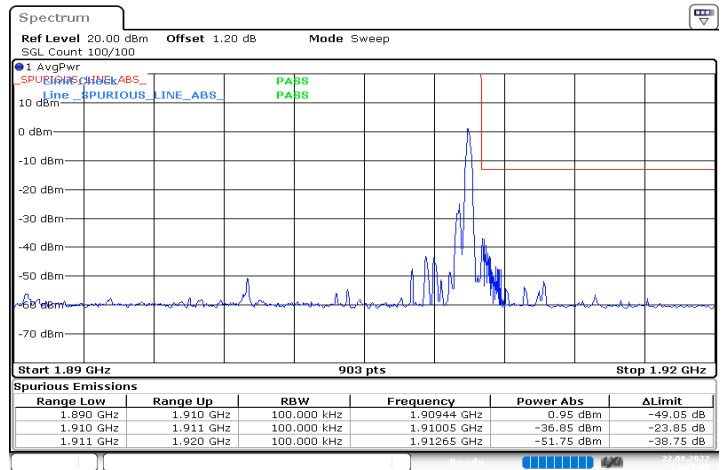
n2_20MHz_15kHz_1900MHz_DFT-s-OFDM QPSK_RB1@105
