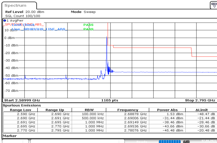
DC_2A_n41A_10MHz|80MHz_30kHz_1880MHz|2649.99MHz_DFT-s-OFDM QPSK_RB0|RB1@216
