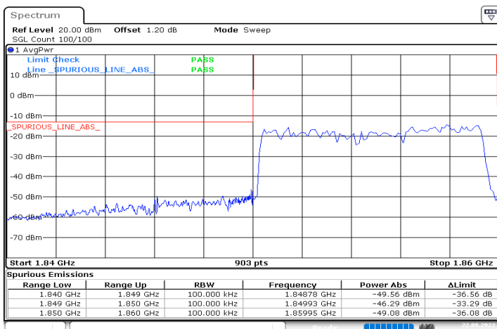
n25_10MHz_15kHz_1855MHz_DFT-s-OFDM QPSK_RB50@0
