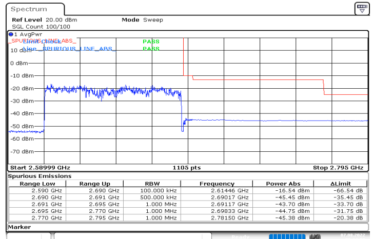
DC_2A_n41A_10MHz|80MHz_30kHz_1880MHz|2649.99MHz_DFT-s-OFDM QPSK_RB0|RB216@0
