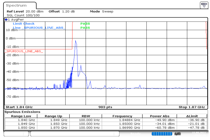
n2_20MHz_15kHz_1860MHz_DFT-s-OFDM QPSK_RB1@0
