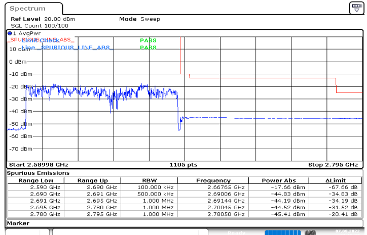
DC_2A_n41A_10MHz|90MHz_30kHz_1880MHz|2644.98MHz_DFT-s-OFDM QPSK_RB0|RB243@0
