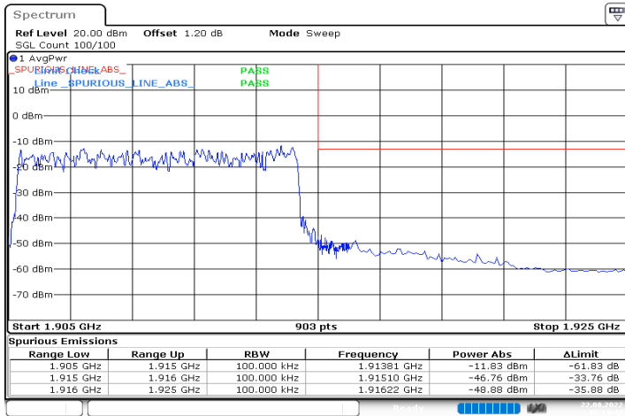
n25_10MHz_15kHz_1910MHz_DFT-s-OFDM QPSK_RB50@0
