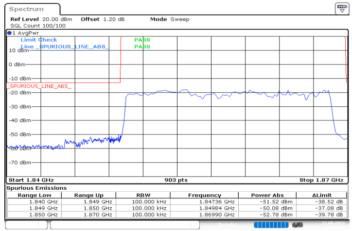
n2_20MHz_15kHz_1860MHz_DFT-s-OFDM QPSK_RB100@0
