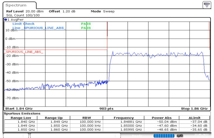
n2_10MHz_15kHz_1855MHz_DFT-s-OFDM QPSK_RB50@0
