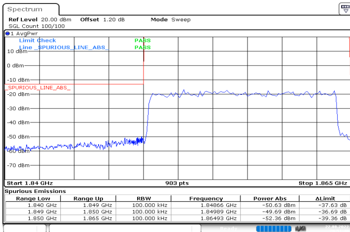
n2_15MHz_15kHz_1857.5MHz_DFT-s-OFDM QPSK_RB75@0
