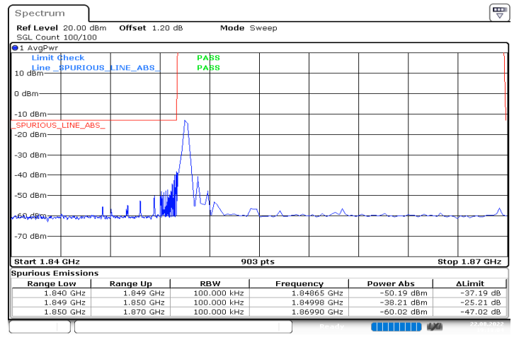
n25_20MHz_15kHz_1860MHz_DFT-s-OFDM QPSK_RB1@0
