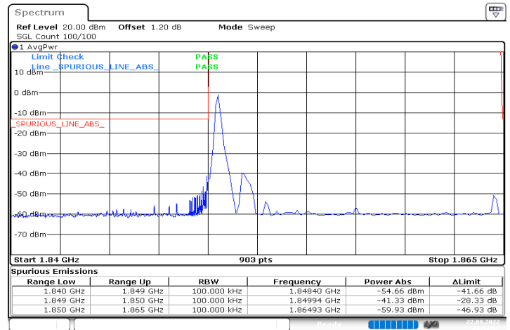
n2_15MHz_15kHz_1857.5MHz_DFT-s-OFDM QPSK_RB1@0
