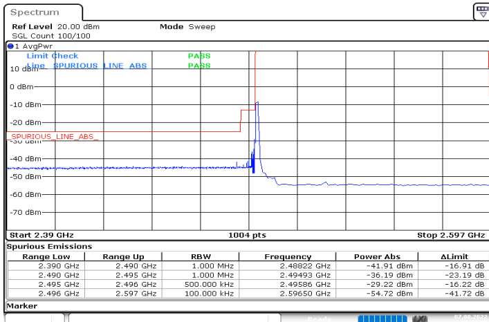
DC_66A_n41A_10MHz|60MHz_30kHz_1745MHz|2526MHz_DFT-s-OFDM QPSK_RB0|RB1@0
