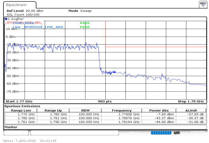
DC_12A_n66A_10MHz|10MHz_15kHz_707.5MHz|1775MHz_DFT-s-OFDM QPSK_RB0|RB50@0
