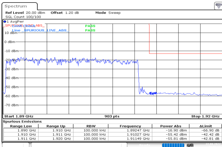
n2_20MHz_15kHz_1900MHz_DFT-s-OFDM QPSK_RB100@0
