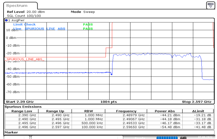
DC_2A_n41A_10MHz|90MHz_30kHz_1880MHz|2541MHz_DFT-s-OFDM QPSK_RB0|RB243@0
