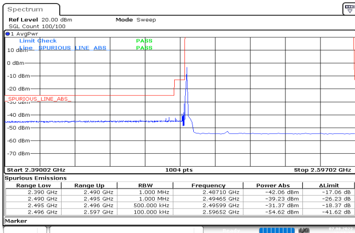
DC_2A_n41A_10MHz|50MHz_30kHz_1880MHz|2521.02MHz_DFT-s-OFDM QPSK_RB0|RB1@0
