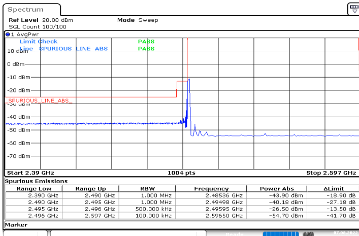
DC_2A_n41A_10MHz|90MHz_30kHz_1880MHz|2541MHz_DFT-s-OFDM QPSK_RB0|RB1@0
