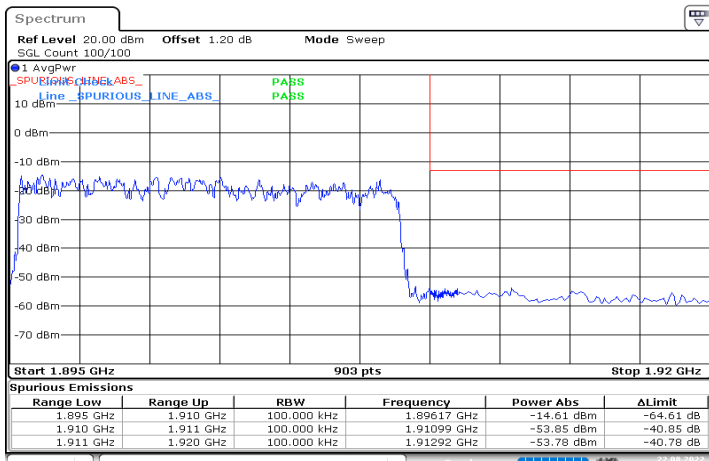
n2_15MHz_15kHz_1902.5MHz_DFT-s-OFDM QPSK_RB75@0
