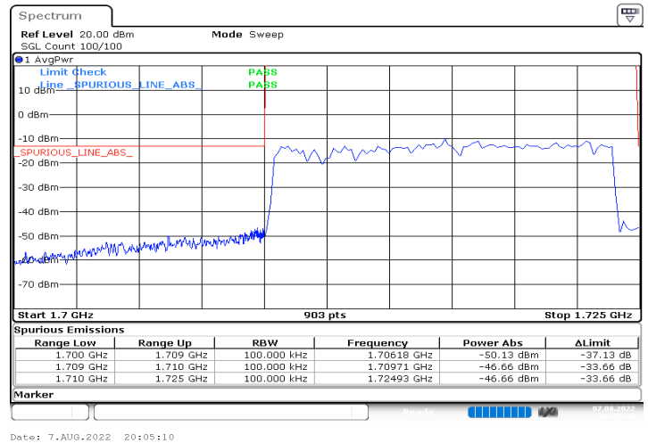
DC_12A_n66A_10MHz|15MHz_15kHz_707.5MHz|1717.5MHz_DFT-s-OFDM QPSK_RB0|RB75@0
