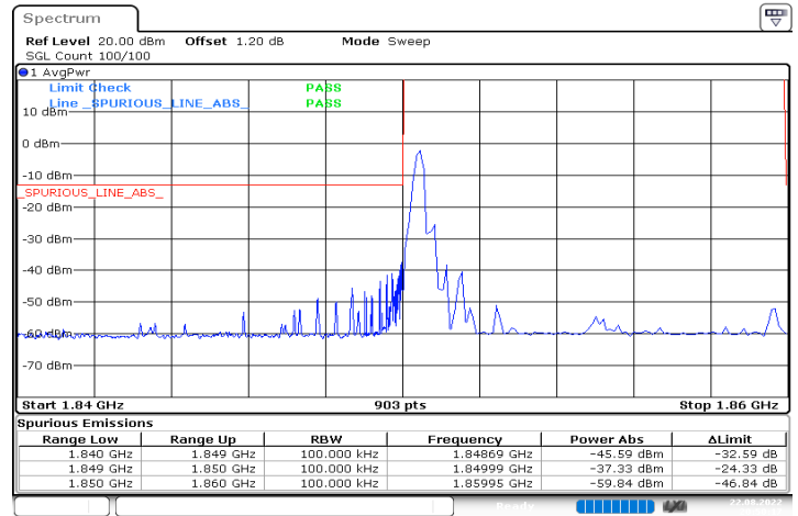
n2_10MHz_15kHz_1855MHz_DFT-s-OFDM QPSK_RB1@0
