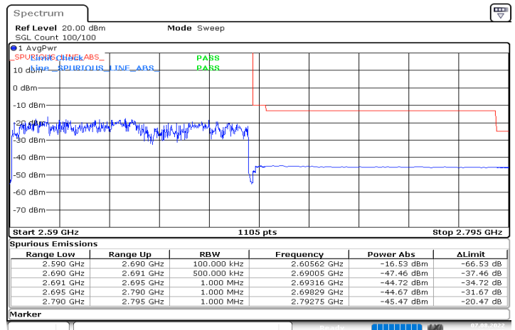
DC_2A_n41A_10MHz|100MHz_30kHz_1880MHz|2640MHz_DFT-s-OFDM QPSK_RB0|RB270@0
