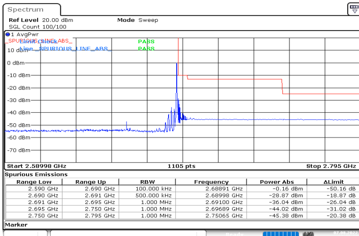
DC_66A_n41A_10MHz|60MHz_30kHz_1745MHz|2659.98MHz_DFT-s-OFDM QPSK_RB0|RB1@161
