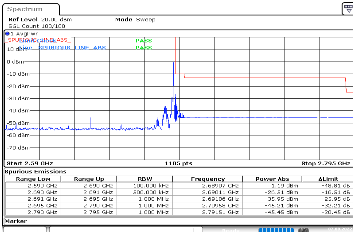
DC_2A_n41A_10MHz|100MHz_30kHz_1880MHz|2640MHz_DFT-s-OFDM QPSK_RB0|RB1@272
