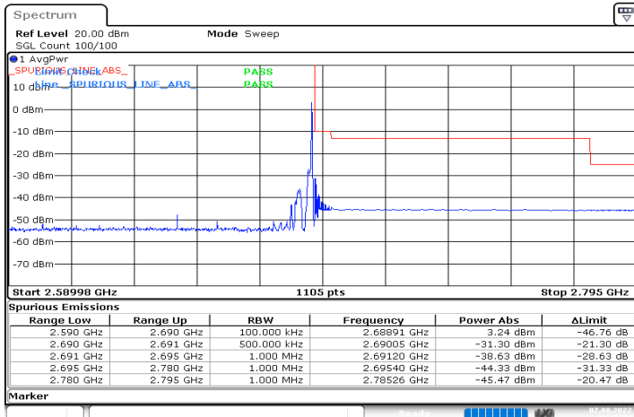
DC_2A_n41A_10MHz|90MHz_30kHz_1880MHz|2644.98MHz_DFT-s-OFDM QPSK_RB0|RB1@244
