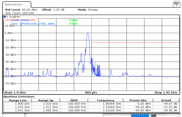
n2_10MHz_15kHz_1905MHz_DFT-s-OFDM QPSK_RB1@51
