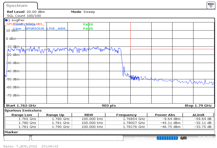
DC_12A_n66A_10MHz|15MHz_15kHz_707.5MHz|1772.5MHz_DFT-s-OFDM QPSK_RB0|RB75@0
