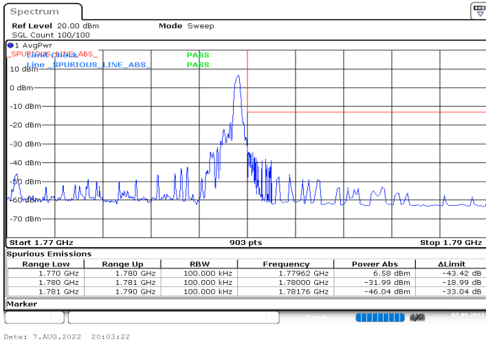
DC_12A_n66A_10MHz|10MHz_15kHz_707.5MHz|1775MHz_DFT-s-OFDM QPSK_RB0|RB1@51
