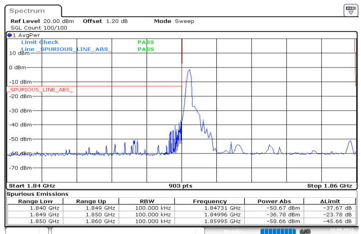
n2_10MHz_15kHz_1855MHz_DFT-s-OFDM QPSK_RB1@0
