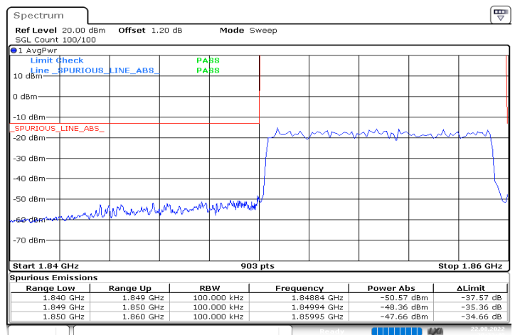
n2_10MHz_15kHz_1855MHz_DFT-s-OFDM QPSK_RB50@0
