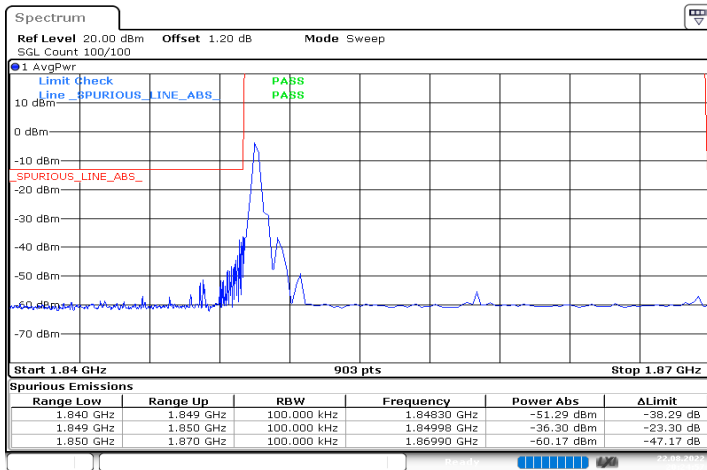
n2_20MHz_15kHz_1860MHz_DFT-s-OFDM QPSK_RB1@0
