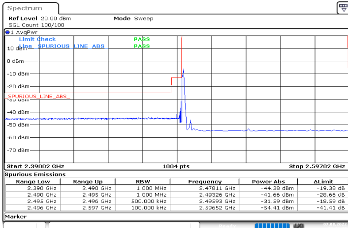
DC_2A_n41A_10MHz|80MHz_30kHz_1880MHz|2536.02MHz_DFT-s-OFDM QPSK_RB0|RB1@0
