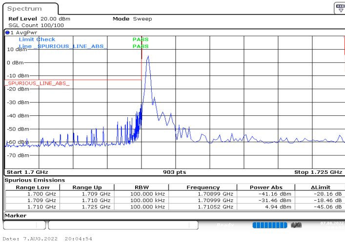
DC_12A_n66A_10MHz|15MHz_15kHz_707.5MHz|1717.5MHz_DFT-s-OFDM QPSK_RB0|RB1@0
