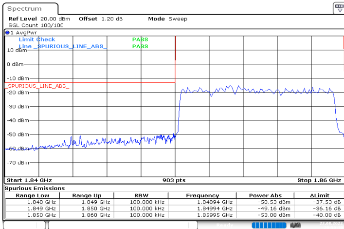
n2_10MHz_15kHz_1855MHz_DFT-s-OFDM QPSK_RB50@0
