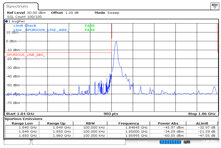
n25_10MHz_15kHz_1855MHz_DFT-s-OFDM QPSK_RB1@0
