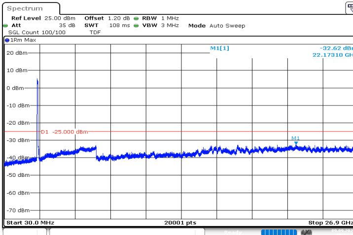
n41_100MHz_30kHz_2546.01MHz_DFT-s-OFDM_QPSK_RB270@0|30MHz_26.9GHz
