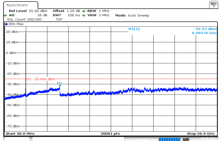
n41_40MHz_30kHz_2670MHz_DFT-s-OFDM QPSK_RB1@0|30MHz_26.9GHz
