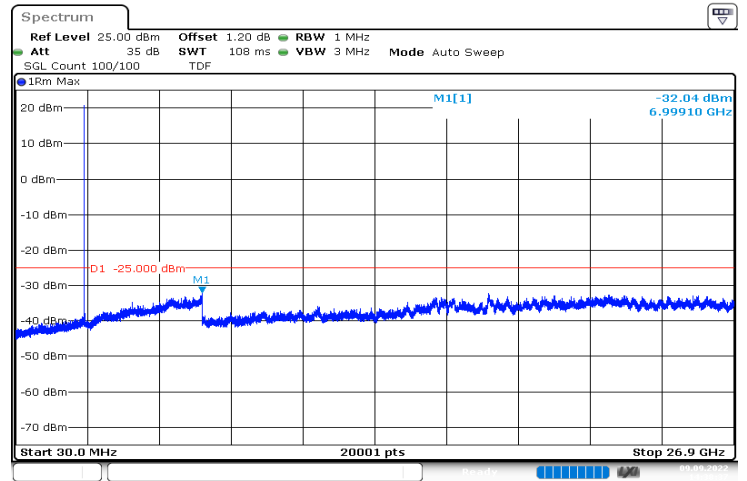
n41_10MHz_30kHz_2592.99MHz_DFT-s-OFDM QPSK_RB1@0|30MHz_26.9GHz
