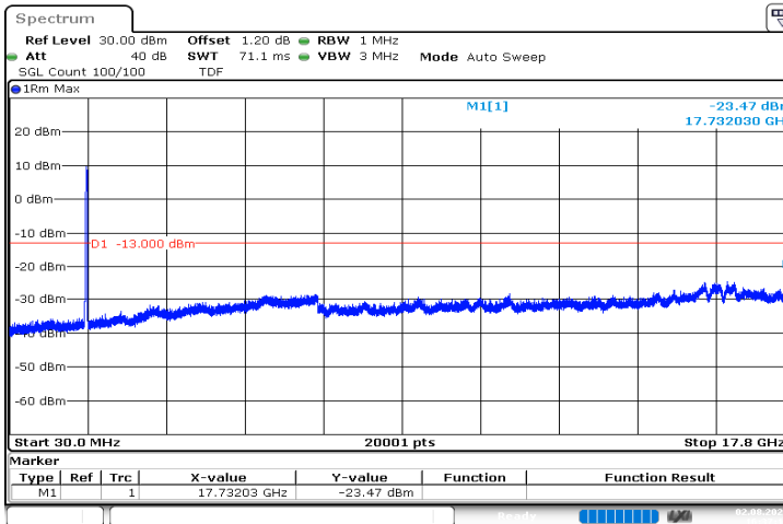
n66_30MHz_15kHz_1765MHz_DFT-s-OFDM QPSK_RB160@0|30MHz_17.8GHz
