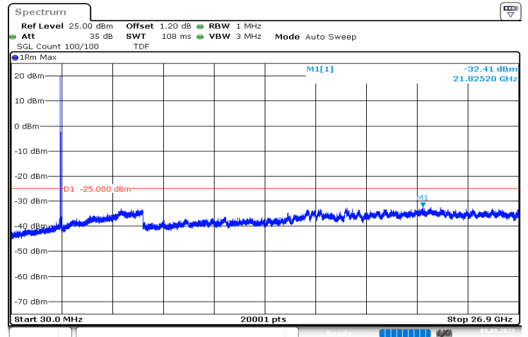
n41_60MHz_30kHz_2659.98MHz_DFT-s-OFDM QPSK_RB1@0|30MHz_26.9GHz
