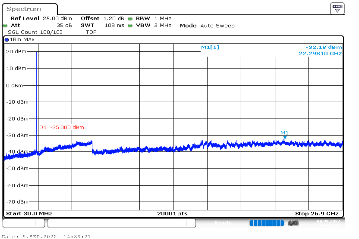
n41_10MHz_30kHz_2592.99MHz_DFT-s-OFDM QPSK_RB1@23|30MHz_26.9GHz
