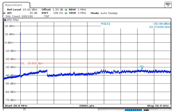
n41_15MHz_30kHz_2682.48MHz_DFT-s-OFDM QPSK_RB36@0|30MHz_26.9GHz
