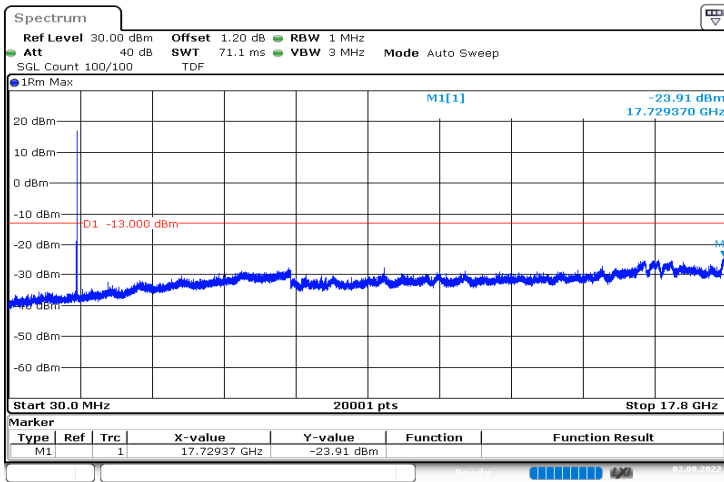
n66_5MHz_15kHz_1712.5MHz_DFT-s-OFDM QPSK_RB25@0|30MHz_17.8GHz
