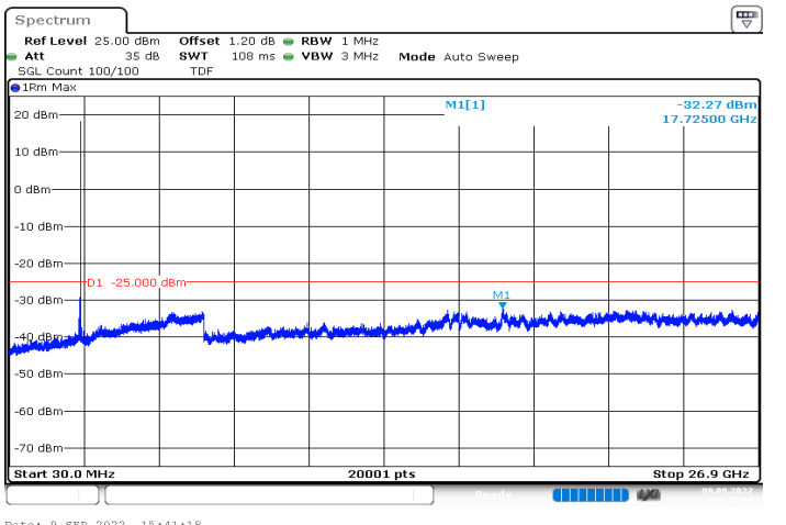
n41_90MHz_30kHz_2541MHz_DFT-s-OFDM QPSK_RB1@244|30MHz_26.9GHz
