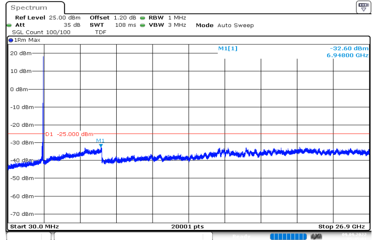
n41_90MHz_30kHz_2592.99MHz_DFT-s-OFDM QPSK_RB1@244|30MHz_26.9GHz
