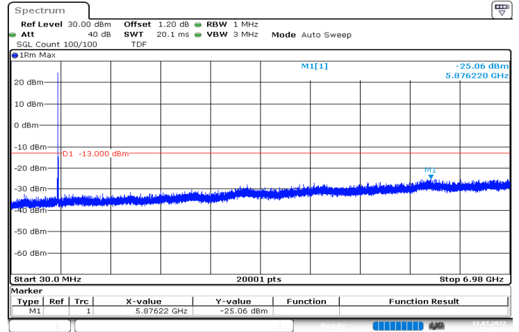
n71_5MHz_15kHz_680.5MHz_DFT-s-OFDM QPSK_RB1@0|30MHz_6.98GHz
