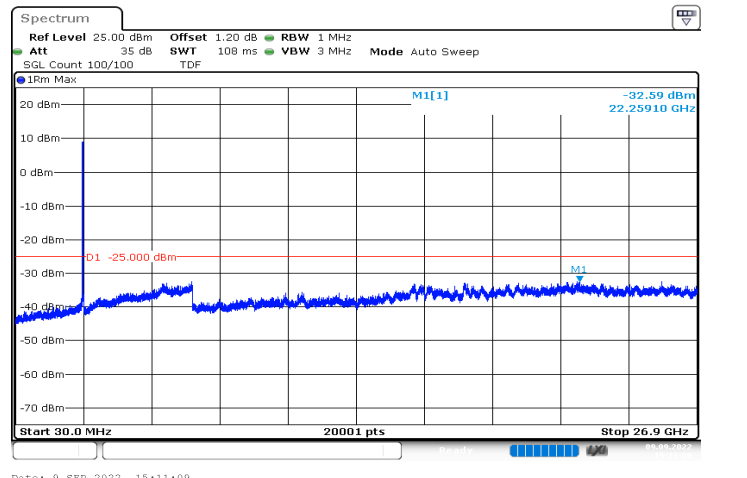
n41_40MHz_30kHz_2670MHz_DFT-s-OFDM QPSK_RB100@0|30MHz_26.9GHz
