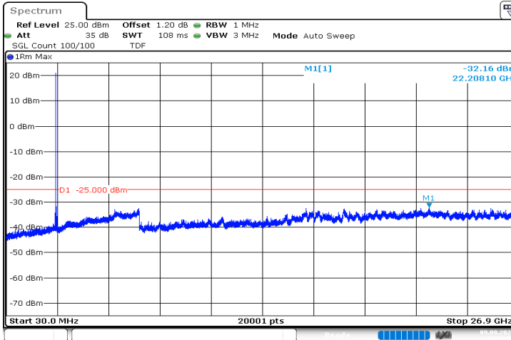
n41_80MHz_30kHz_2649.99MHz_DFT-s-OFDM QPSK_RB1@0|30MHz_26.9GHz
