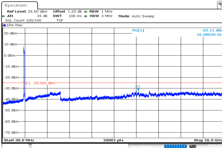
n41_90MHz_30kHz_2592.99MHz_DFT-s-OFDM QPSK_RB243@0|30MHz_26.9GHz
