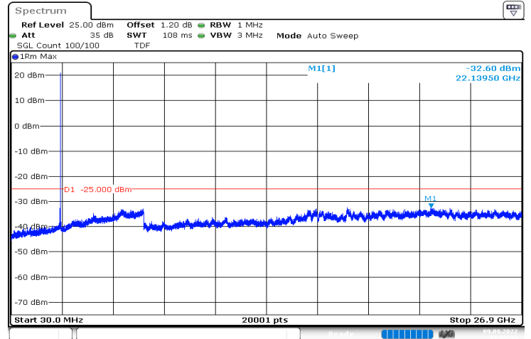
n41_40MHz_30kHz_2592.99MHz_DFT-s-OFDM QPSK_RB1@105|30MHz_26.9GHz
