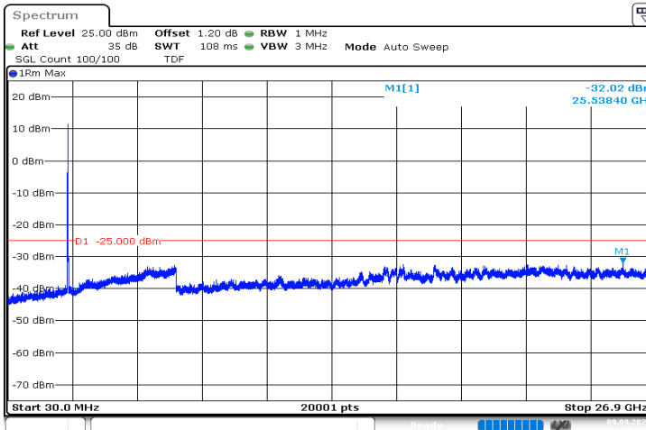
n41_20MHz_30kHz_2506.02MHz_DFT-s-OFDM QPSK_RB50@0|30MHz_26.9GHz
