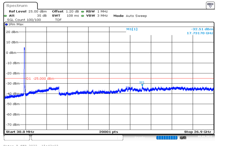
n41_90MHz_30kHz_2541MHz_DFT-s-OFDM QPSK_RB243@0|30MHz_26.9GHz
