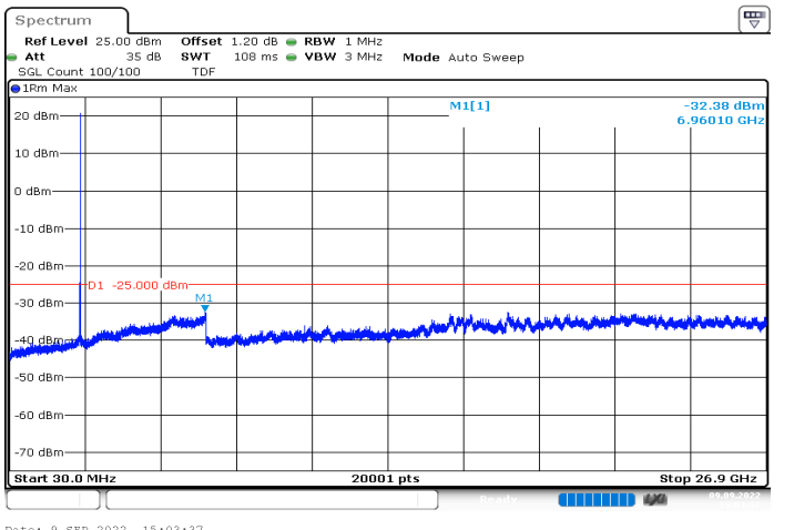
n41_40MHz_30kHz_2516.01MHz_DFT-s-OFDM QPSK_RB1@105|30MHz_26.9GHz
