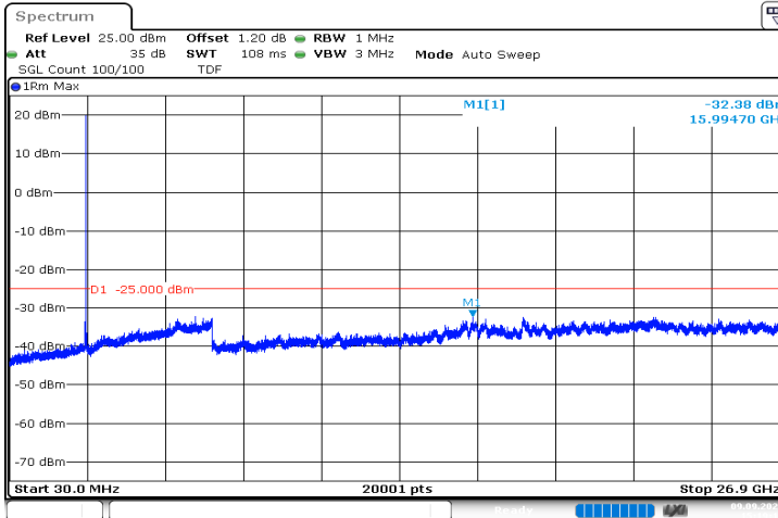
n41_50MHz_30kHz_2664.99MHz_DFT-s-OFDM QPSK_RB1@0|30MHz_26.9GHz
