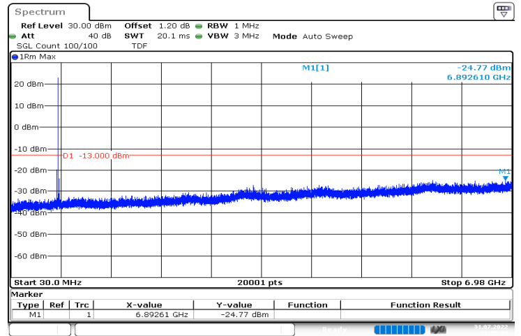
n71_20MHz_15kHz_688MHz_DFT-s-OFDM QPSK_RB1@0|30MHz_6.98GHz
