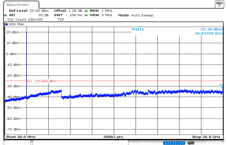
n41_10MHz_30kHz_2685MHz_DFT-s-OFDM QPSK_RB1@23|30MHz_26.9GHz
