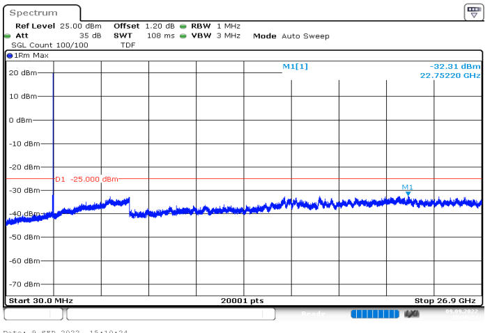
n41_40MHz_30kHz_2670MHz_DFT-s-OFDM QPSK_RB1@105|30MHz_26.9GHz
