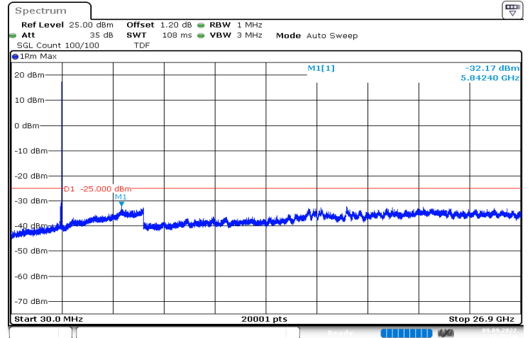
n41_80MHz_30kHz_2649.99MHz_DFT-s-OFDM QPSK_RB1@216|30MHz_26.9GHz
