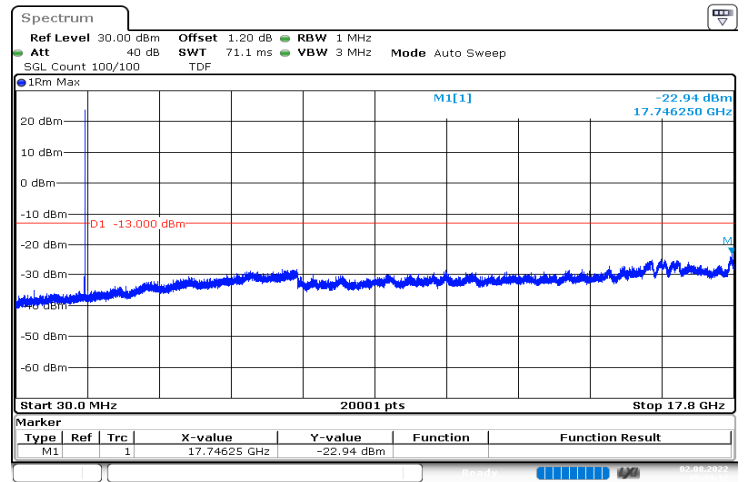
n66_5MHz_15kHz_1745MHz_DFT-s-OFDM QPSK_RB1@24|30MHz_17.8GHz
