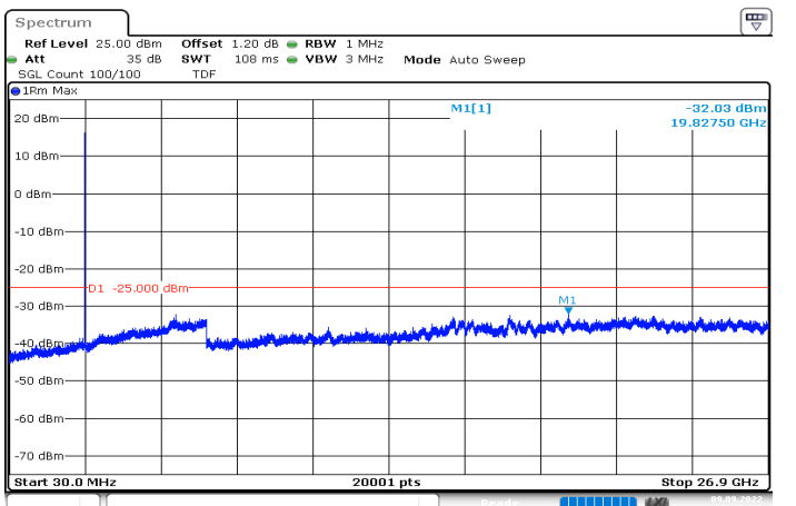
n41_15MHz_30kHz_2682.48MHz_DFT-s-OFDM QPSK_RB1@37|30MHz_26.9GHz
