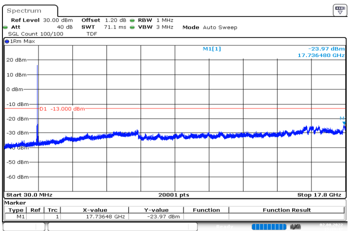
n66_5MHz_15kHz_1745MHz_DFT-s-OFDM QPSK_RB25@0|30MHz_17.8GHz
