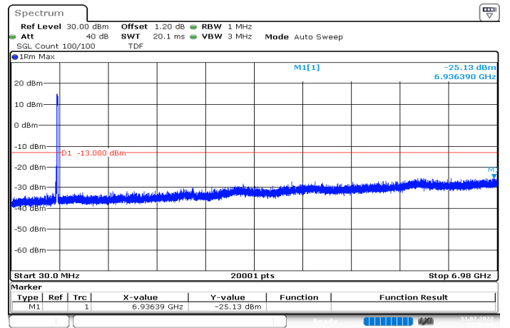
n71_20MHz_15kHz_688MHz_DFT-s-OFDM QPSK_RB100@0|30MHz_6.98GHz
