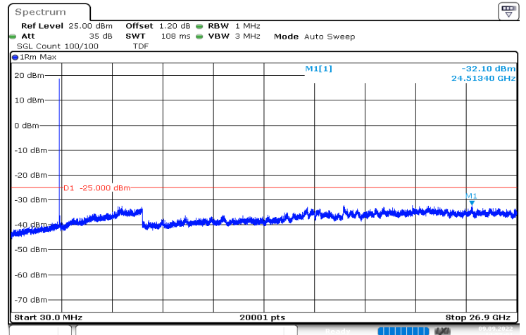
n41_20MHz_30kHz_2592.99MHz_DFT-s-OFDM QPSK_RB1@0|30MHz_26.9GHz
