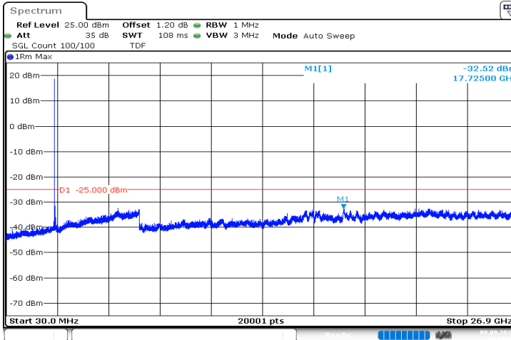
n41_90MHz_30kHz_2592.99MHz_DFT-s-OFDM QPSK_RB1@0|30MHz_26.9GHz
