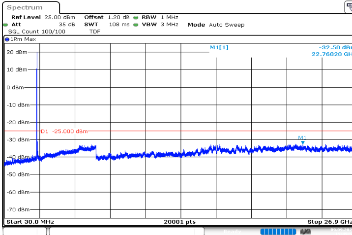
n41_100MHz_30kHz_2546.01MHz_DFT-s-OFDM_QPSK_RB1@0|30MHz_26.9GHz
