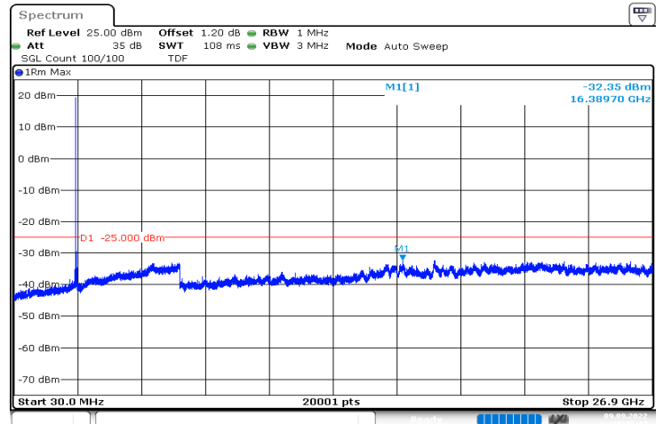
n41_90MHz_30kHz_2644.98MHz_DFT-s-OFDM QPSK_RB1@0|30MHz_26.9GHz
