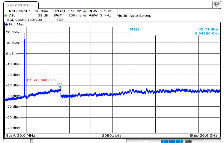
n41_15MHz_30kHz_2503.5MHz_DFT-s-OFDM QPSK_RB1@0|30MHz_26.9GHz
