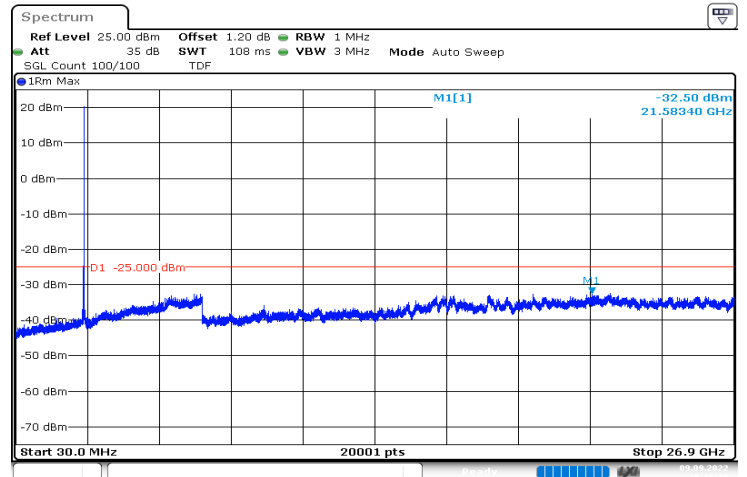
n41_50MHz_30kHz_2592.99MHz_DFT-s-OFDM QPSK_RB1@0|30MHz_26.9GHz
