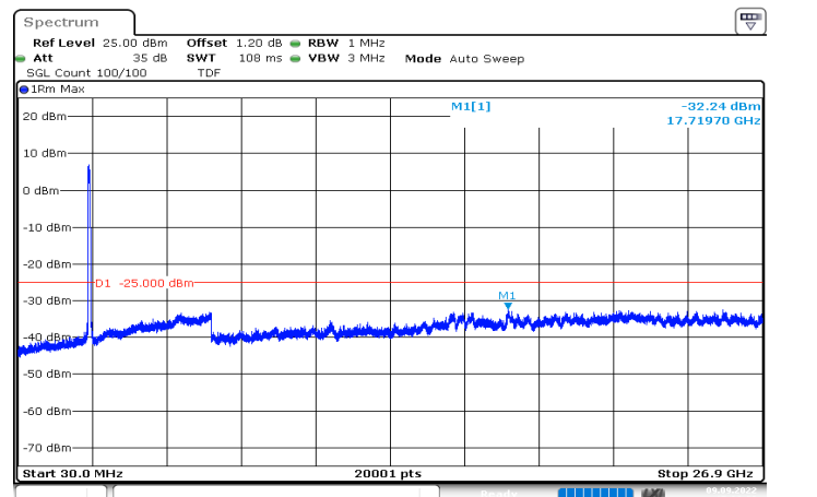
n41_80MHz_30kHz_2592.99MHz_DFT-s-OFDM QPSK_RB216@0|30MHz_26.9GHz
