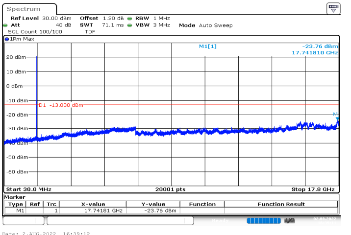
n66_40MHz_15kHz_1730MHz_DFT-s-OFDM QPSK_RB1@215|30MHz_17.8GHz
