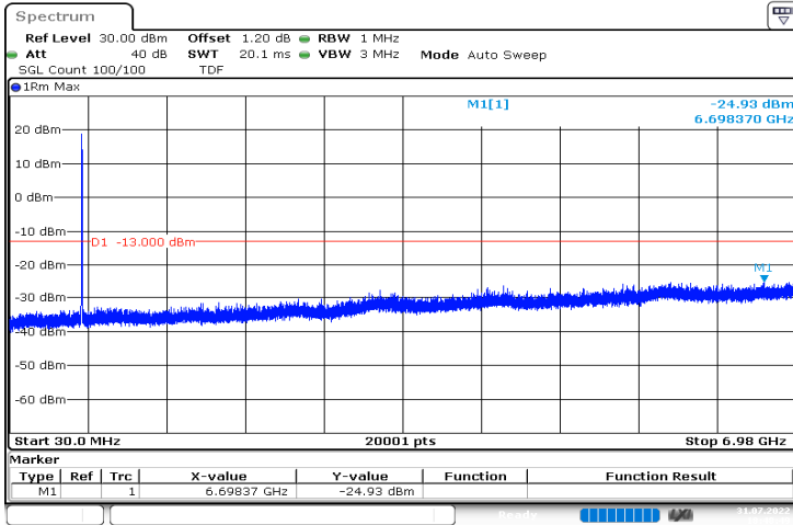
n71_5MHz_15kHz_665.5MHz_DFT-s-OFDM QPSK_RB25@0|30MHz_6.98GHz
