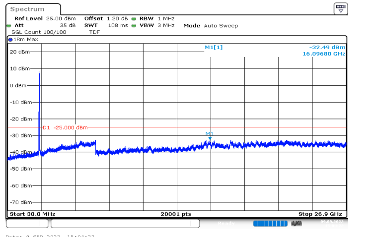
n41_40MHz_30kHz_2516.01MHz_DFT-s-OFDM QPSK_RB100@0|30MHz_26.9GHz
