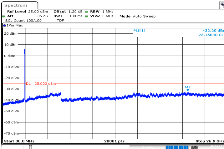
n41_80MHz_30kHz_2649.99MHz_DFT-s-OFDM QPSK_RB216@0|30MHz_26.9GHz
