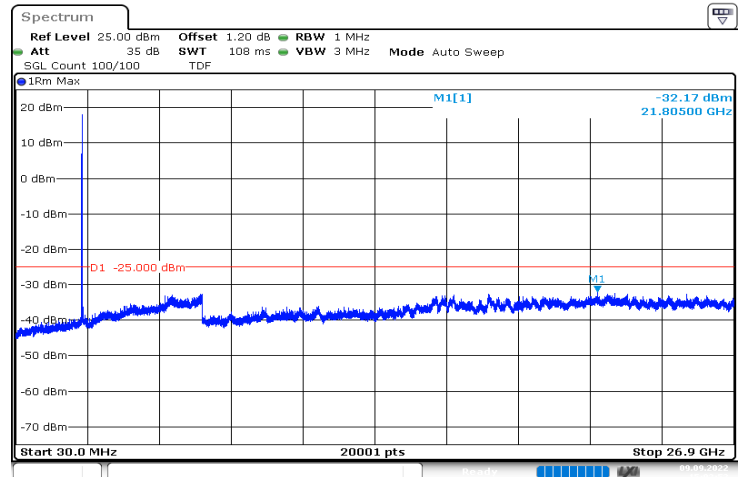
n41_40MHz_30kHz_2516.01MHz_DFT-s-OFDM QPSK_RB1@0|30MHz_26.9GHz
