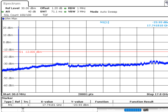
n66_30MHz_15kHz_1765MHz_DFT-s-OFDM QPSK_RB1@0|30MHz_17.8GHz
