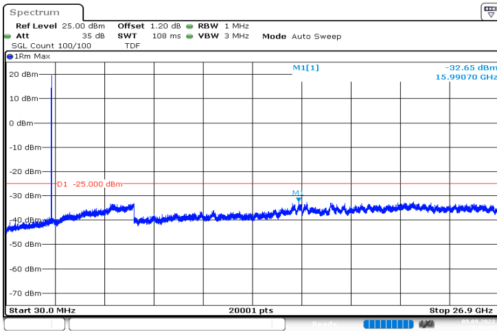
n41_10MHz_30kHz_2501.01MHz_DFT-s-OFDM QPSK_RB1@0|30MHz_26.9GHz
