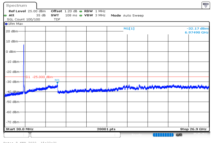
n41_60MHz_30kHz_2526MHz_DFT-s-OFDM QPSK_RB162@0|30MHz_26.9GHz
