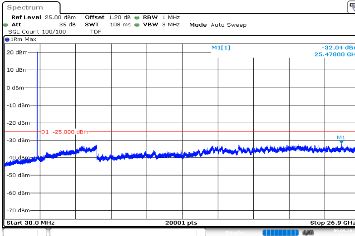
n41_20MHz_30kHz_2506.02MHz_DFT-s-OFDM QPSK_RB1@0|30MHz_26.9GHz
