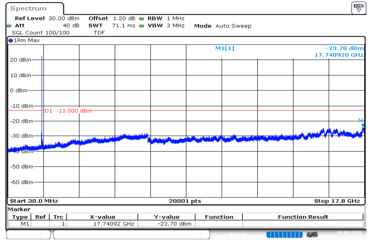
n66_5MHz_15kHz_1712.5MHz_DFT-s-OFDM QPSK_RB1@24|30MHz_17.8GHz
