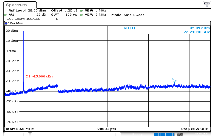
n41_90MHz_30kHz_2541MHz_DFT-s-OFDM QPSK_RB1@0|30MHz_26.9GHz
