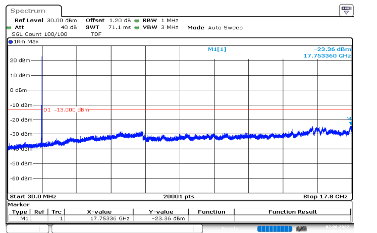
n66_5MHz_15kHz_1777.5MHz_DFT-s-OFDM QPSK_RB1@0|30MHz_17.8GHz
