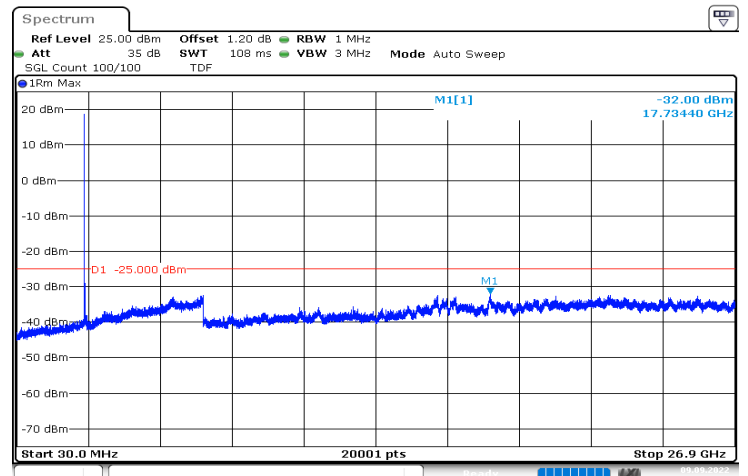
n41_80MHz_30kHz_2592.99MHz_DFT-s-OFDM QPSK_RB1@0|30MHz_26.9GHz
