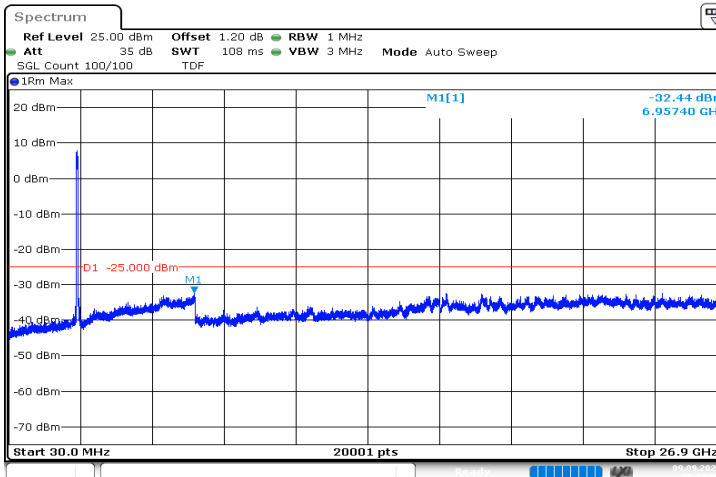
n41_60MHz_30kHz_2592.99MHz_DFT-s-OFDM QPSK_RB162@0|30MHz_26.9GHz
