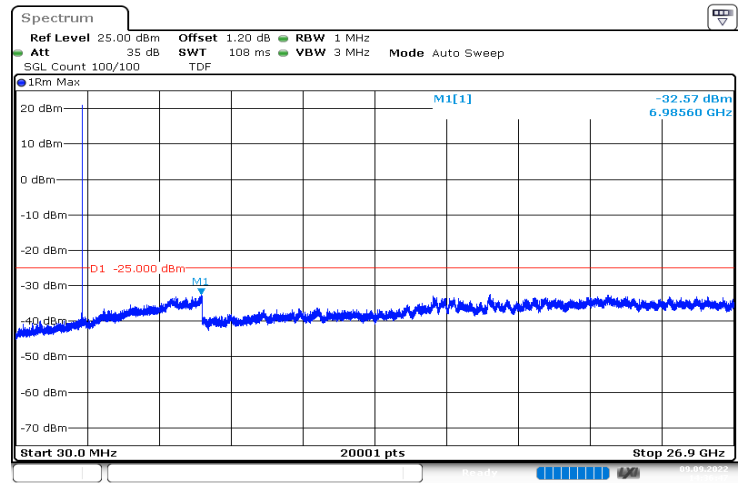
n41_10MHz_30kHz_2501.01MHz_DFT-s-OFDM QPSK_RB1@23|30MHz_26.9GHz
