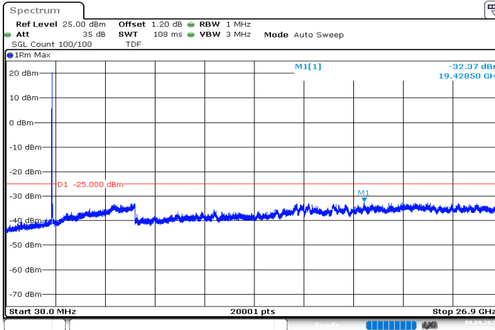
n41_50MHz_30kHz_2521.02MHz_DFT-s-OFDM QPSK_RB1@0|30MHz_26.9GHz
