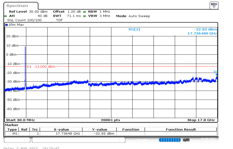
n66_40MHz_15kHz_1730MHz_DFT-s-OFDM QPSK_RB216@0|30MHz_17.8GHz
