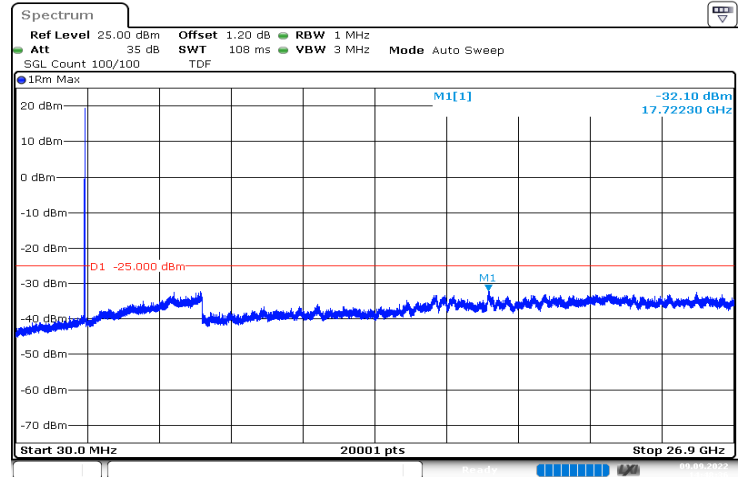
n41_15MHz_30kHz_2592.99MHz_DFT-s-OFDM QPSK_RB1@37|30MHz_26.9GHz
