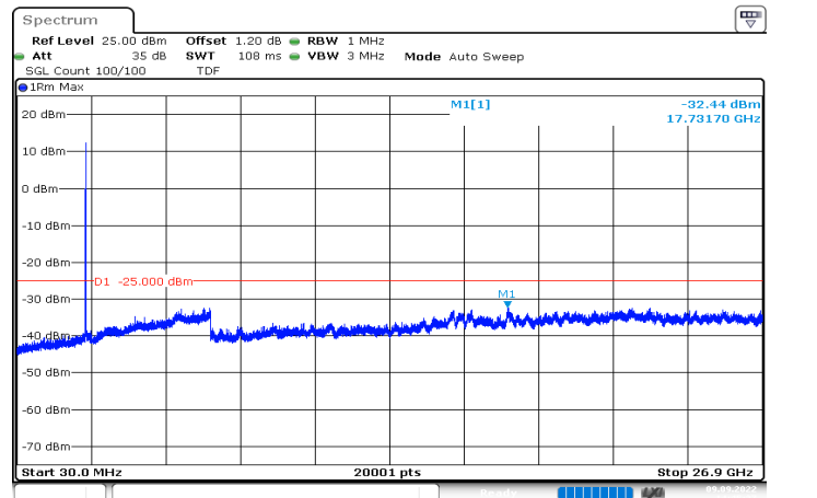
n41_15MHz_30kHz_2503.5MHz_DFT-s-OFDM QPSK_RB36@0|30MHz_26.9GHz
