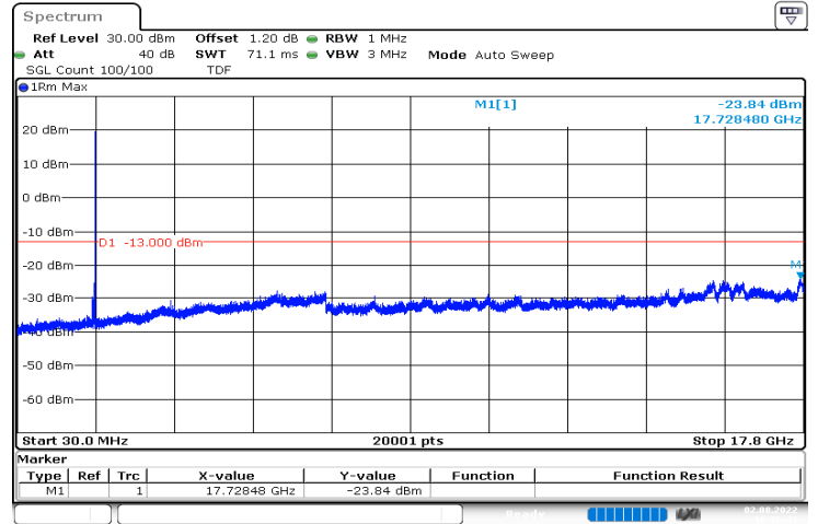
n66_30MHz_15kHz_1765MHz_DFT-s-OFDM QPSK_RB1@159|30MHz_17.8GHz
