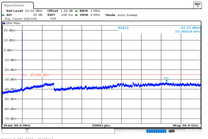
n41_60MHz_30kHz_2659.98MHz_DFT-s-OFDM QPSK_RB1@161|30MHz_26.9GHz
