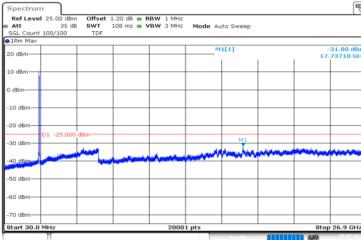
n41_40MHz_30kHz_2592.99MHz_DFT-s-OFDM QPSK_RB100@0|30MHz_26.9GHz
