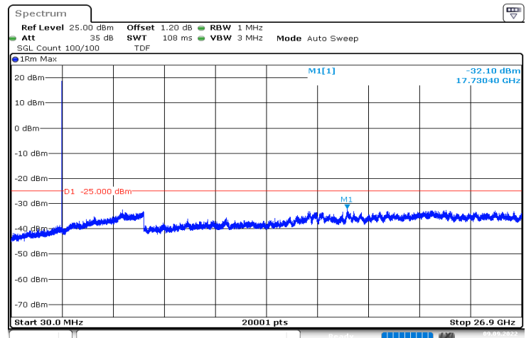
n41_15MHz_30kHz_2682.48MHz_DFT-s-OFDM QPSK_RB1@0|30MHz_26.9GHz
