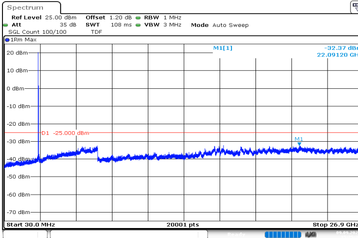
n41_60MHz_30kHz_2592.99MHz_DFT-s-OFDM QPSK_RB1@0|30MHz_26.9GHz
