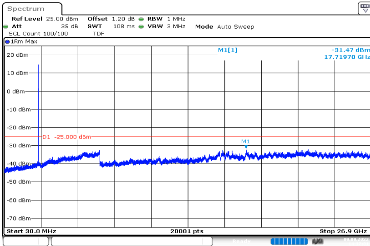
n41_10MHz_30kHz_2501.01MHz_DFT-s-OFDM QPSK_RB24@0|30MHz_26.9GHz
