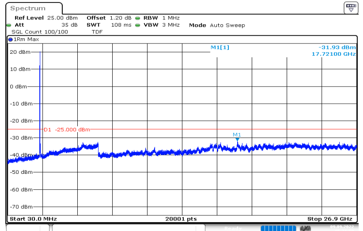
n41_60MHz_30kHz_2526MHz_DFT-s-OFDM QPSK_RB1@0|30MHz_26.9GHz
