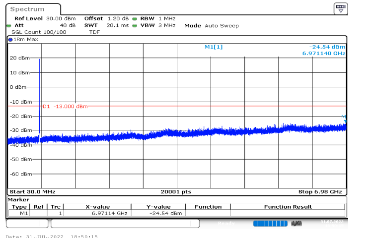
n71_5MHz_15kHz_680.5MHz_DFT-s-OFDM QPSK_RB25@0|30MHz_6.98GHz
