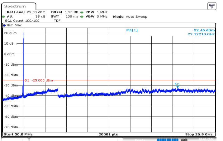
n41_80MHz_30kHz_2592.99MHz_DFT-s-OFDM QPSK_RB1@216|30MHz_26.9GHz
