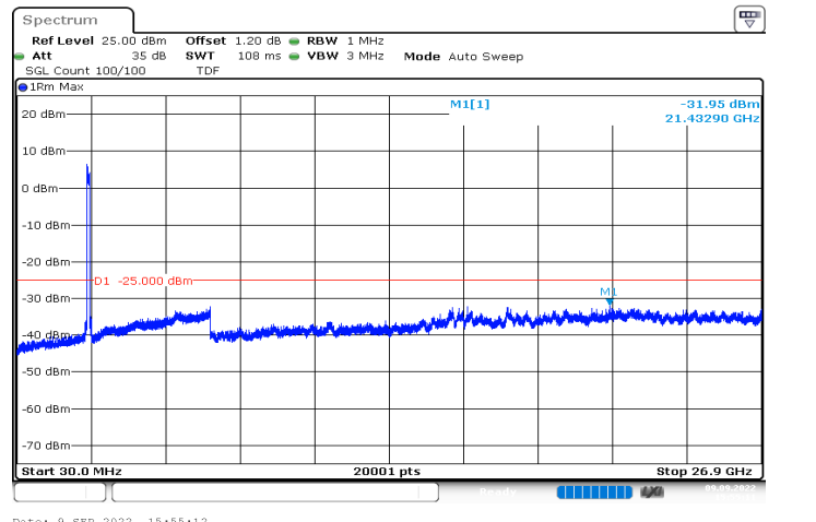
n41_100MHz_30kHz_2592.99MHz_DFT-s-OFDM_QPSK_RB270@0|30MHz_26.9GHz
