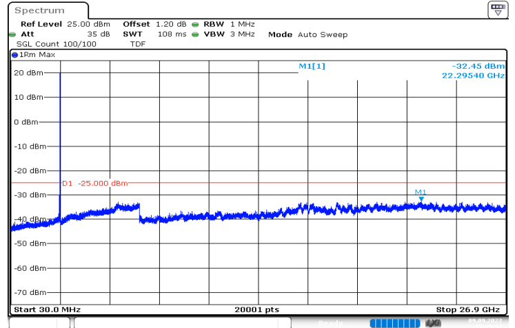
n41_50MHz_30kHz_2664.99MHz_DFT-s-OFDM QPSK_RB1@132|30MHz_26.9GHz
