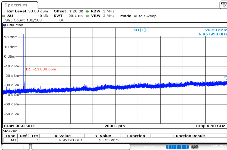
n71_5MHz_15kHz_665.5MHz_DFT-s-OFDM QPSK_RB1@0|30MHz_6.98GHz
