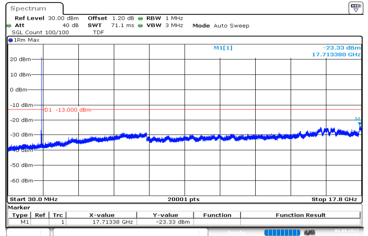
n66_40MHz_15kHz_1730MHz_DFT-s-OFDM QPSK_RB1@0|30MHz_17.8GHz
