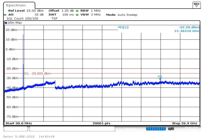
n41_10MHz_30kHz_2592.99MHz_DFT-s-OFDM QPSK_RB24@0|30MHz_26.9GHz
