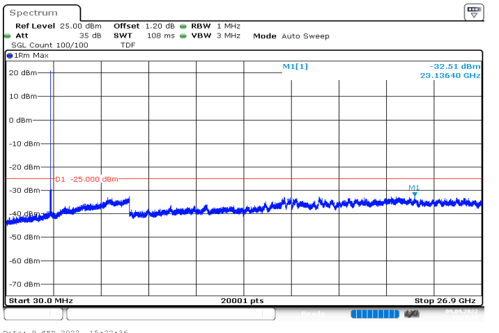
n41_60MHz_30kHz_2526MHz_DFT-s-OFDM QPSK_RB1@161|30MHz_26.9GHz
