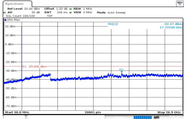
n41_20MHz_30kHz_2679.99MHz_DFT-s-OFDM QPSK_RB1@50|30MHz_26.9GHz
