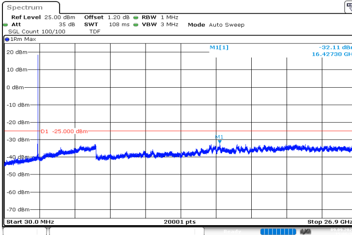
n41_40MHz_30kHz_2592.99MHz_DFT-s-OFDM QPSK_RB1@0|30MHz_26.9GHz
