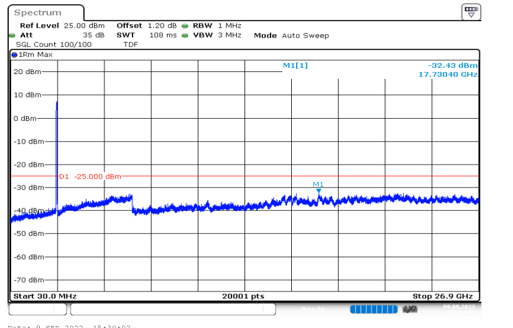
n41_60MHz_30kHz_2659.98MHz_DFT-s-OFDM QPSK_RB162@0|30MHz_26.9GHz
