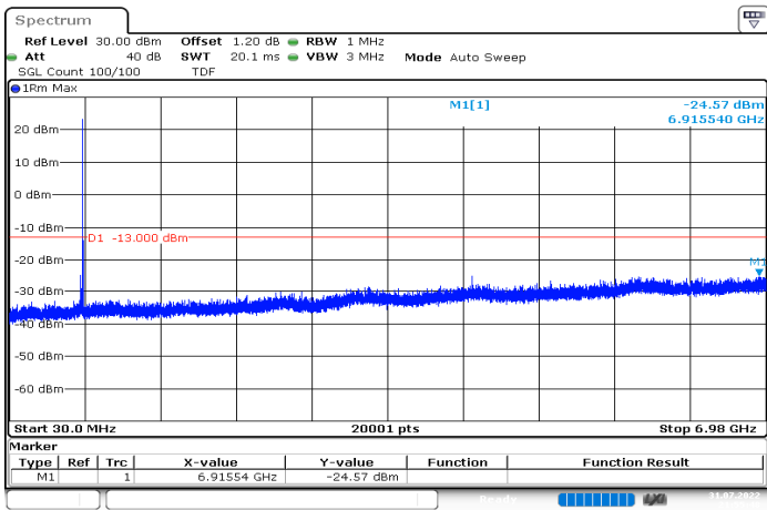
n71_20MHz_15kHz_688MHz_DFT-s-OFDM QPSK_RB1@105|30MHz_6.98GHz
