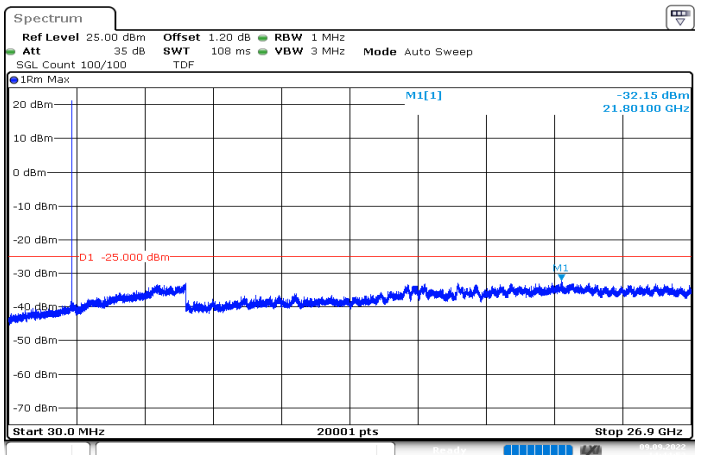
n41_15MHz_30kHz_2503.5MHz_DFT-s-OFDM QPSK_RB1@37|30MHz_26.9GHz
