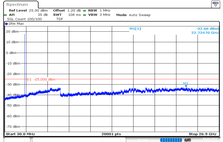
n41_20MHz_30kHz_2506.02MHz_DFT-s-OFDM QPSK_RB1@50|30MHz_26.9GHz
