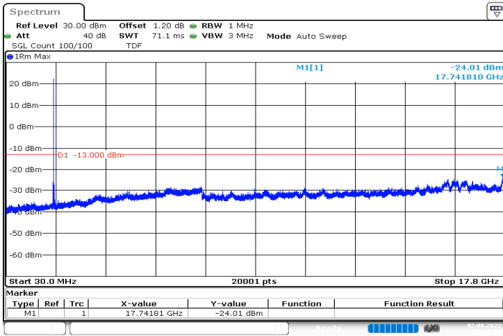
n66_5MHz_15kHz_1712.5MHz_DFT-s-OFDM QPSK_RB1@0|30MHz_17.8GHz
