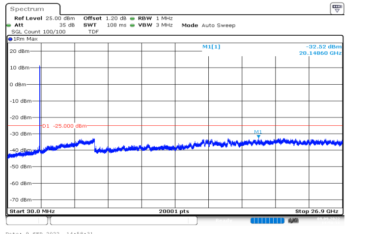
n41_20MHz_30kHz_2592.99MHz_DFT-s-OFDM QPSK_RB50@0|30MHz_26.9GHz
