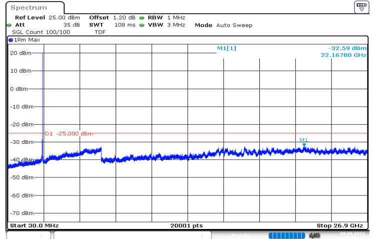
n41_60MHz_30kHz_2592.99MHz_DFT-s-OFDM QPSK_RB1@161|30MHz_26.9GHz
