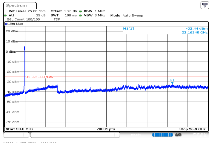
n41_90MHz_30kHz_2644.98MHz_DFT-s-OFDM QPSK_RB243@0|30MHz_26.9GHz
