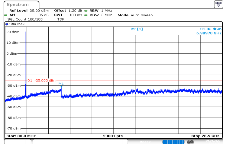
n41_80MHz_30kHz_2536.02MHz_DFT-s-OFDM QPSK_RB1@216|30MHz_26.9GHz
