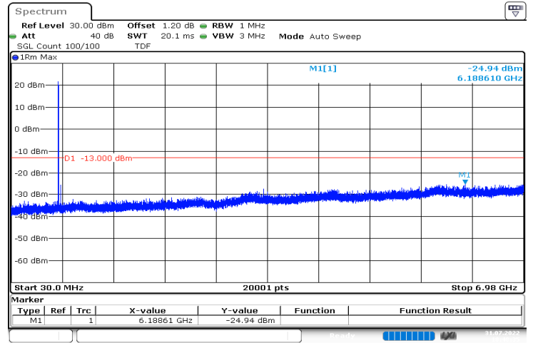
n71_5MHz_15kHz_665.5MHz_DFT-s-OFDM QPSK_RB1@24|30MHz_6.98GHz
