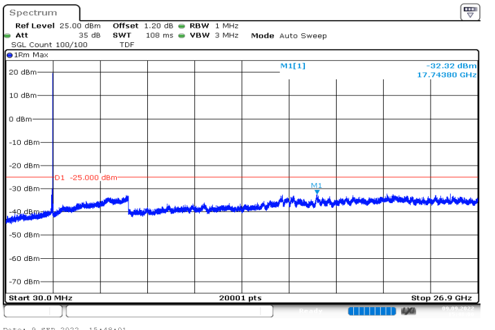
n41_90MHz_30kHz_2644.98MHz_DFT-s-OFDM QPSK_RB1@244|30MHz_26.9GHz
