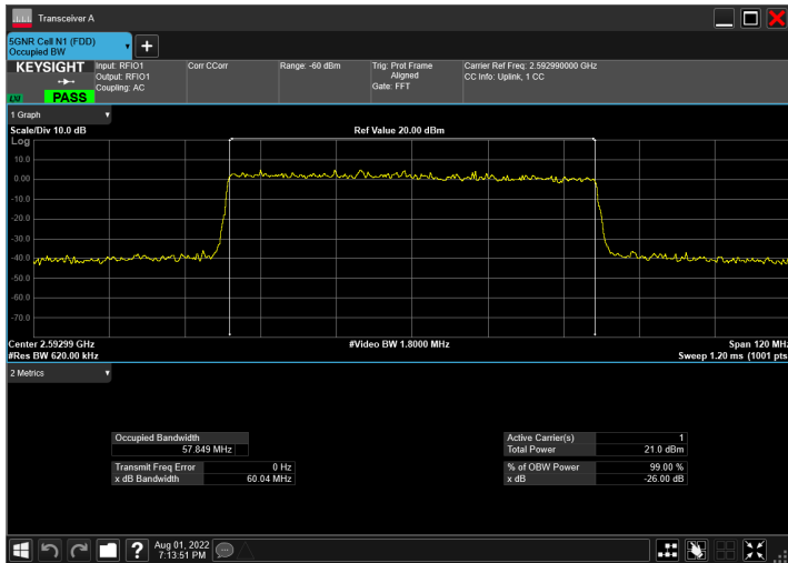
n41_60MHz_30kHz_2592.99MHz_DFT-s-OFDM QPSK_RB162@0
