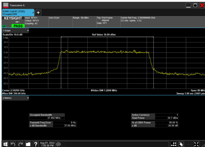
n41_40MHz_30kHz_2592.99MHz_DFT-s-OFDM QPSK_RB100@0
