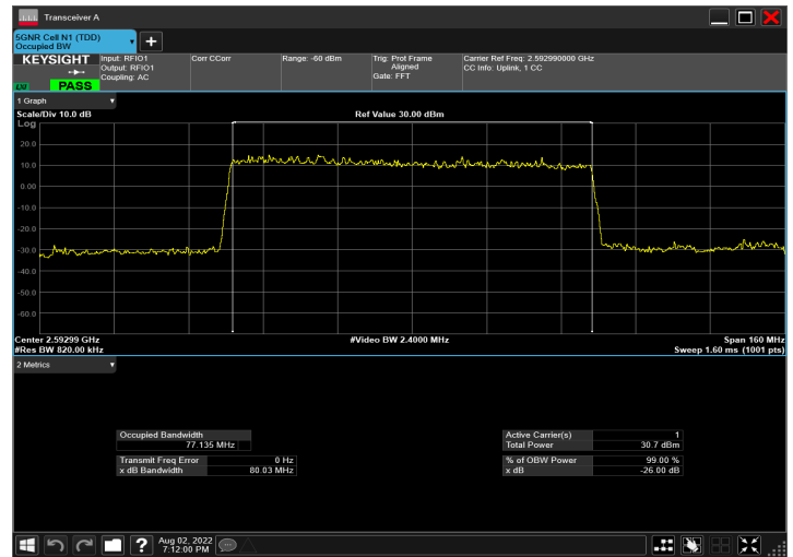
n41_80MHz_30kHz_2592.99MHz_DFT-s-OFDM PI/2 BPSK_RB216@0
