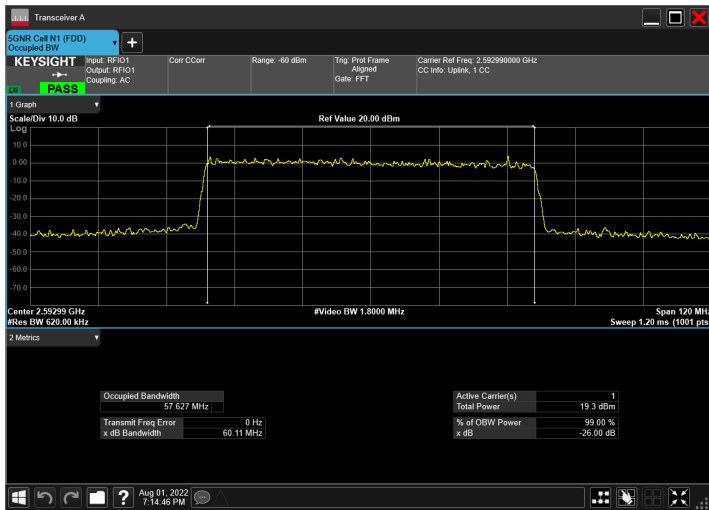
n41_60MHz_30kHz_2592.99MHz_CP-OFDM QPSK_RB162@0
