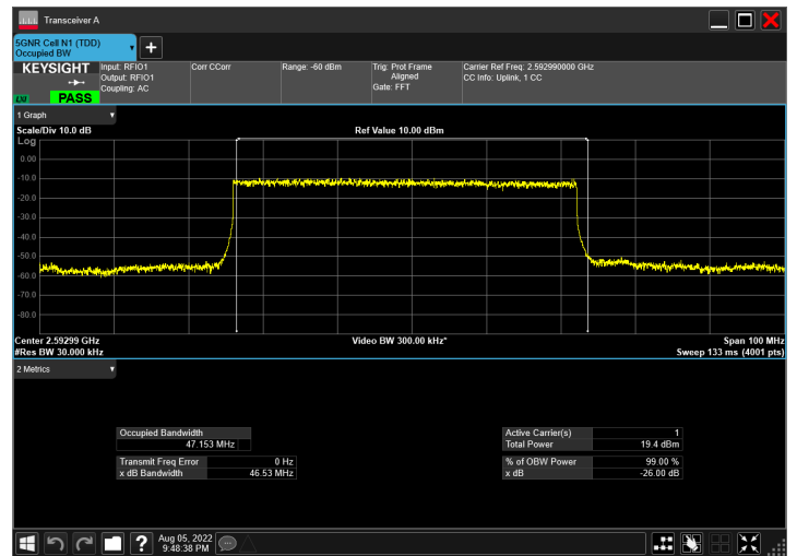
DC_66A_n41A_10MHz|50MHz_30kHz_1745MHz|2592.99MH z_QPSK|CP-OFDM QPSK_RB1@50|RB133@0
