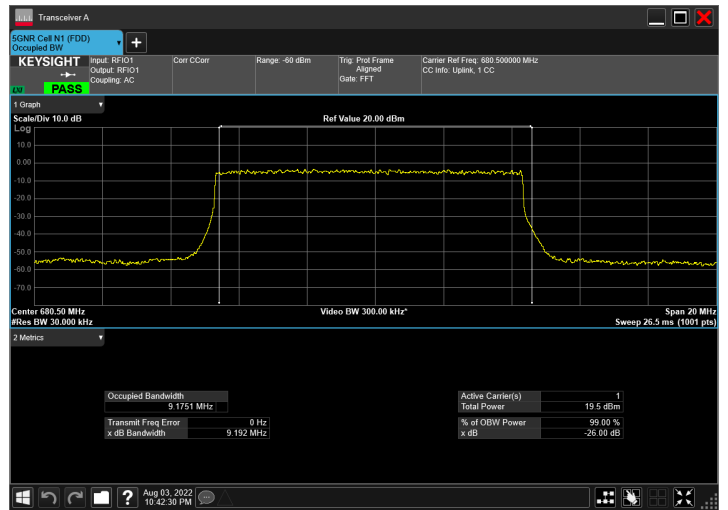
DC_66A_n71A_10MHz|10MHz_15kHz_1745MHz|680.5MHz_QPSK|DFT-s-OFDM PI/2 BPSK_RB1@50|RB50@0
