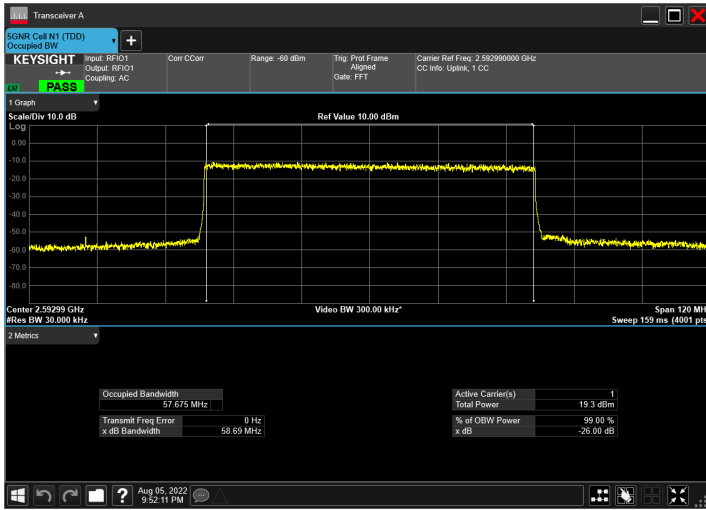
DC_66A_n41A_10MHz|60MHz_30kHz_1745MHz|2592.99MH z_QPSK|CP-OFDM QPSK_RB1@50|RB162@0
