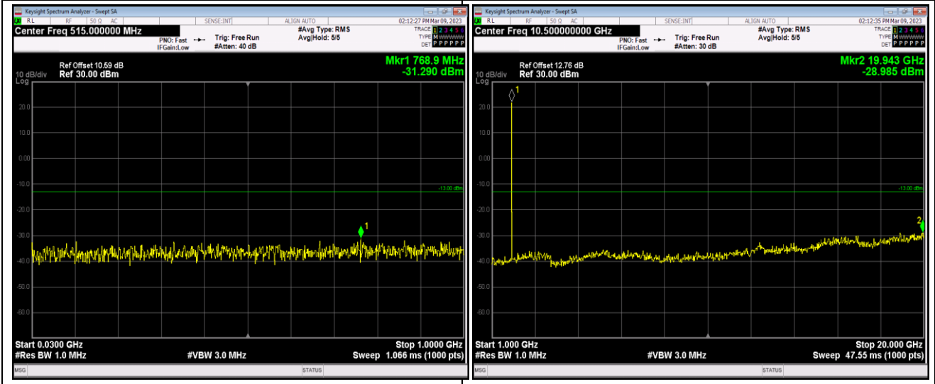
Band25-1.4MHz-64QAM-26365-1RB#0-Range1:30 ~1000MHz
