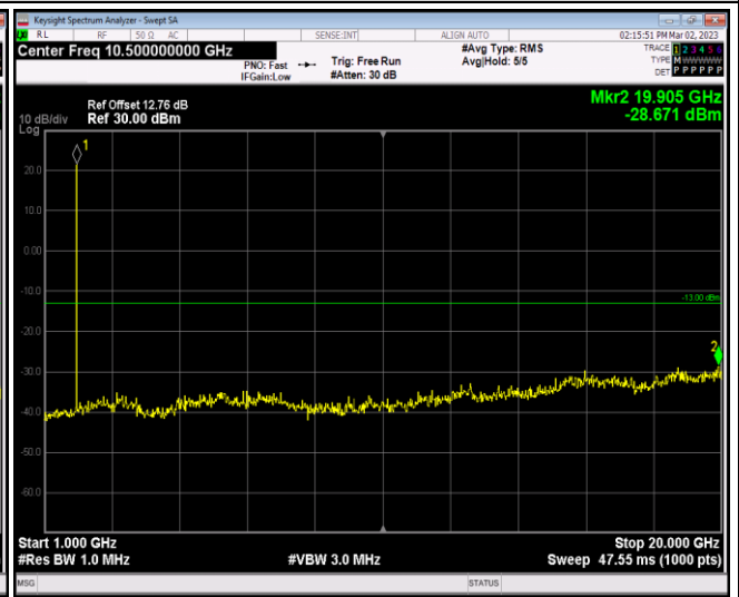
Band25-1.4MHz-QPSK-26683-1RB#0-Range2:1000~20000MHz
