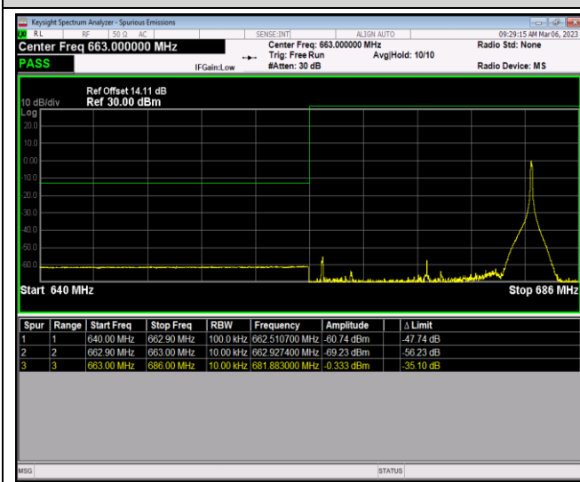
Band71-20MHz-16QAM-133372-1RB#0
