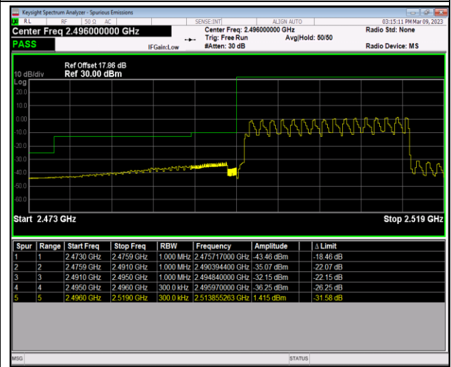
Band41-20MHz-64QAM-41490-1RB#99
