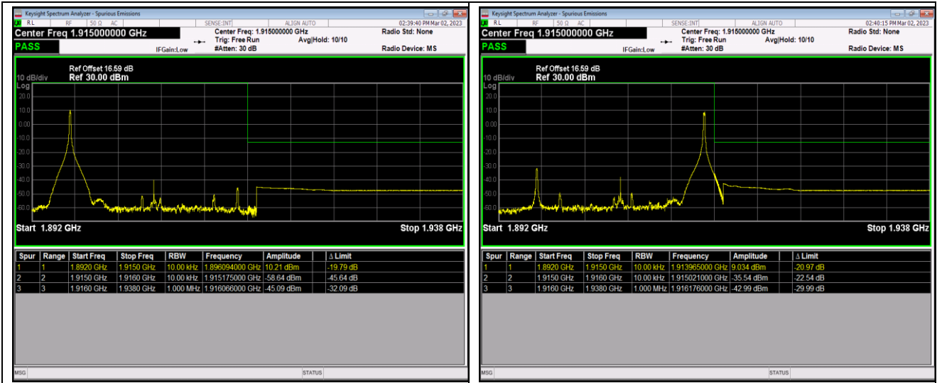
Band25-20MHz-QPSK-26590-100RB#0
