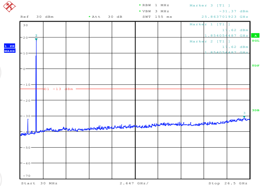
BW1.4MHz-1850.7MHz,QPSK-6RB_LOW@Pass
