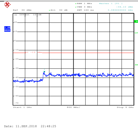
1GHz~9GHz
