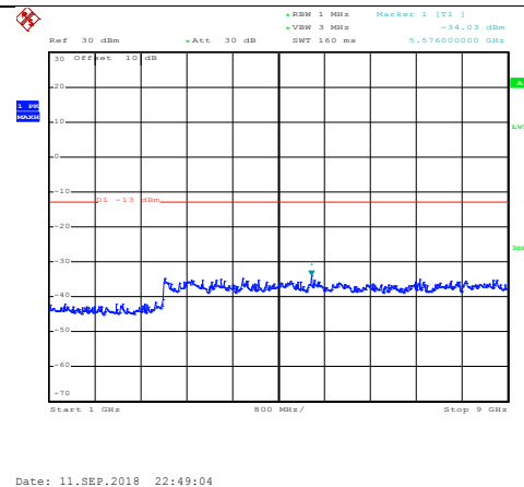
1GHz~9GHz
