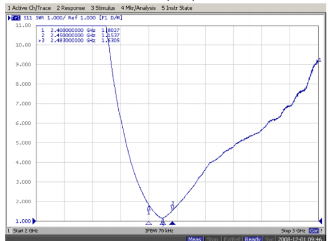
VSWR(S 11 )
