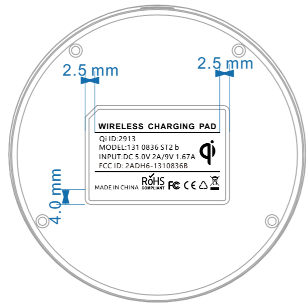
镭射雕刻位置图（正中心）
