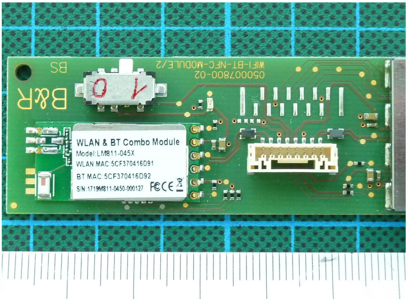
170923_pcb_04
