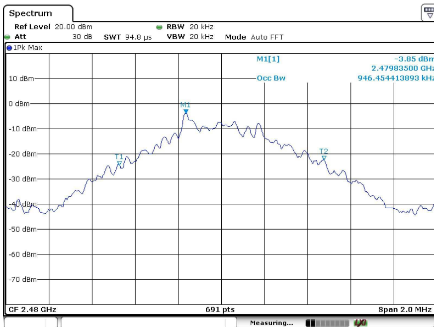
2480MHz, GFSK
