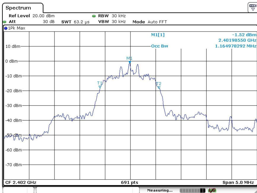
2402MHz, 8DPSK
