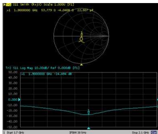
1900MHz Head
