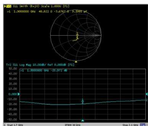
1900MHz Body
