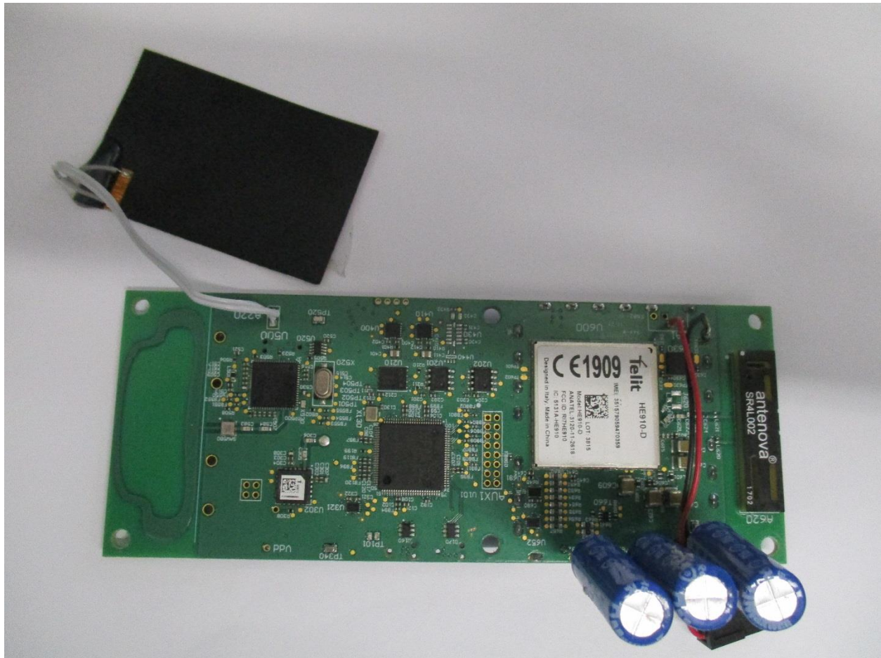
PCB Top
