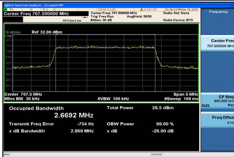
Band12-3MHz-16QAM-23095-15RB#0-2.6692
