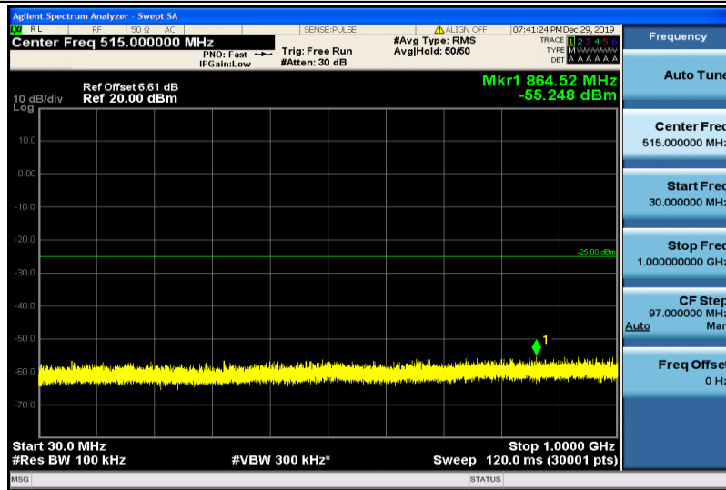
Band41-10MHz-QPSK-40290-1RB#0-30~1000MHz
