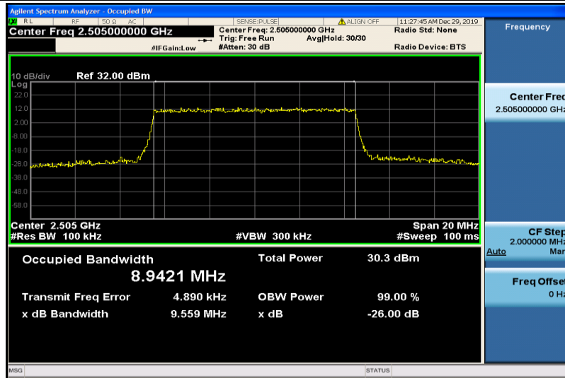
Band7-10MHz-QPSK-20800-50RB#0-8.9421
