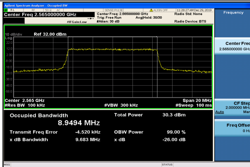
Band7-10MHz-QPSK-21400-50RB#0-8.9494
