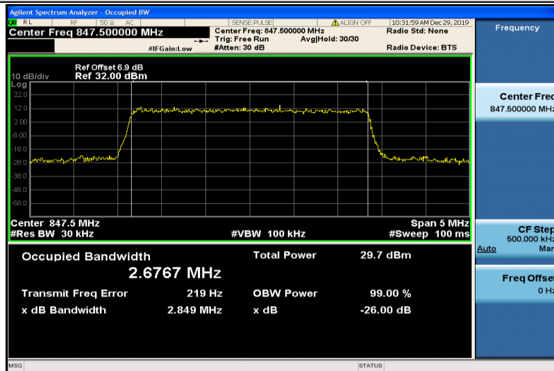
Band5-3MHz-QPSK-20635-15RB#0-2.6767
