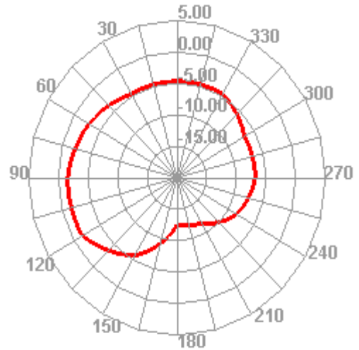
5150.000MHz H
