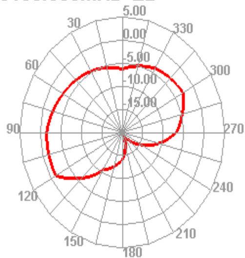
5150.000MHz E2
