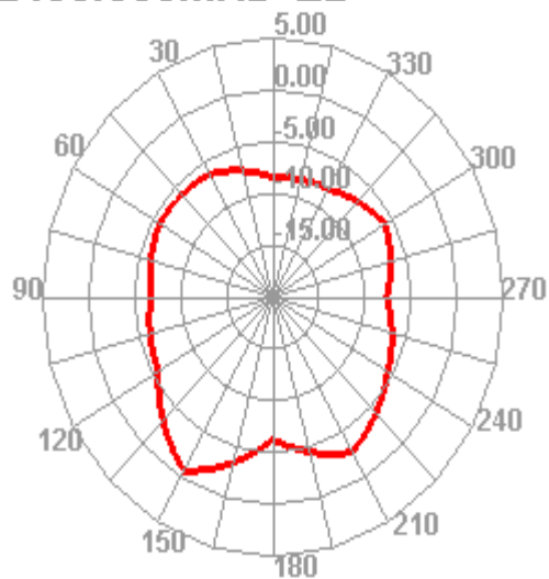
2400.000MHz E2
