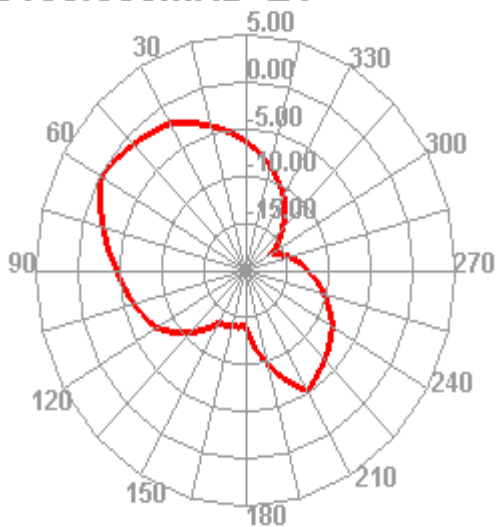
5150.000MHz E1
