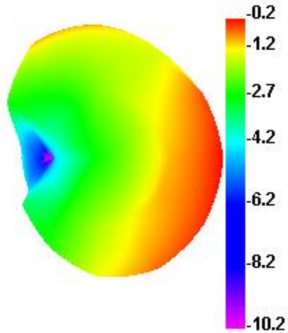
5150.000MHz
