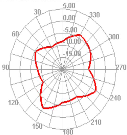
2400.000MHz E1
